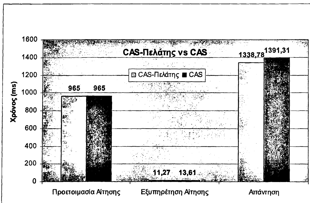
Σχήμα 4.3 Λήψη πιστοποιητικού σε τοπικό δίκτυο και χαμηλό φορτίο
