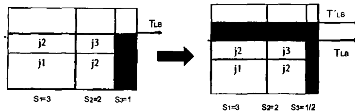
Σχήμα 4.7: "Ο Πιθανοτικός Μηχανισμός είναι Υλοποιήσιμος"
