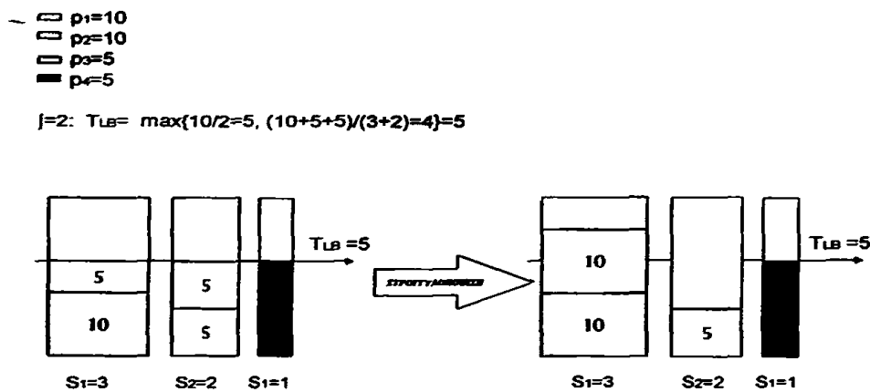
Σχήμα 4.5: "Παράδειγμα Μηχανισμού με Ακέραιες Αναθέσεις Διεργασιών"
