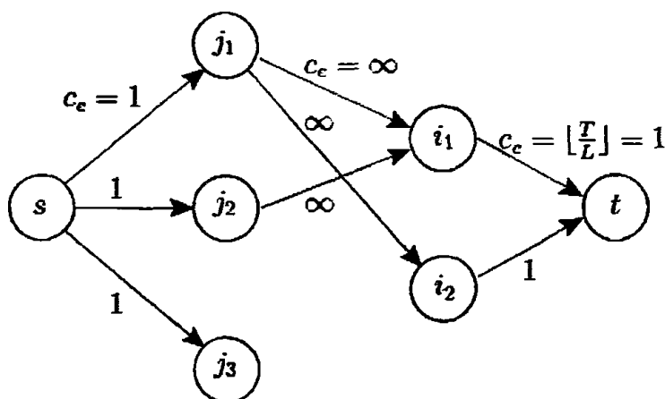
Σχήμα 5.5: Δίκτυο Ροής (p, T) , με 3 Διεργασίες, 2 Μηχανές και T=L
