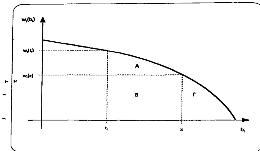
Σχήμα 4.2α: "Ο παίκτης i δεν κερδίζει ποτέ αν «μπλοφάρει»"
