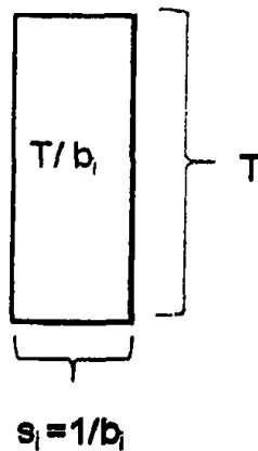
Σχήμα 4.4: Καλάθι Μεγέθους T/b_i
