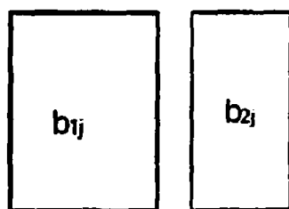
Σχήμα 6.1: "Ο Γενικός Μηχανισμός είναι Φιλαλήθης"
