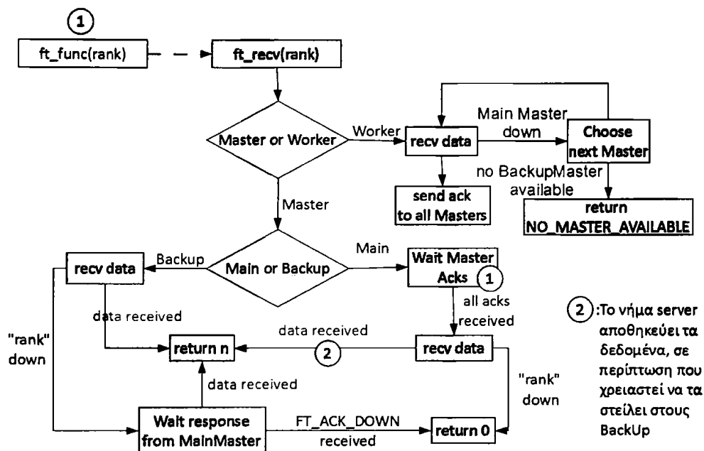
Εικόνα 4.8: Διάγραμμα Ροής ft_recv, με Πολλαπλούς Master
