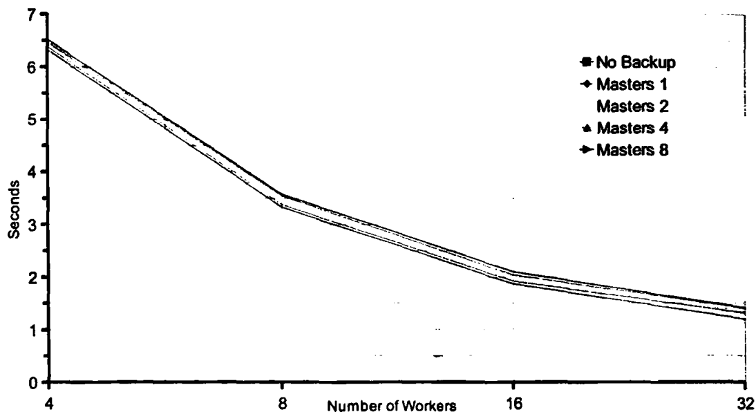
Εικόνα 5.8: Χρόνος Εκτέλεσης για 128 Βελτιστοποιήσεις
