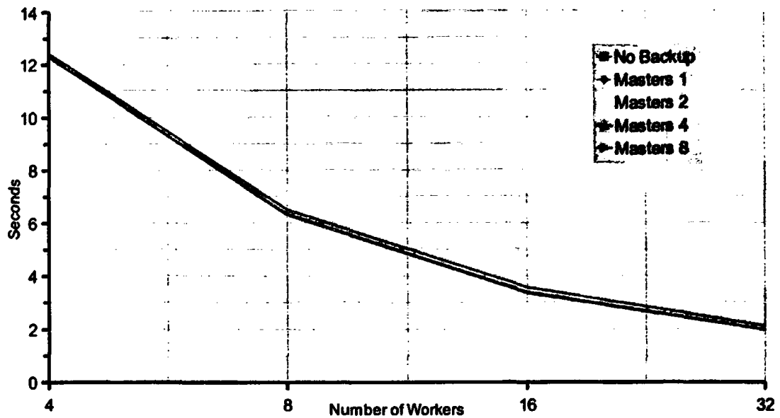
Εικόνα 5.9: Χρόνος Εκτέλεσης για 256 Βελτιστοποιήσεις
