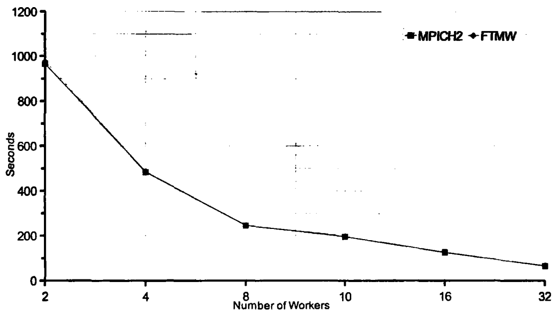
Εικόνα 5.4: Χρόνος Εκτέλεσης για 256 Βελτιστοποιήσεις (100ms)
