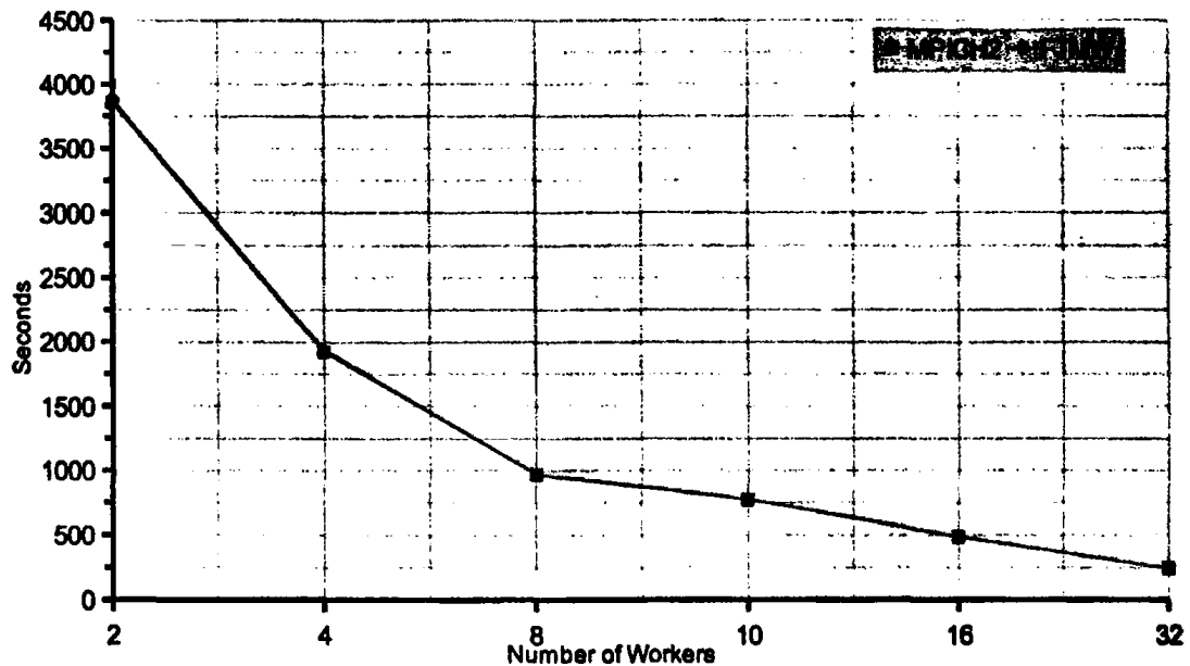
Εικόνα 5.5: Χρόνος Εκτέλεσης για 1024 Βελτιστοποιήσεις (100ms)
