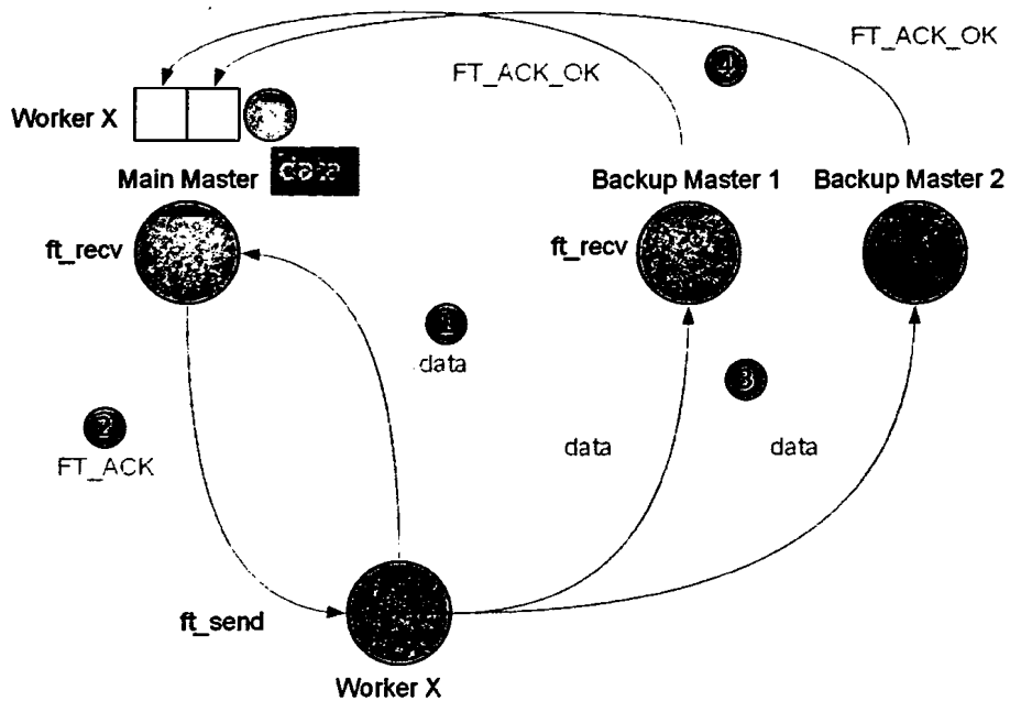
Εικόνα 4.11: Βήματα Διαδικασίας Παράλαβης Δεδομένων, με Πολλαπλούς Master
