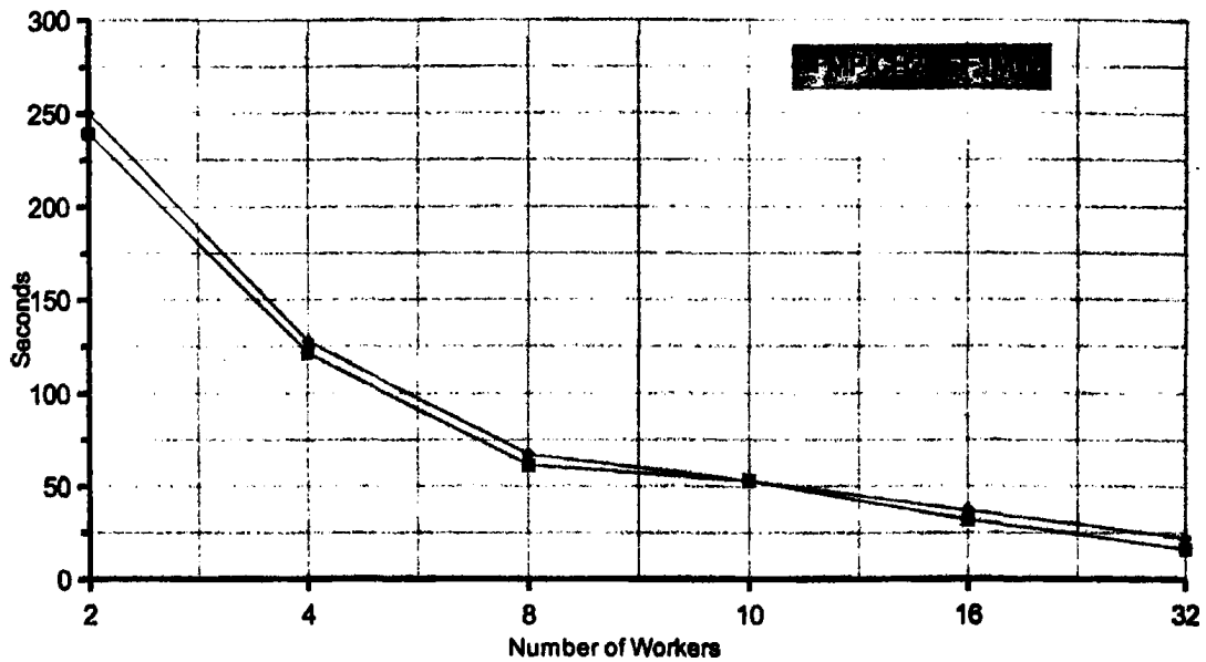
Εικόνα 5.3: Χρόνος Εκτέλεσης για 64 Βελτιστοποιήσεις (100ms)
