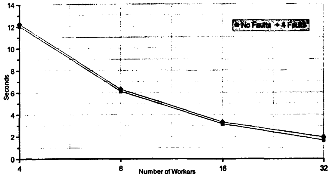
Εικόνα 5.7: Χρόνος Εκτέλεσης για 256 Βελτιστοποιήσεις
