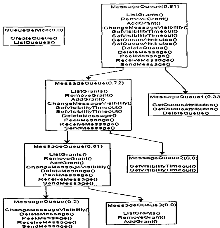
Σχήμα 4.7 Ομαδοποίηση της Διεπαφής Amazon MessageQueuePortType από τον Διαιρετικό Αλγόριθμο
