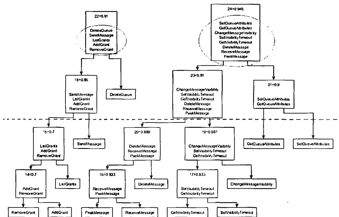
Σχήμα 4.4 Ομαδοποίηση της Διεπαφής Amazon MessageQueuePortType
