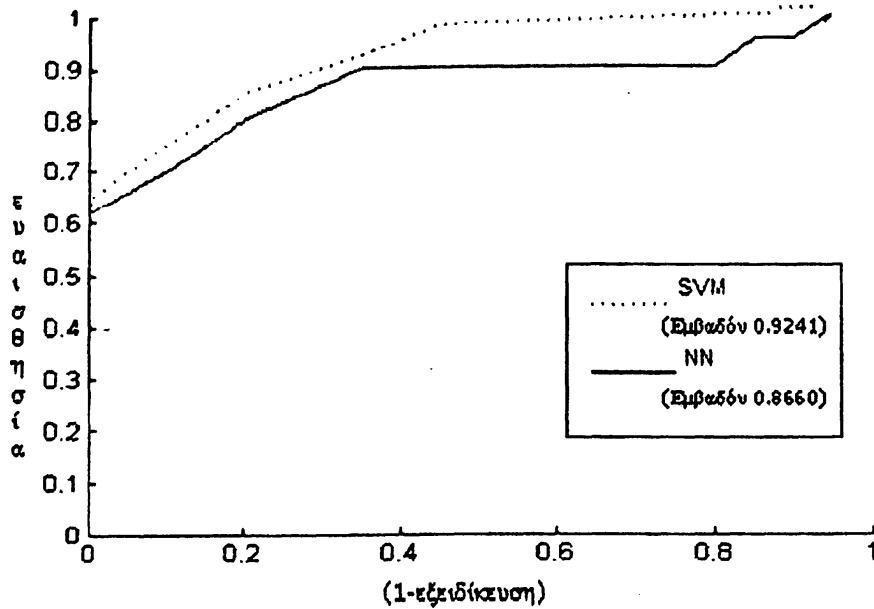
Σχήμα 5.1: Καμπύλες ROC για τους δύο ταξινομητές στην περίπτωση διαχωρισμού παθολογικής από κανονική βάδιση.
