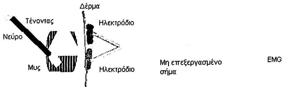
Σχήμα 1.11: Ηλεκτρόδιο για την μέτρηση EMG.
