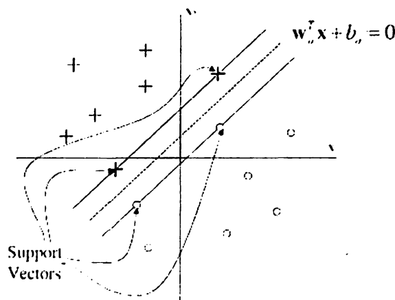
Σχήμα 3.2: Παράδειγμα εφαρμογής SVM και δημιουργία ενός επιπέδου που διαχωρίζει τα δεδομένα σε δύο κλάσεις. Με το σταυρό είναι τα δεδομένα που ανήκουν στην κλάση +1 και με τον κύκλο τα δεδομένα της κλάσης -1.
