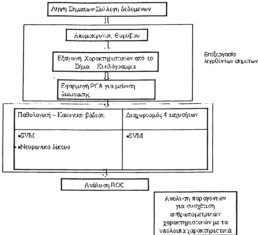
Σχήμα 5.1: Διάγραμμα μεθοδολογίας την οποία ακολουθήσαμε.
