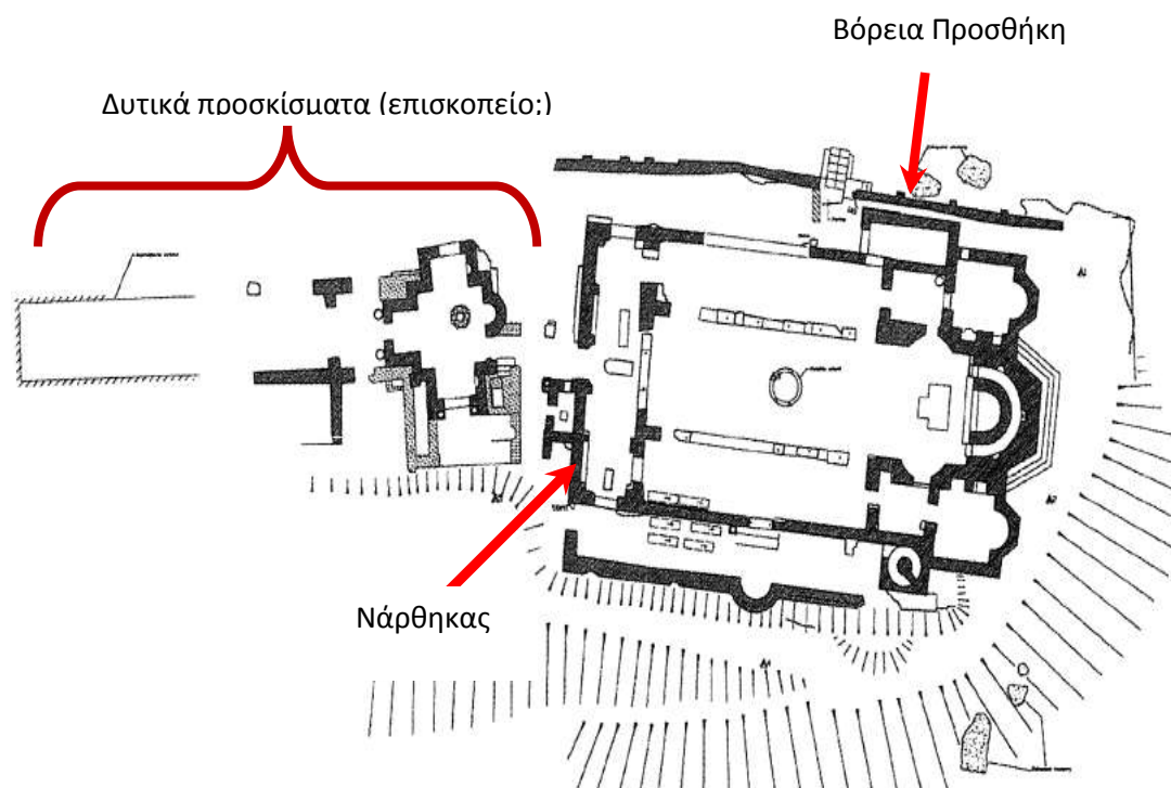
Εικόνα 10. Σχεδιάγραμμα της βασιλικής στην ακρόπολη της Σπάρτης.
