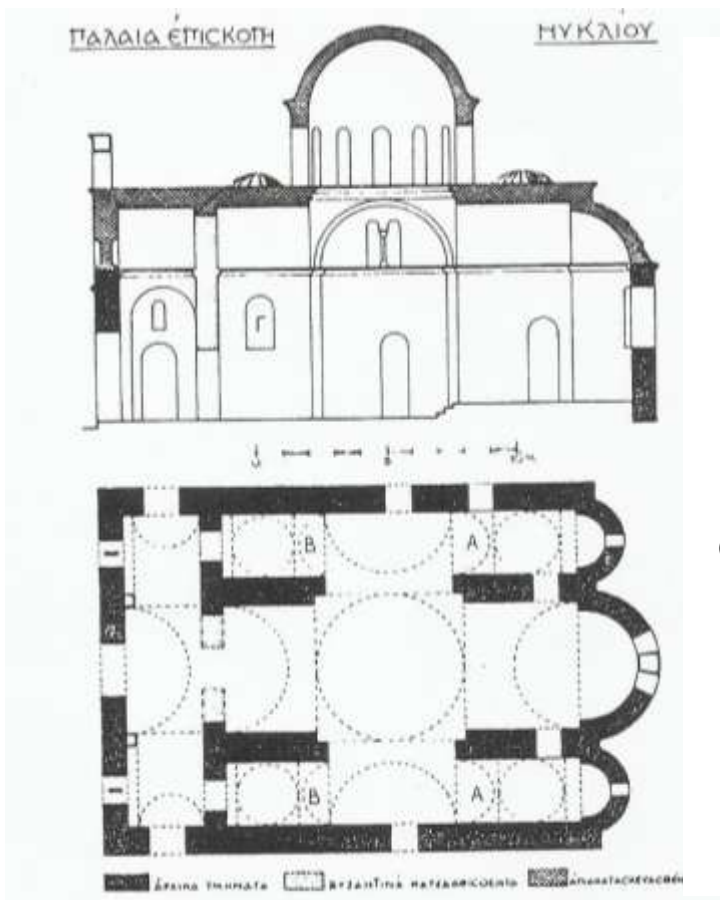
Εικόνα 14. Επισκοπή Τεγέας. Τομή και κάτοψη του ναού, σύμφωνα με τον Α. Ορλάνδο.
