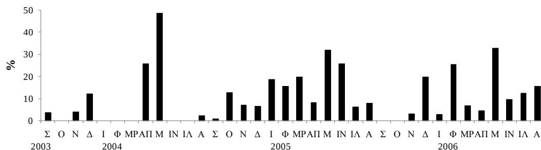
Εικόνα 3.45: Μέση ποσοστιαία συμμετοχή των ωοφόρων απόμων στον πληθυσμό του K. longirostris στο στρώμα των 0-20 m.
