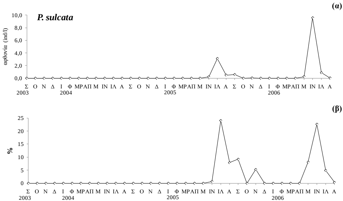
Εικόνα 3.61: (α) Εποχική διακύμανση της μέσης αφθονίας του είδους P. sulcata και (β) ποσοστιαία συμμετοχή του στο σύνολο των τροχόζωων στο στρώμα των 0-20 m.
