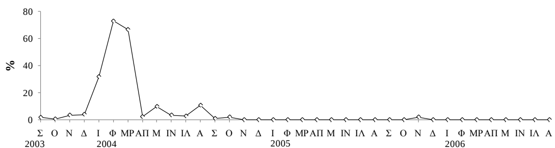
Εικόνα 3.74: (α) Εποχική διακύμανση της μέσης αφθονίας του είδους B. calyciflorus και (β) ποσοστιαία συμμετοχή του στο σύνολο των τροχοζώων στο στρώμα των 0-20 m.
