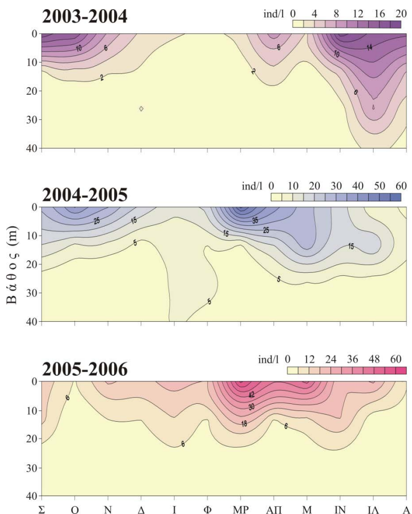
Εικόνα 3.8: Κατακόρυφη κατανομή της αφθονίας (ind/l) του E. drieschi στο σταθμό Α κατά τις τρεις δειγματοληπτικές περιόδους.
