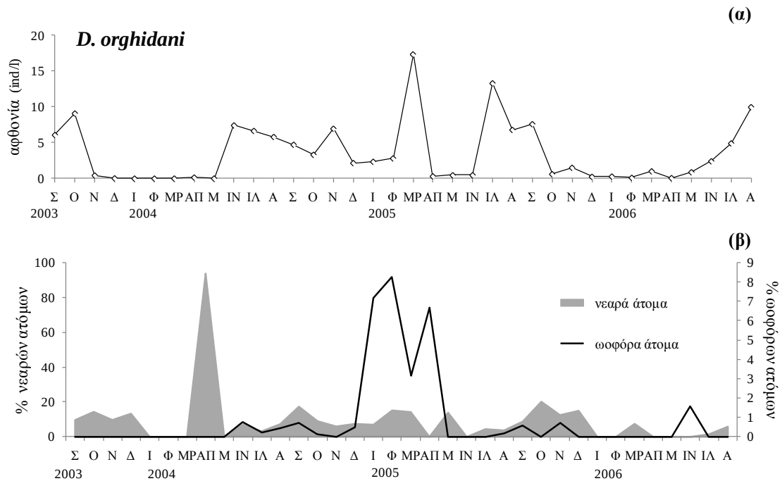
Εικόνα 4.31: (α) Εποχική διακύμανση της μέσης συνολικής αφθονίας του είδους D. orghidani και (β) μέση ποσοστιαία συμμετοχή των ωοφόρων και των νεαρών ατόμων του είδους στη συνολική του αφθονία του πληθυσμού στο στρώμα των 0-20 m.
