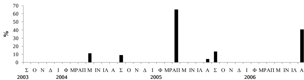
Εικόνα 3.68: Μέση ποσοστιαία συμμετοχή των ωοφόρων ατόμων στον πληθυσμό του είδους priodonta στο στρώμα των 0-20 m.
