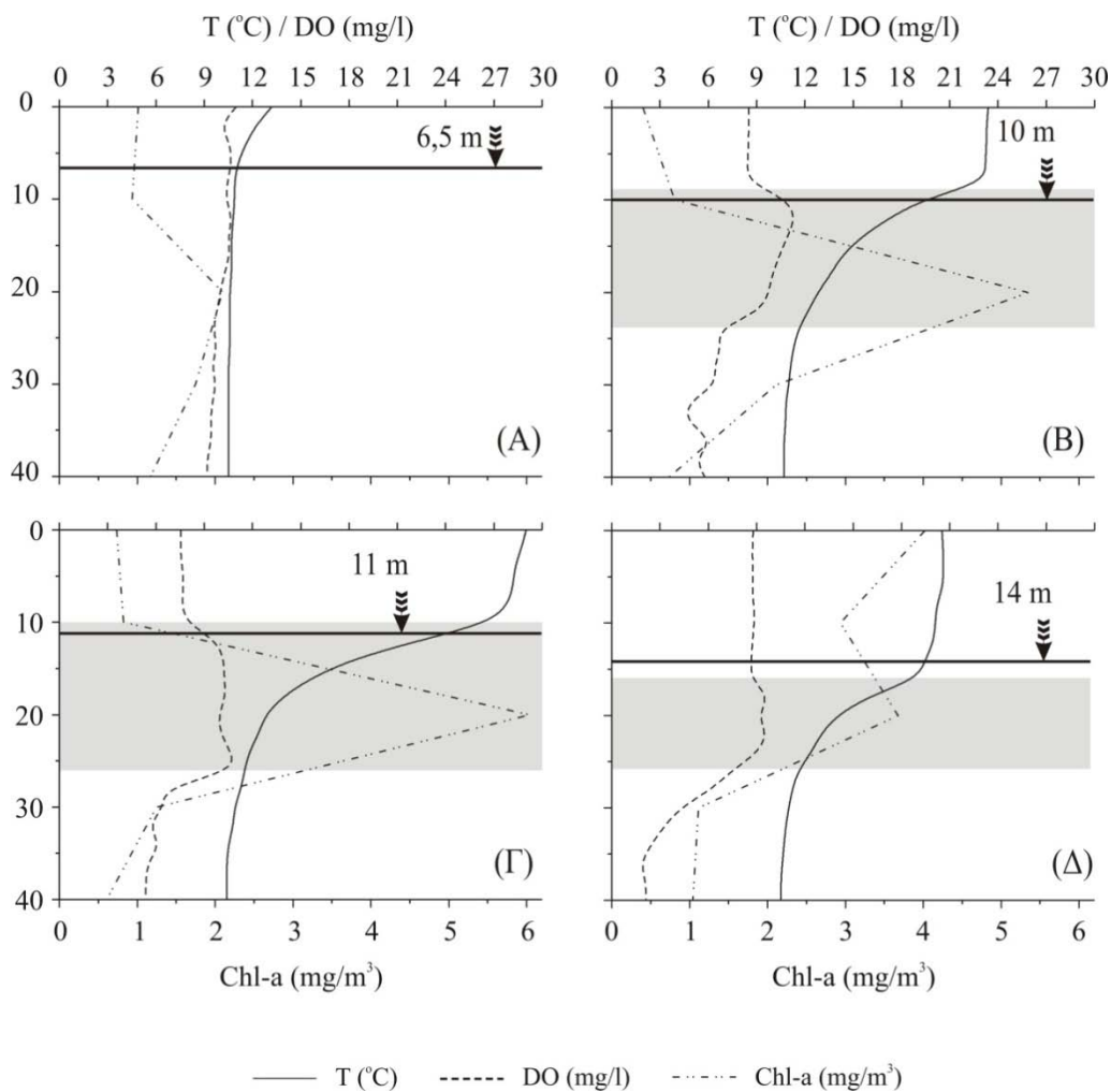
Εικόνα 4.1: Εποχική διακύμανση της κατακόρυφης κατανομής της θερμοκρασίας (T, °C), του διαλυμένου οξυγόνου (DO, mg/l) και της συγκέντρωσης χλωροφύλλης-α (chl-a, mg/m 3 ) στον σταθμό δειγματοληψίας, (Α) το χειμώνα, (Β) την άνοιξη, (Γ) το καλοκαίρι και (Δ) το φθινόπωρο. Με τη σκιασμένη περιοχή δηλώνεται το θερμοκλινές, ενώ το κατακόρυφο βέλος δείχνει την διαφάνεια του νερού.
