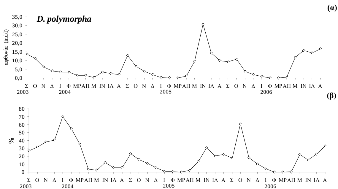
Εικόνα 3.85: (α) Εποχική διακύμανση της μέσης αφθονίας του είδους D. polymorpha και (β) ποσοστιαία συμμετοχή του είδους στο σύνολο των τροχοζώων στο στρώμα των 0-20 m.
