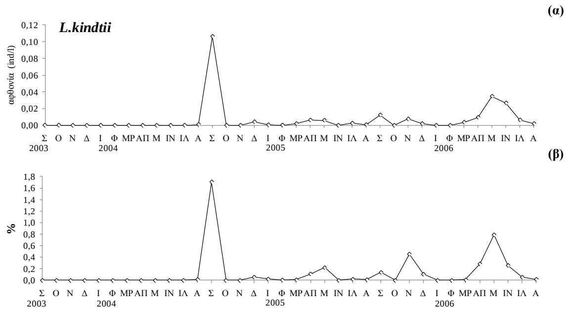
Εικόνα 3.36: (α) Εποχική διακύμανση της μέσης αφθονίας του είδους L. kindtii και (β) ποσοστιαία συμμετοχή του είδους στο σύνολο των τροχοζώων στο στρώμα των 0-20 m.
