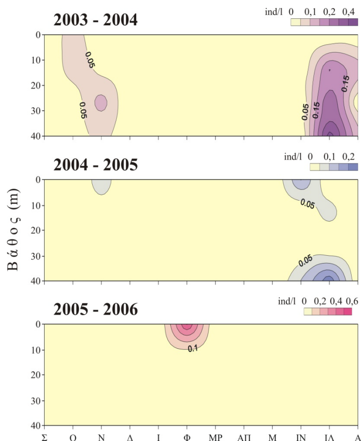
Εικόνα 3.82: Κατακόρυφη κατανομή της αφθονίας (ind/l) των τροχοζών της τάξης Bdelloidea στο σταθμό Α κατά τις τρεις δειγματοληπτικές περιόδους.
