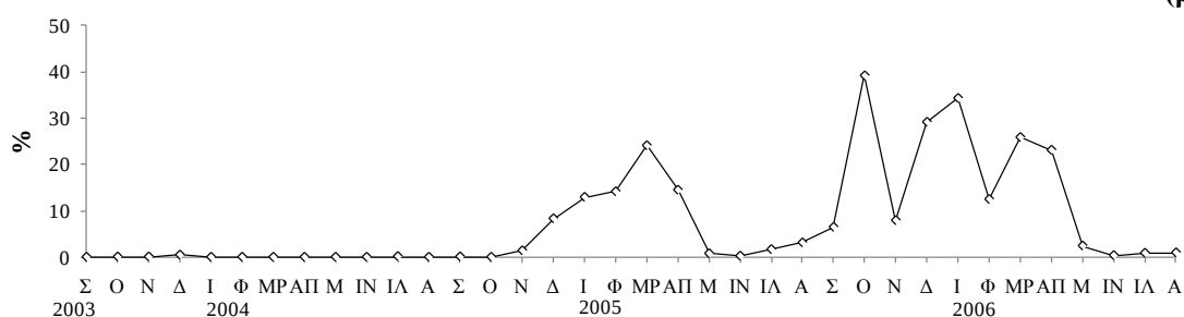
Εικόνα 3.52: (α) Εποχική διακύμανση της μέσης αφθονίας του είδους T. similis και (β) ποσοστιαία συμμετοχή του στο σύνολο των τροχοζώων στο στρώμα των 0-20 m.
