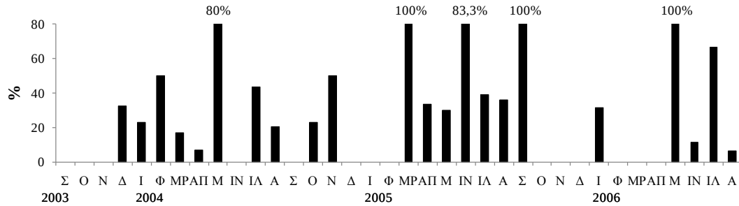
Εικόνα 3.72: Μέση ποσοστιαία συμμετοχή των ωοφόρων ατόμων στο σύνολο του γένους Colotheca sp. στο στρώμα των 0-20 m.
