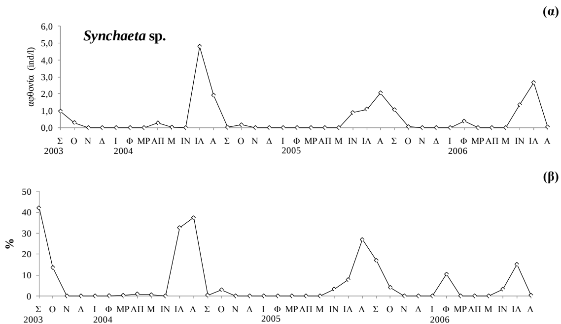
Εικόνα 3.54: (α) Εποχική διακύμανση της μέσης αφθονίας του γένους Synchaeta και (β) ποσοστιαία συμμετοχή του στο σύνολο των τροχοζώων στο στρώμα των 0-20 m.
