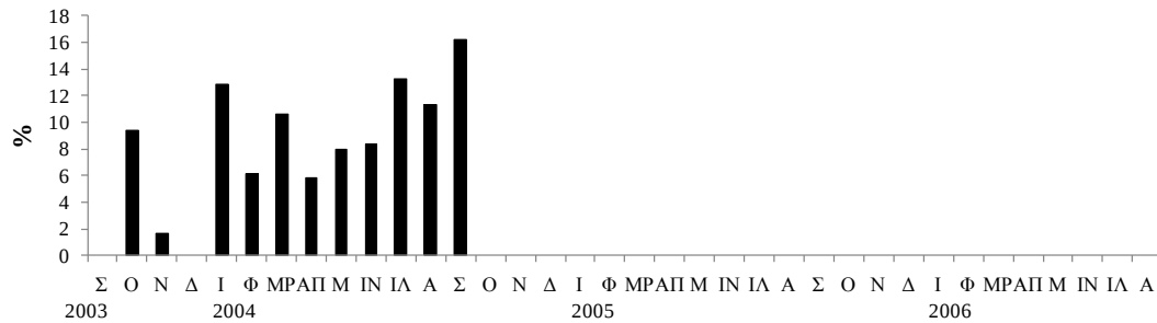
Εικόνα 3.75: Μέση ποσοστιαία συμμετοχή των ωοφόρων ατόμων στον πληθυσμό του είδους calyciflorus στο στρώμα των 0-20 m.
