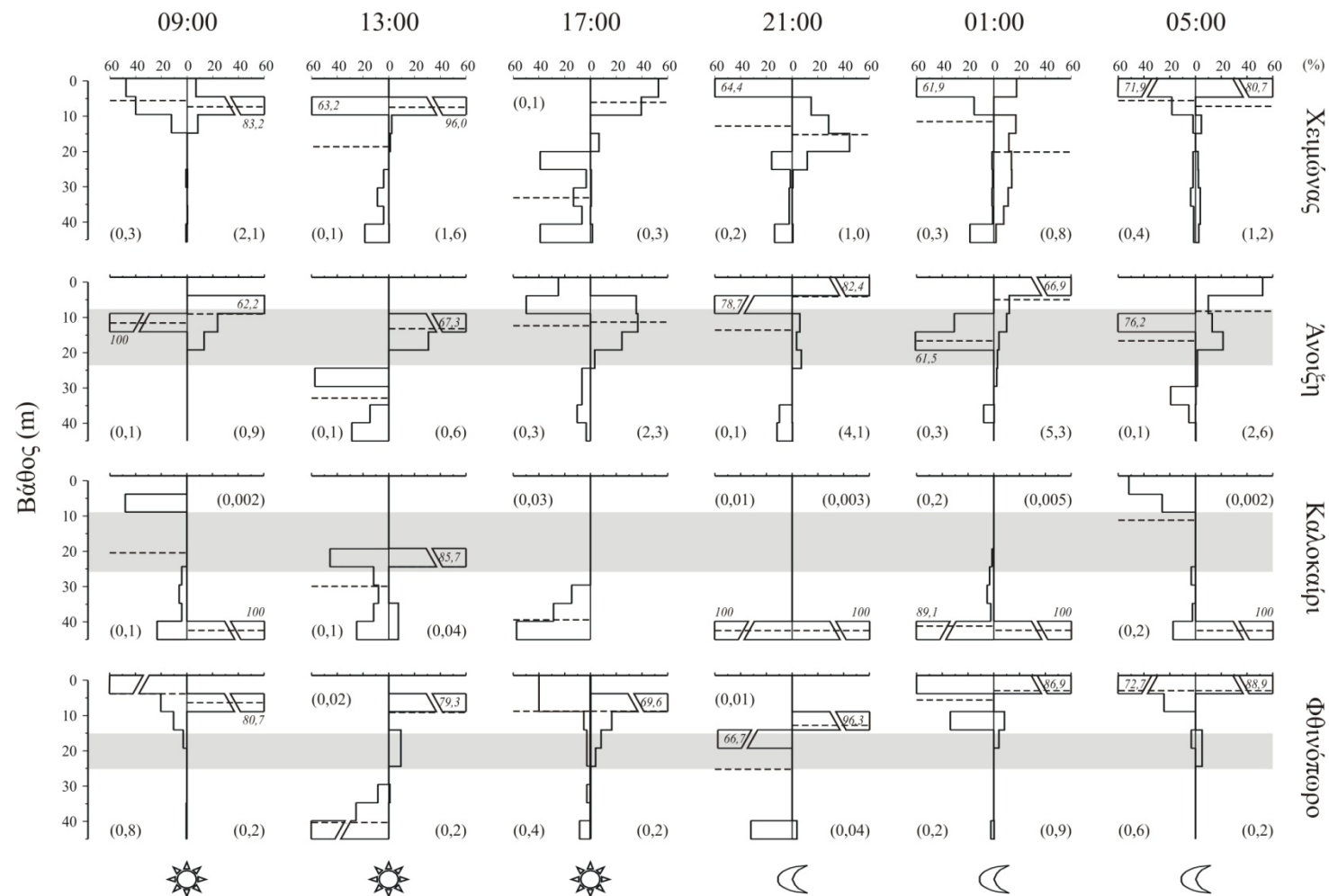
Εικόνα 4.15: Εποχική διακύμανση της ημερονύκτιας κατακόρυφης κατανομής των κωπηποδιών (αριστερά) και ενήλικων ατόμων (δεξιά) των κυκλοποειδών κωπηπόδων. Με τη σκιασμένη περιοχή δηλώνεται το θερμοκλινές ενώ με τη διακεκομμένη γραμμή το μέσο βάθος της κατακόρυφης κατανομής. Στην παρένθεση δίνεται η συνολική αφθονία (ind/l) των οργανισμών στην υδάτινη στήλη.
