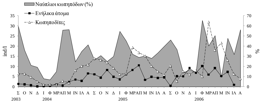
Εικόνα 3.20: Τριετής εποχική διακύμανση της μέσης αφθονίας του συνόλου των ενήλικων κωπηπόδων και των κωπηποδιτών και ποσοστιαία συμμετοχή των ναύπλιων στο σύνολο των κωπηπόδων στο στρώμα των 0-20 m.
