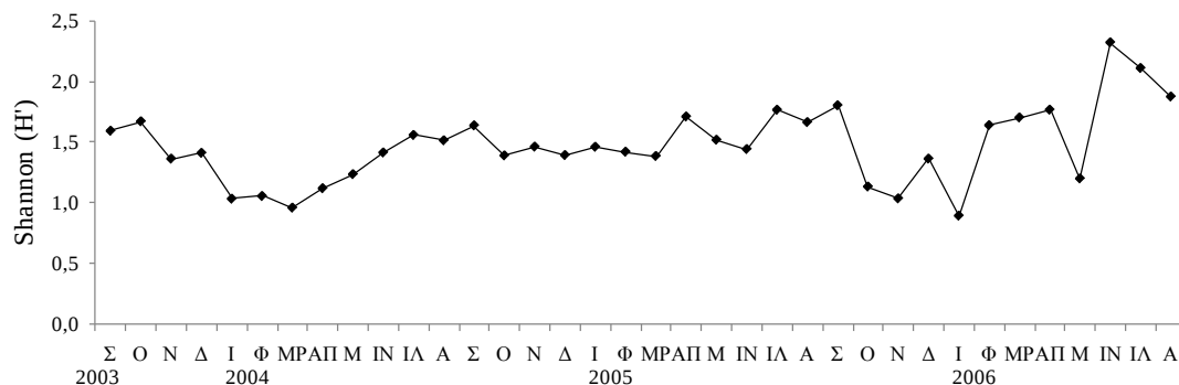
Εικόνα 3.86: Εποχικές μεταβολές του δείκτη ποικιλότητας Shannon.
