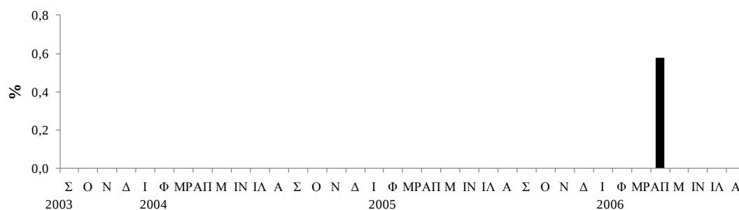
Εικόνα 3.48: Μέση ποσοστιαία συμμετοχή των ωοφόρων από μων στον πληθυσμό του C. unicornis στο στρώμα των 0-20 m.
