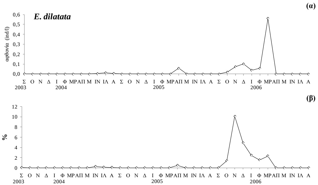
Εικόνα 3.79: (α) Εποχική διακύμανση της μέσης αφθονίας του είδους E. dilatata και (β) ποσοστιαία συμμετοχή του είδους στο σύνολο των τροχοζώων στο στρώμα των 0-20 m.
