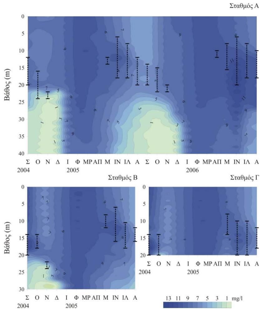
Εικόνα 2.4: Μηνιαία διακύμανση της κατακόρυφης κατανομής της συγκέντρωσης του διαλυμένου οξυγόνου στους 3 σταθμούς, κατά τις αντίστοιχες χρονικές περιόδους. Με τη διακεκομμένη κατακόρυφη γραμμή δηλώνονται τα όρια του θερμοκλινούς.
