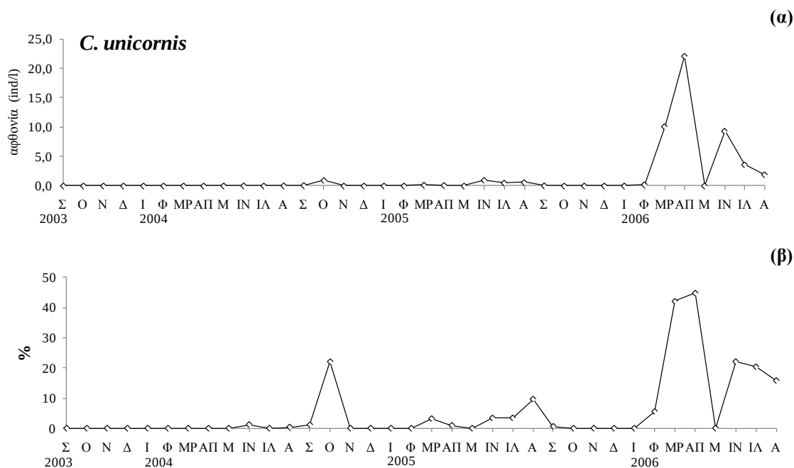
Εικόνα 3.47: (α) Εποχική διακύμανση της μέσης αφθονίας του είδους C. unicornis και (β) ποσοστιαία συμμετοχή του στο σύνολο των τροχοζώων στο στρώμα των 0-20 m.
