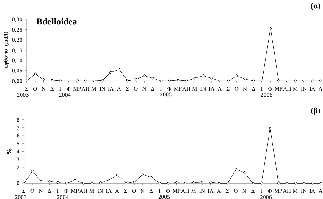
Εικόνα 3.81: (α) Εποχική διακύμανση της μέσης αφθονίας των τροχοζώνων της τάξης Bdelloidea και (β) ποσοστιαία συμμετοχή τους στο σύνολο των τροχοζώνων στο στρώμα των 0-20 m.
