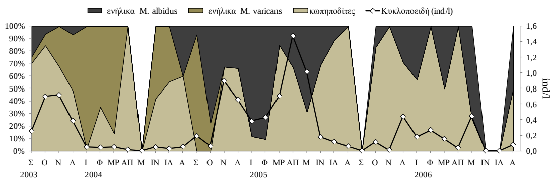
Εικόνα 3.15: Εποχική διακύμανση της μέσης αφθονίας των κυκλοποειδών κωπηπόδων και ποσοστιαία συμμετοχή των επιμέρους αναπτυξιακών σταδίων στο στρώμα των 0-20 m.
