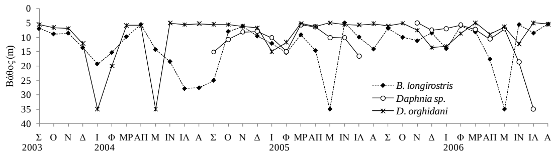
Εικόνα 3.37: Εποχική διακύμανση του μέσου βάθους κατακόρυφης κατανομής των κυριότερων ειδών κλαδόκερων στο σταθμό Α την περίοδο 2003-2006.
