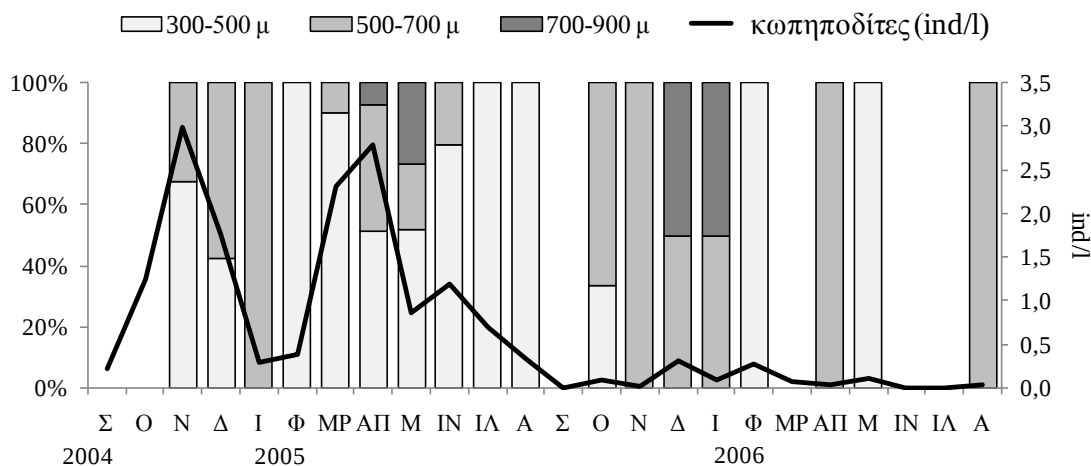
Εικόνα 3.18: Μείση ποσοστιαία συμμετοχή των κλάσεων μεγέθους των κωπηποδιτών καλανοειδών κωπηπόδων στην αφθονία τους στο στρώμα των 0-20 m και εποχική διακύμανσή της.
