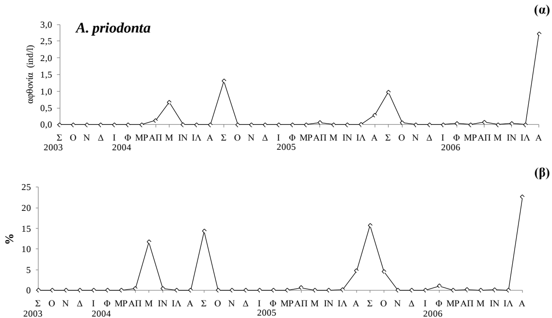
Εικόνα 3.69: (α) Εποχική διακύμανση της μέσης αφθονίας του είδους A. priodonta και (β) ποσοστιαία συμμετοχή του είδους στο σύνολο των τροχοζώων στο στρώμα των 0-20 m.
