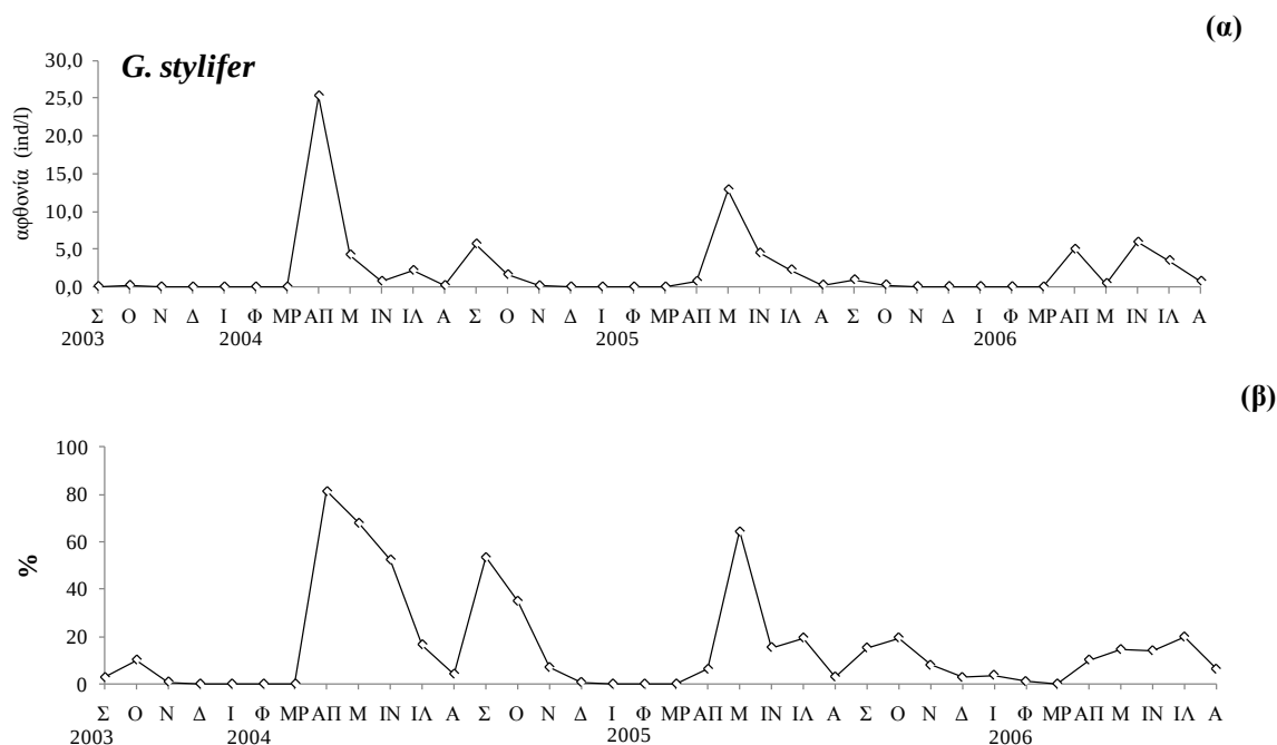
Εικόνα 3.42: (α) Εποχική διακύμανση της μέσης αφθονίας του είδους G. styliifer και (β) ποσοστιαία συμμετοχή του στο σύνολο των τροχοζώων στο στρώμα των 0-20 m.
