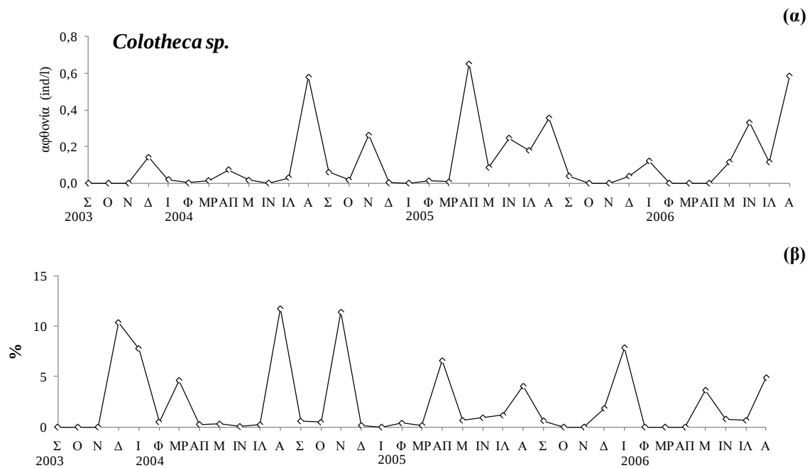
Εικόνα 3.71: (α) Εποχική διακύμανση της μέσης αφθονίας του γένους Colotheca sp. και (β) ποσοστιαία συμμετοχή του γένους στο σύνολο των τροχοζώων στο στρώμα των 0-20 m.
