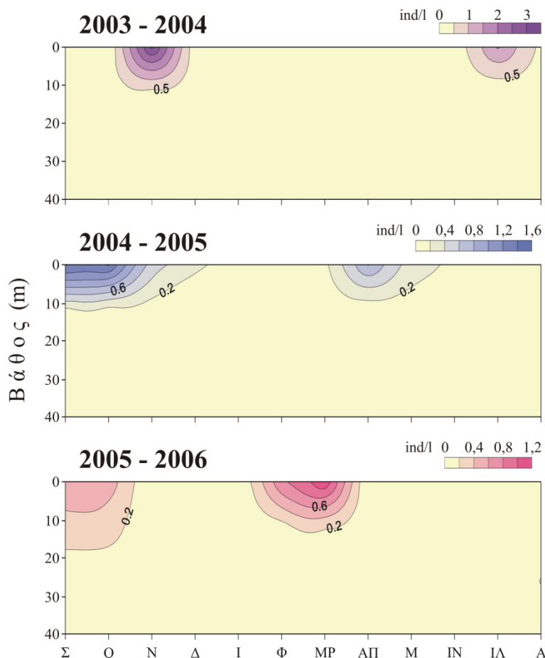
Εικόνα 3.65: Κατακόρυφη κατανομή της αφθονίας (ind/l) του γένους Polyarthra στο σταθμό Α κατά τις τρεις δειγματοληπτικές περιόδους.
