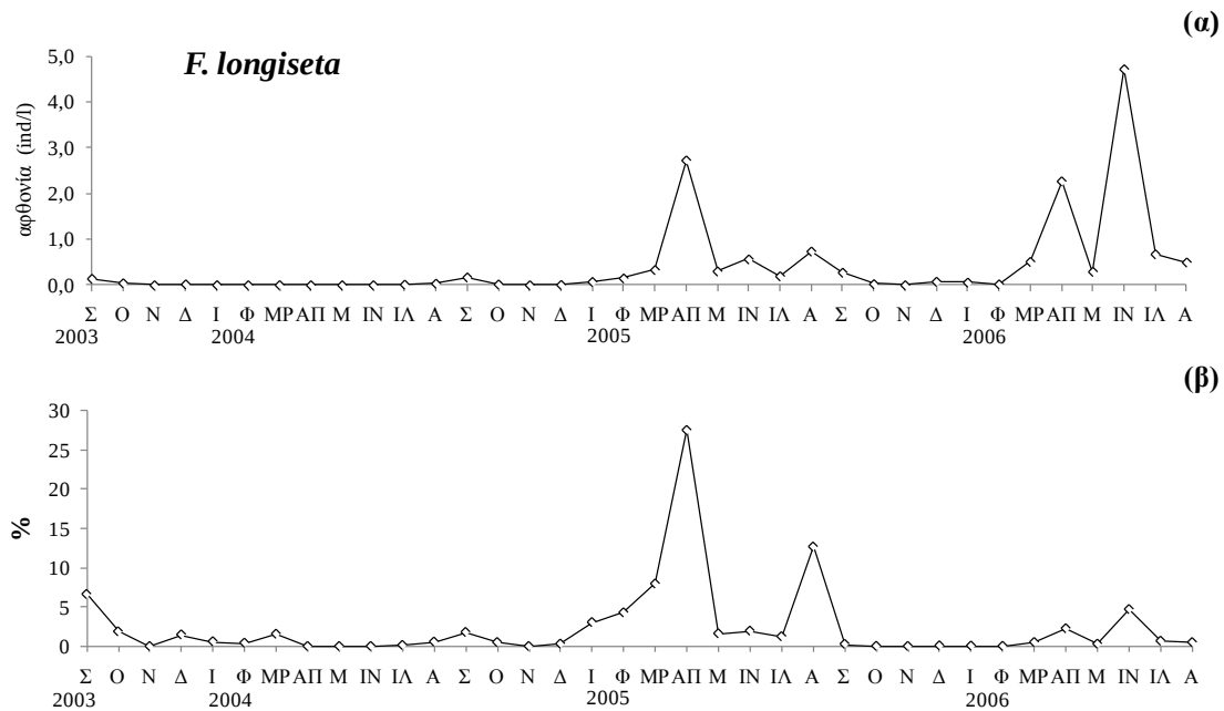
Εικόνα 3.63: (α) Εποχική διακύμανση της μέσης αφθονίας του είδους F. longiseta και (β) ποσοστιαία συμμετοχή του στο σύνολο των τροχοζώων στο στρώμα των 0-20 m.
