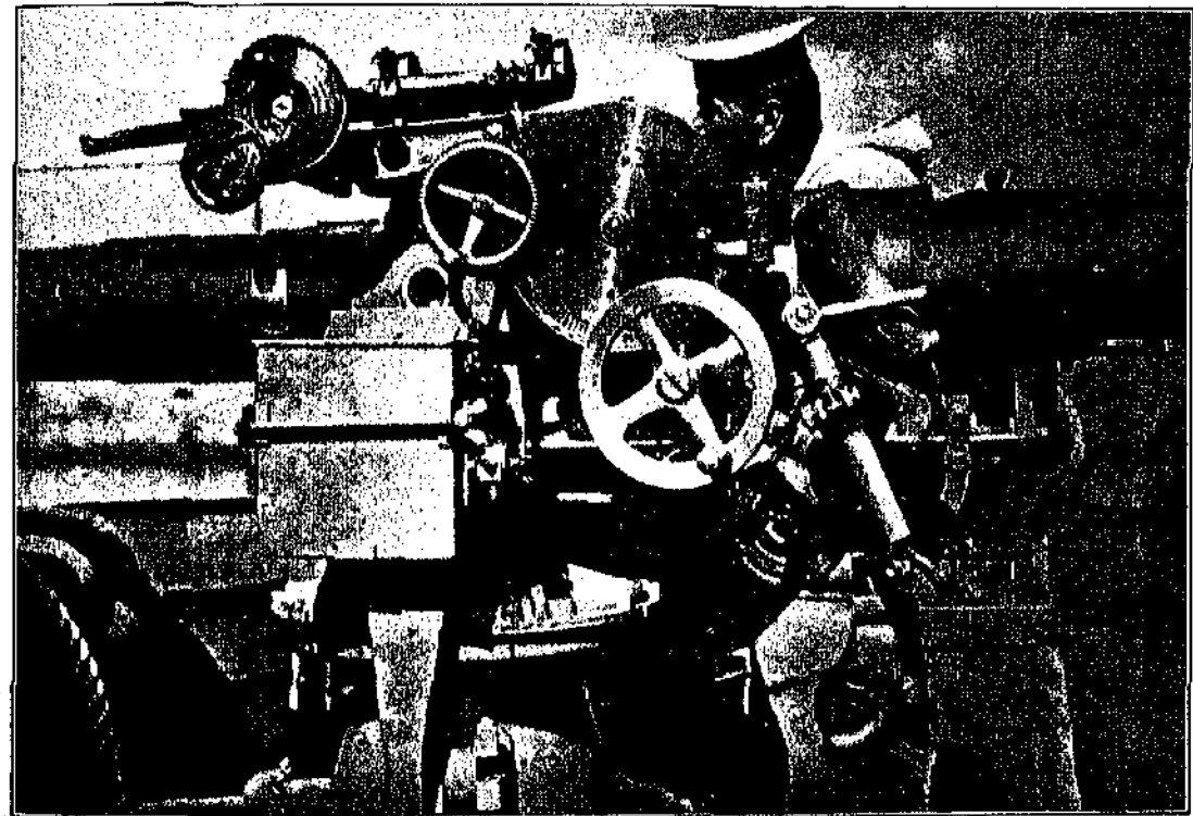
ΤΥΠΟΣ ΤΕΛΕΙΟΠΟΙΗΜΕΝΟΥ ΑΓΓΛΙΚΟΥ ΥΠΕΡΒΑΡΩΤΗ ΤΩΝ 12 ΔΑΚΤΥΛΩΝ
