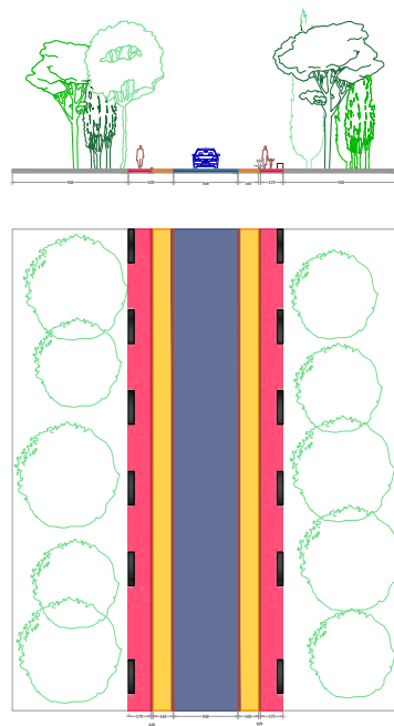
τομή αξονικής διαδρομής- σε προβολή με κάτοψη
