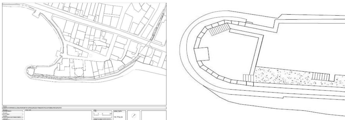
Αρχείο, ΕΦ.Α. Κάτοψη του ανατολικού λιμενοβραχίονα και λεπτομέρεια κάτοψης του προμαχώνα του Φάρου
