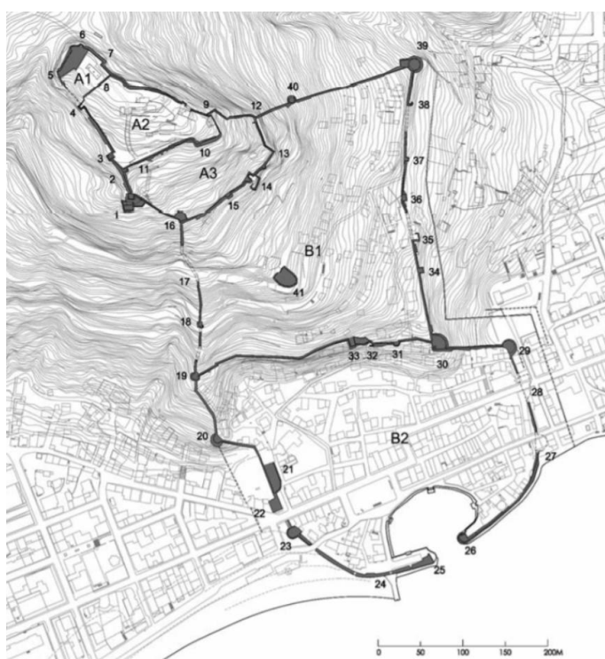
Αρχείο/ΕΦΑ.ΑΙΤ./ΑΚΑΡΝΑΝΙΑΣ. Σχ.1: Κάτοψη του κάστρου
