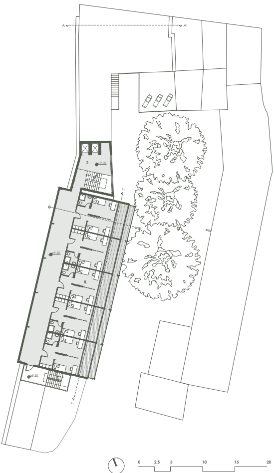
κατόψη 3 ου - 5 ου ορόφου
