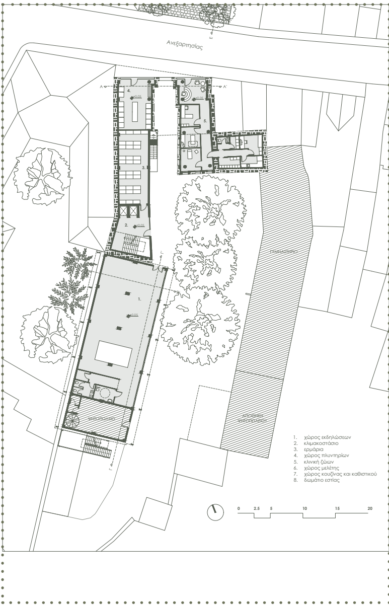
κατόψη ισογείου
