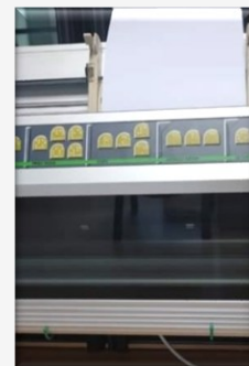
Εκτυπωτής ανάγλυφης αποτύπωσης Braille
