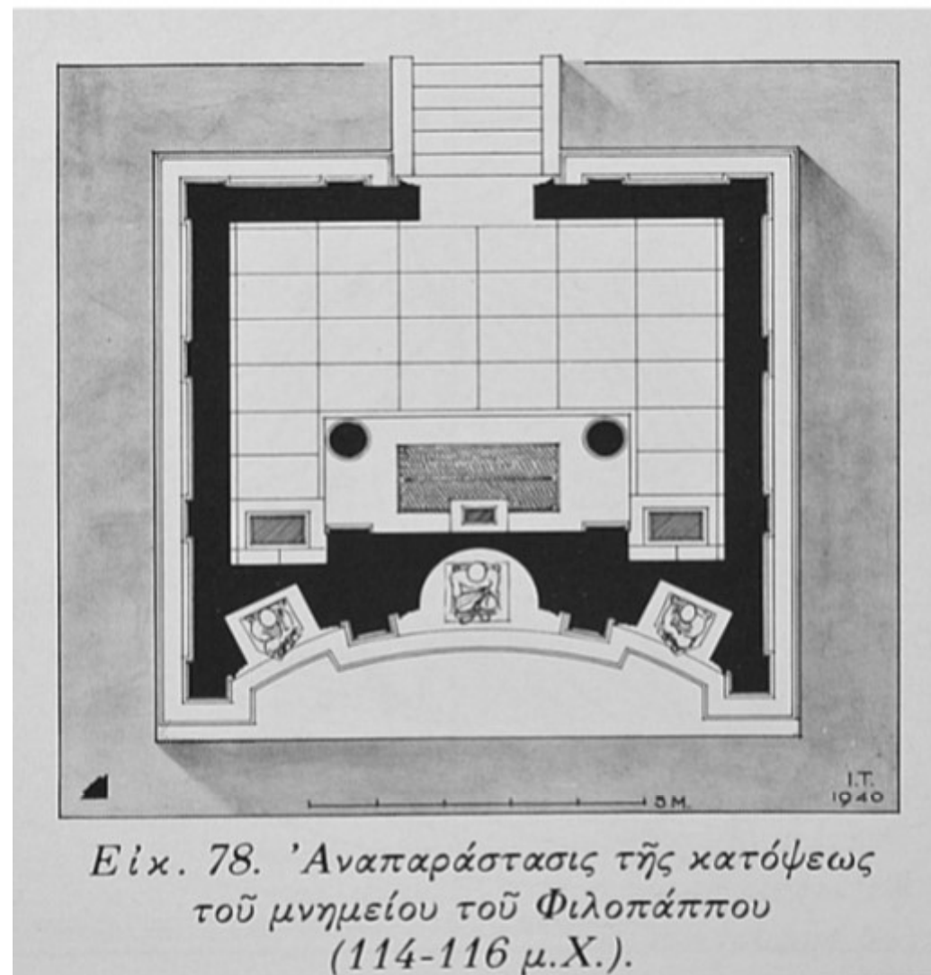
Αναπαράσταση της κάτοψης του μνημείου του Φιλοπάππου από τον Ι. Τραυλό.
