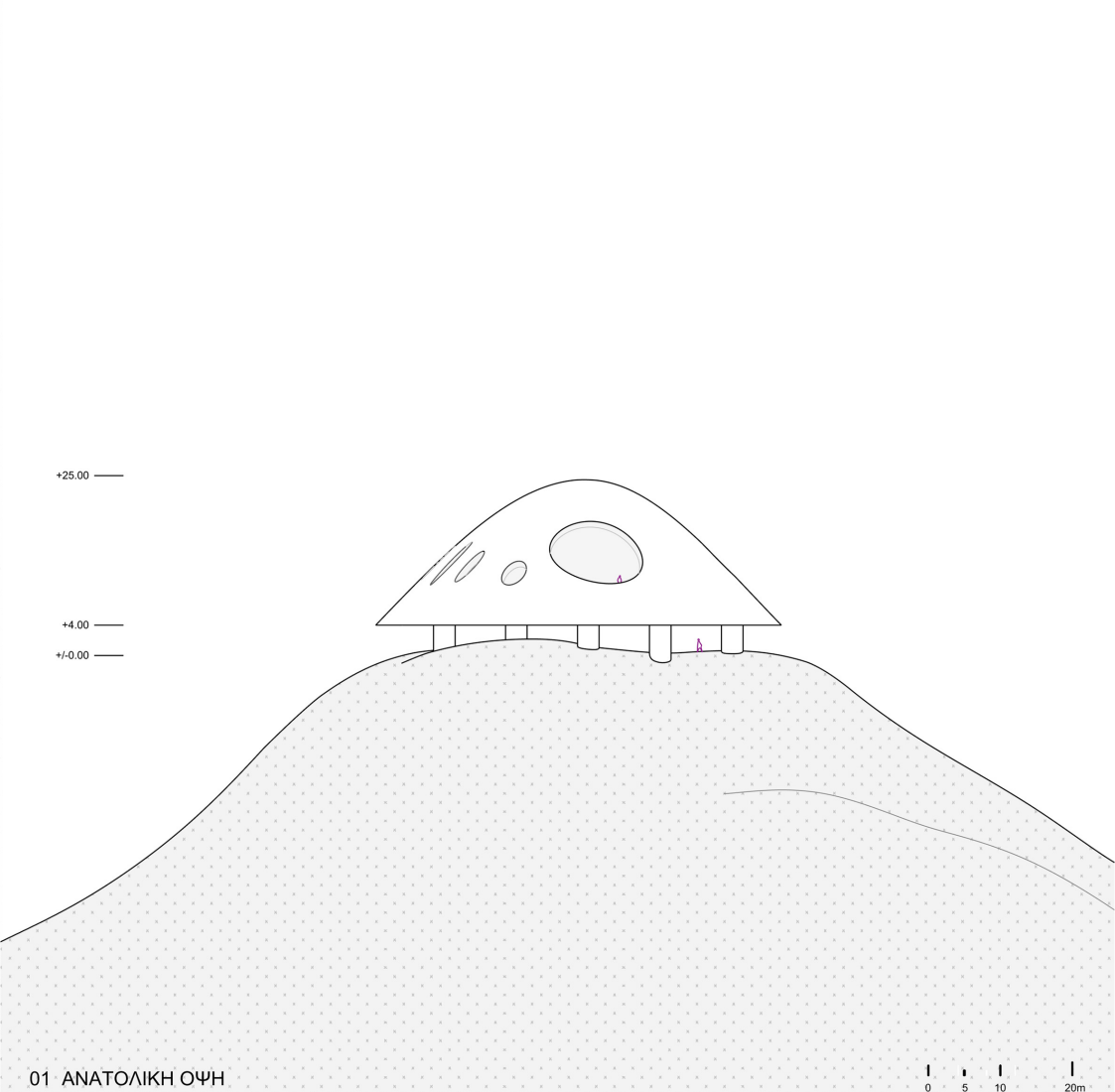
01 ΑΝΑΤΟΛΙΚΗ ΟΨΗ
