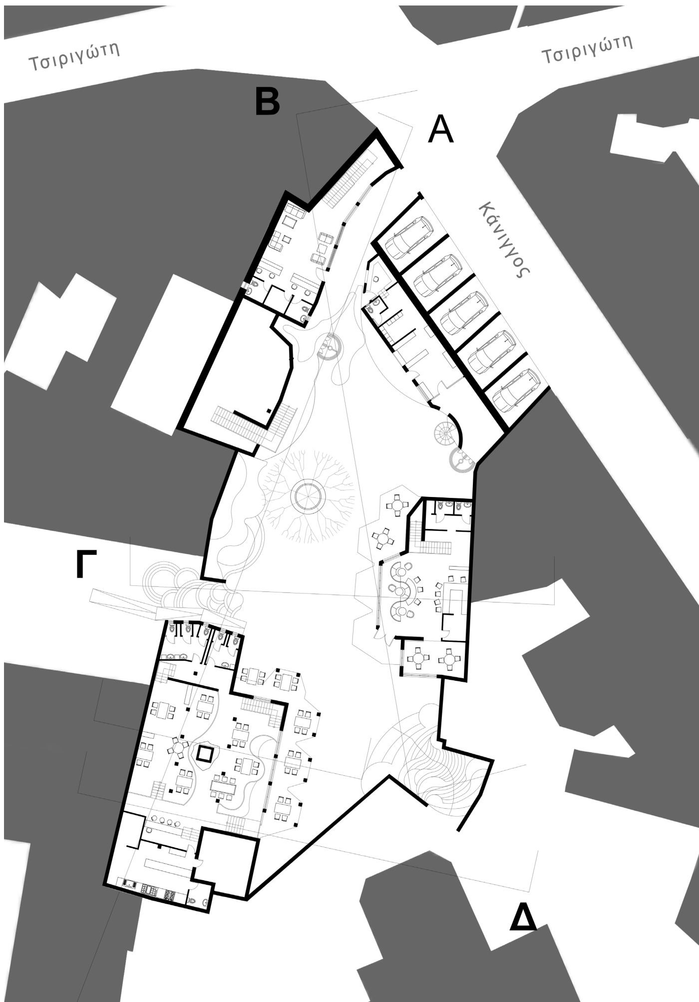
εικ.21 Κάτοψη ισογείου της πρότασης
