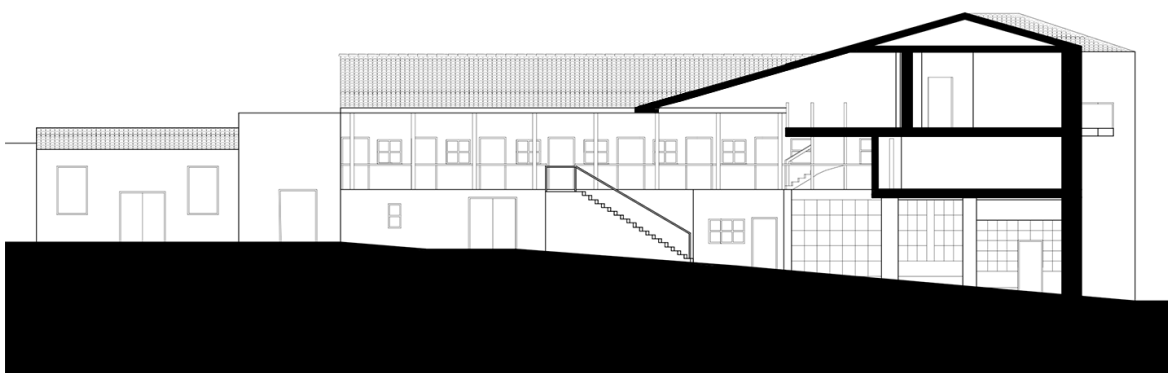
εικ.18 Η βόρειοανατολική όψη του κτίσματος του χανιού με μέρος της τομής του οικοπέδου
