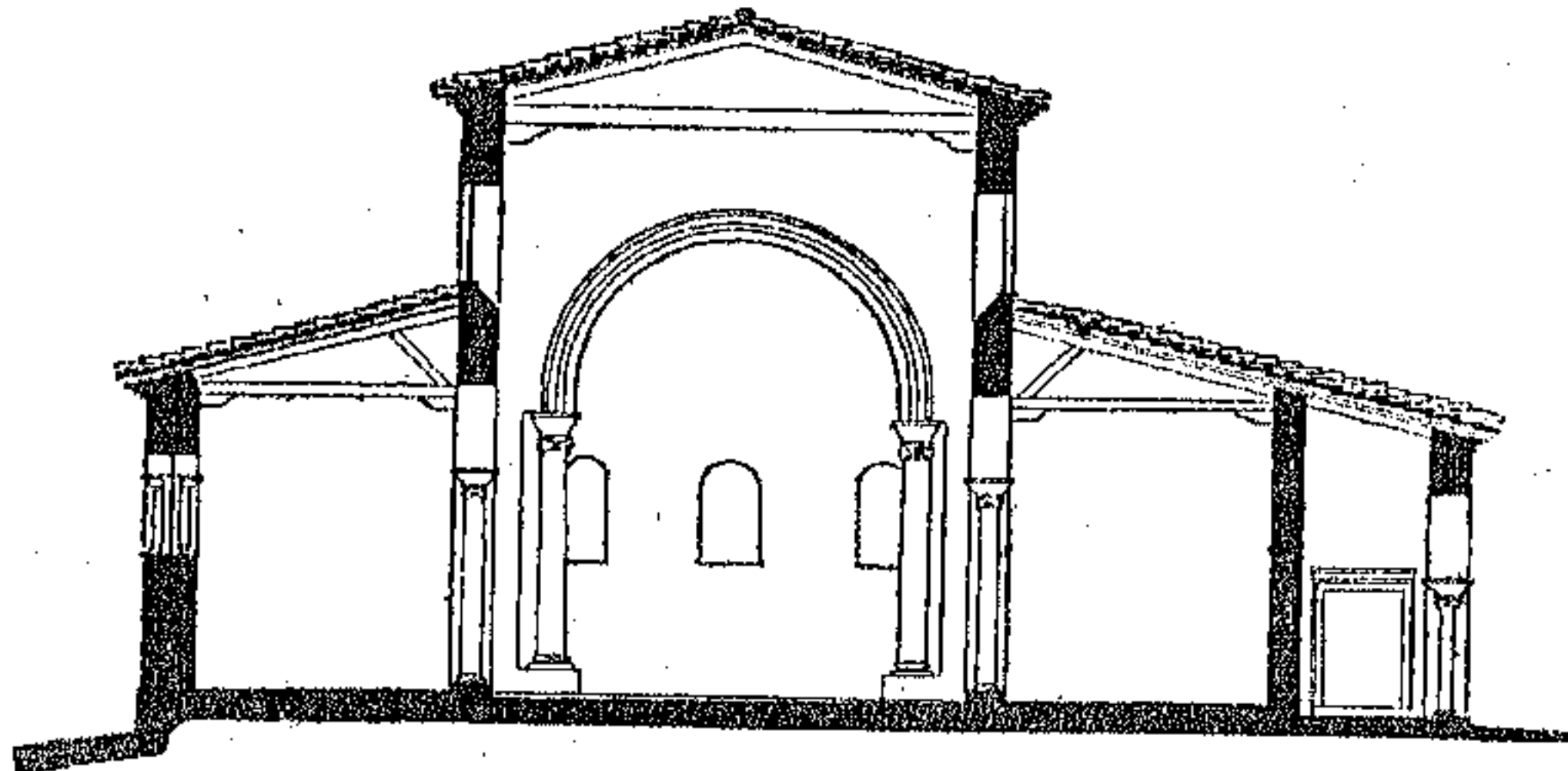
Τομὴ κατὰ πλάτος τῆς αὐτῆς Βασιλικῆς. (Εἰς τὸ βάθος φαίνεται καθαρὰ ἡ μεγαλοπρεπὴς Ἄψις τῆς Κόγχης. Εἰς τὸ δεξιὸν ἄκρον διακρίνεται ἐπίσης ἡ εἴσοδος μικροῦ παρεκκλήσιου).
