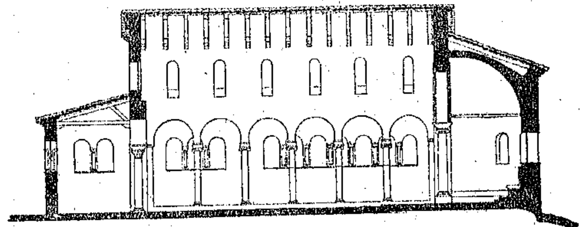
Τομὴ κατὰ μῆκος Παλαιοχριστιανικῆς Βασιλικῆς μετὰ μονορόφου νάρθηκος (Πρόκειται περὶ Βασιλικῆς ἀπλῆς ἀνευ προνάρθου καὶ γυναικονότου)
