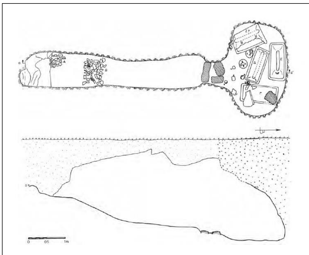
Εικόνα 150. Αγγελιανά Μυλοποτάμον. Κάτοψη θαλαμωτού τάφου.
