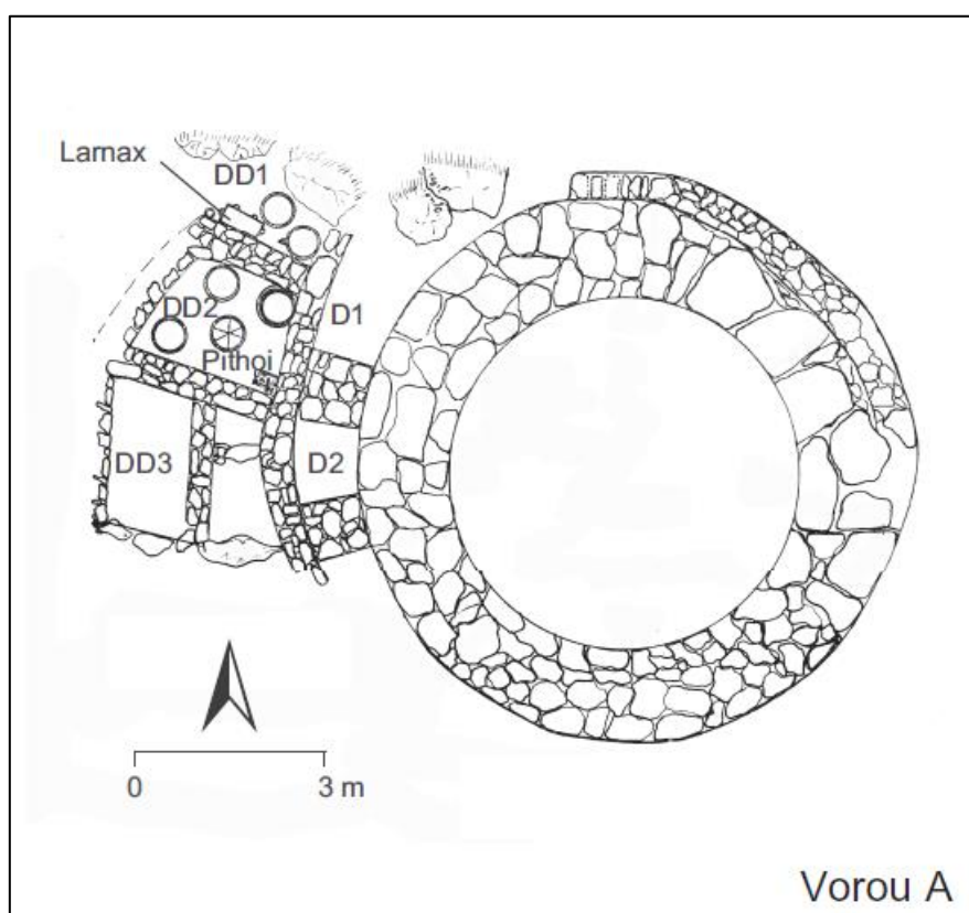
Εικόνα 85. Βορινά. Κάτοψη Θολωτού Α.
