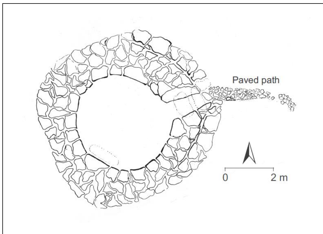
Εικόνα 112. Κράσι. Κάτοψη Θολωτού Α.
