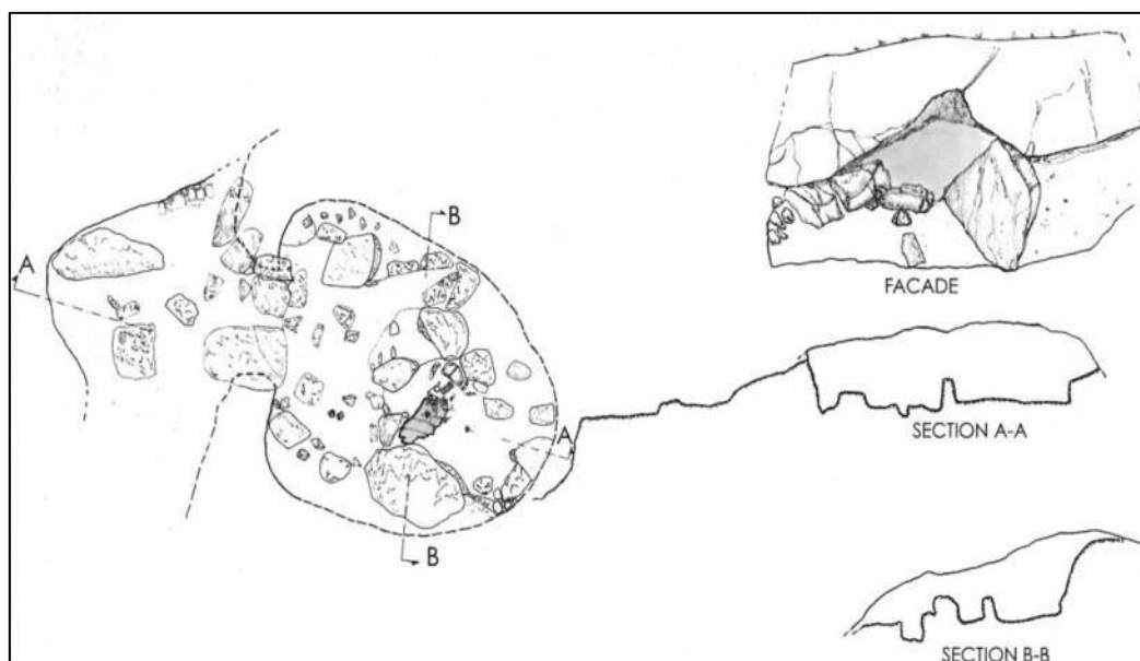
Εικόνα 145. Κερά Λιμανιώτισσα. Κάτοψη του τάφου.
