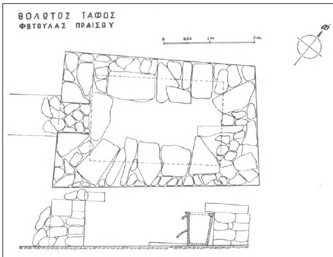
Εικόνα 51. Φωτούλα Πραισού. Κάτοψη θολωτού τάφου.
