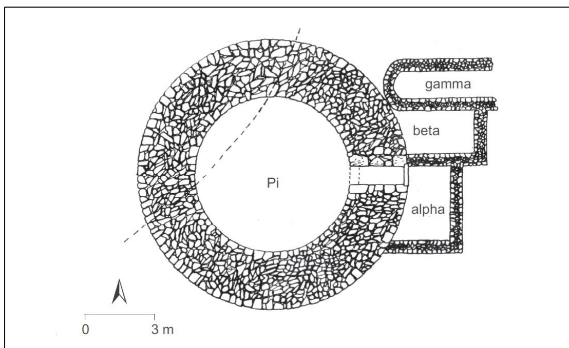
Εικόνα 80. Πορτί. Κάτοψη Θολωτού Π.
