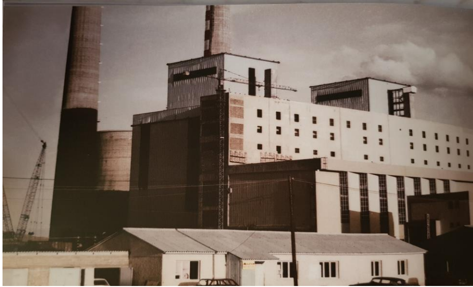
Εικόνα 15: ΑΗΣ Πτολεμαΐδας με την 1 και 2 μονάδα ισχύος 70 MW και 125 MW 1962. Συλλογή Ιωάννη Τσιομπάνου.
