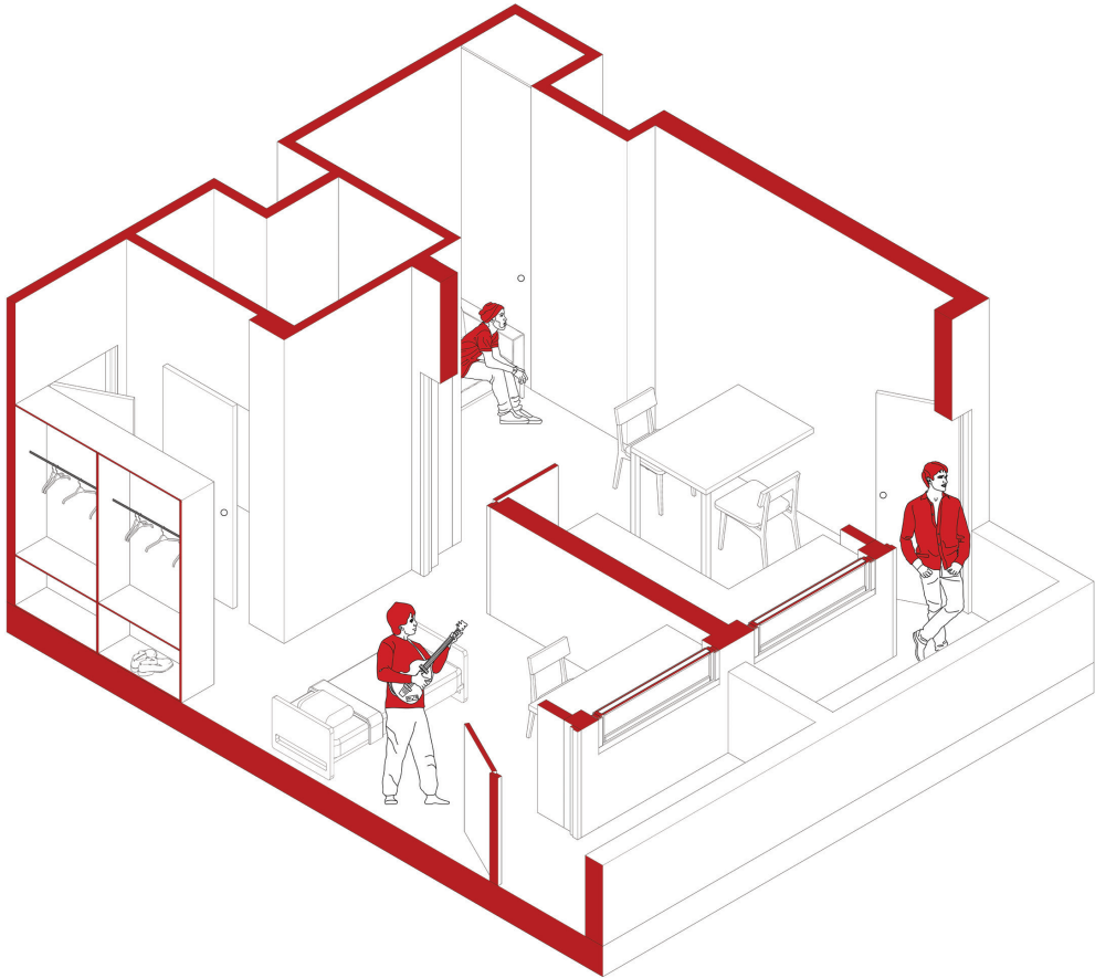
Εικ. 37 Πτέρυγα Γ' εστιών Πανεπιστημίου, δωμάτιο 24 τ.μ.
