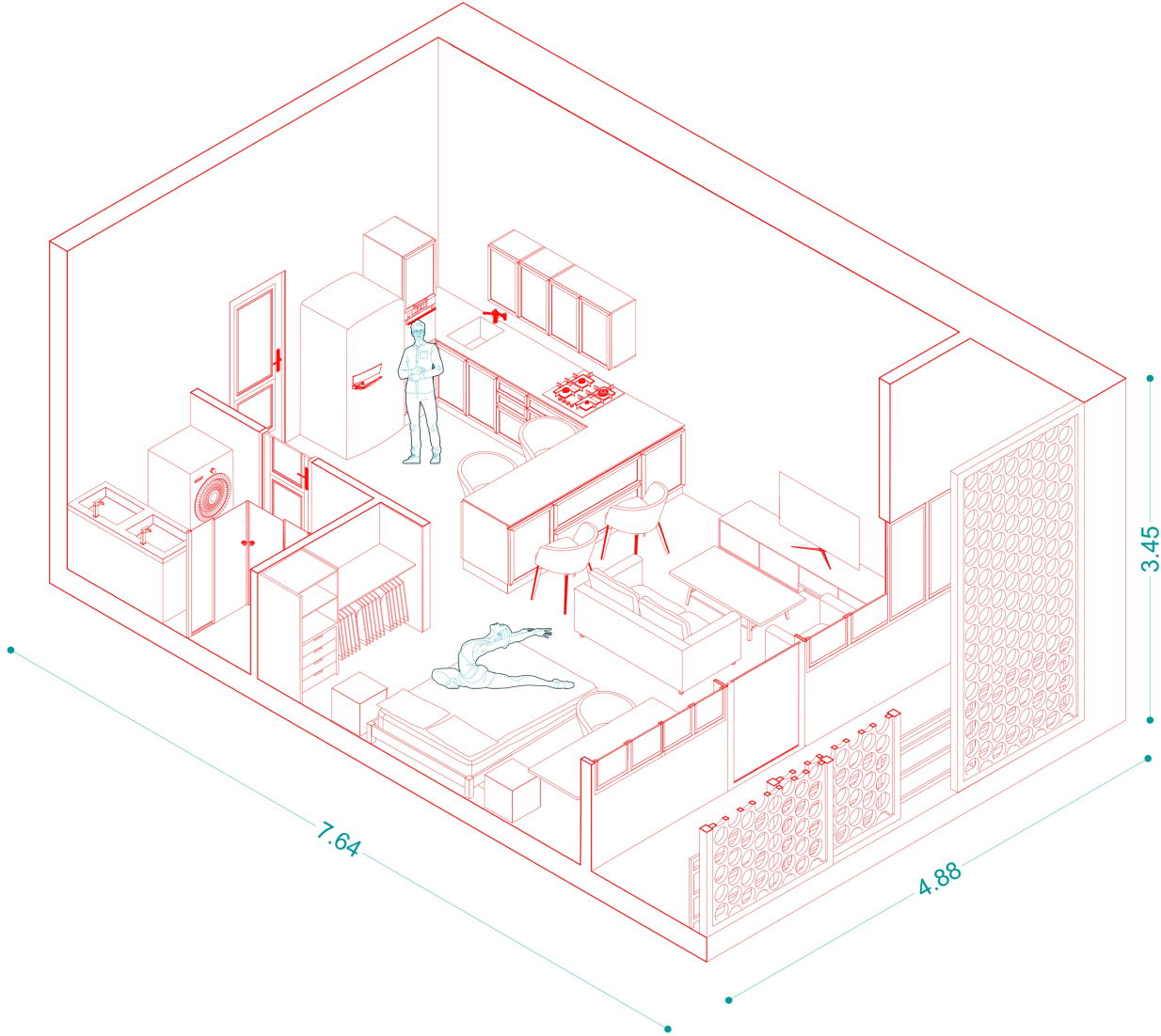
Εικ. 101 Δωμάτιο 50 τ.μ.
