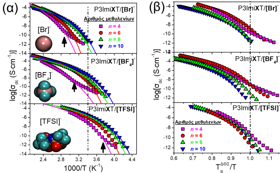
Σχήμα 8.13. (α) Dc-αγωγιμότητα των πολυμερικών ηλεκτρολυτών βασιζόμενων σε πολυθειοφαινεία με διαφορετικά μήκη της πλευρικής ομάδας και σταθερά ανιόντα: (πάνω) [\text{Br}^-] , (μέση) [\text{BF}_4^-] και (κάτω) [\text{TFSI}^-] , κατά τη θέρμανση. Οι συνεχείς γραμμές είναι προσομοιώσεις της VFT εξίσωσης για την αγωγιμότητα (Εξ. 8.2). Τα βέλη δείχνουν τη θερμοκρασία αποσύζευξης για τους αντίστοιχους P3lmiBT πολυηλεκτρολύτες. (β) Η dc-αγωγιμότητα σαν συνάρτηση της ανοιγμένης θερμοκρασίας για διαφορετικά μήκη της πλευρικής ομάδας και σταθερό ανιόν: [\text{Br}^-] (πάνω), [\text{BF}_4^-] (μέση) και [\text{TFSI}^-] (κάτω), κατά τη θέρμανση. Χρησιμοποιήθηκαν οι τιμές της θερμοκρασίας υάλου από τη Διαφορική Θερμιδομετρία Σάρωσης. Από τις αναφορές [7,8].
