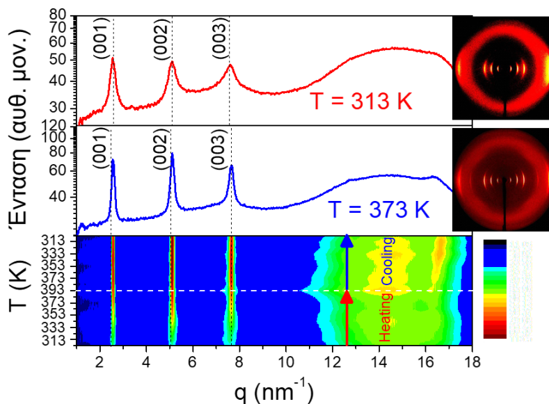
Σχήμα 8.19. Διαγράμματα WAXS για τον ηλεκτρολύτη του τύπου P3ImiHT με ανιόν [BF_4]^- σε δύο θερμοκρασίες: 313 K (πάνω) και 373 K (μέση), κατά τη θέρμανση. Οι διακεκομμένες γραμμές δίνουν τη θέση και τους (hkl) δείκτες από τις ανακλάσεις Bragg που αντιστοιχούν στη φυλλοειδή μορφολογία. Επίσης, δείχνονται οι διδιάστατες εικόνες WAXS από προσανατολισμένη ίνα στις αντίστοιχες θερμοκρασίες. (Κάτω) Διδιάστατο γράφημα έντασης WAXS κατά τη θέρμανση και την ακόλουθη ψύξη. Από την αναφορά [7].
