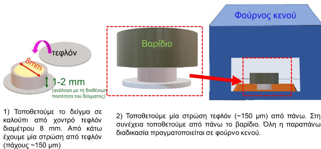
Σχήμα 5.29. Προετοιμασία του δείγματος σε μορφή φιλμ με ομοιόμορφο πάχος (1-2 mm) για τις μετρήσεις της ρεολογίας.
