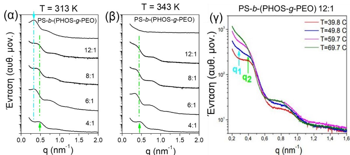
Σχήμα 7.6. (α), (β) Διαγράμματα SAXS του καθαρού \text{PS-b-(PHOS-g-PEO)} (πάνω) και του ηλεκτρολύτη του με \text{LiCF}_3\text{SO}_3 , σε δύο θερμοκρασίες κάτω και πάνω από την θερμοκρασία τήξης του PEO: 313 \text{ K} (αριστερά) και 343 \text{ K} (δεξιά). (γ) Διαγράμματα SAXS του ηλεκτρολύτη \text{PS-b-(PHOS-g-PEO)/LiCF}_3\text{SO}_3 με συγκέντρωση άλατος [\text{EO}]:[\text{Li}^+] = 12:1 ως συνάρτηση της θερμοκρασίας. Τα βέλη και οι γραμμές δίνουν τις θέσεις κορυφής του κρυσταλλικού PEO (μπλε) και του συμπλόκου (πράσινο), αντίστοιχα. Από την αναφορά [4].
