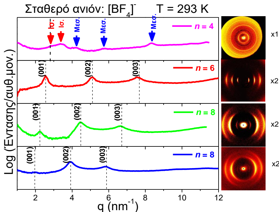
Σχήμα 8.10. Διαγράμματα WAXS για τους πολυηλεκτρολύτες βασιζόμενους σε κατιονικά πολυθειοφαινία με σταθερό ανιόν [\text{BF}_4]^- και διαφορετικά μήκη της πλευρικής ομάδας; n = 4 (ματζέντα γραμμή), n = 6 (κόκκινη γραμμή), n = 8 (πράσινη γραμμή) και n = 10 (μπλε γραμμή) σε θερμοκρασία 293 K. Οι διακεκομμένες γραμμές δίνουν τις θέσεις και τους δείκτες (hkl) από τις ανακλάσεις Bragg που αντιστοιχούν σε μία φυλλοειδή μορφολογία. Τα βέλη δείχνουν τις θέσεις των μεσημβρινών (μπλε κάθετα βέλη) και ισημερινών (κόκκινα κάθετα βέλη) ανακλάσεων του ηλεκτρολύτη P3ImiBT/ [\text{BF}_4]^- . Δεξιά, απεικονίζονται οι διδιάστατες εικόνες WAXS, των αντίστοιχων ηλεκτρολυτών, από προσανατολισμένες ίνες. Από την αναφορά [8].
