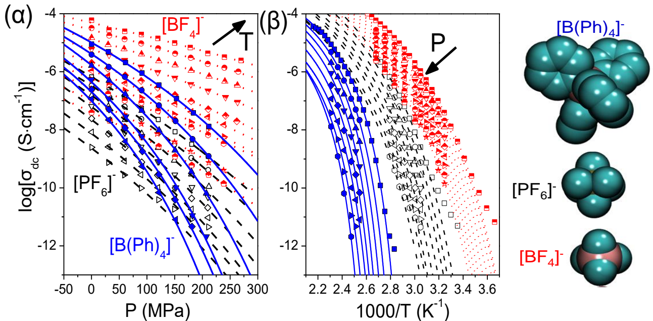
Σχήμα 8.24. (α) Εξάρτηση από την πίεση της dc-αγωγιμότητας για τους πολυμερικούς ηλεκτρολύτες του τύπου P31miHT με ανιόντα: [\text{BF}_4]^- (κόκκινα σύμβολα), [\text{PF}_6]^- (μαύρα σύμβολα) και [\text{B(Ph)}_4]^- (μπλε σύμβολα) στο θερμοκρασιακό εύρος (P31miHT/ [\text{BF}_4]^- ; από 308 έως 373 K, P31miHT/ [\text{PF}_6]^- ; από 328 έως 358 K και P31miHT/ [\text{B(Ph)}_4]^- ; από 393 έως 433 K. Οι συνεχείς, διακεκομμένες και με τελείες γραμμές είναι προσομοιώσεις της Εξ. 8.4 για τους ηλεκτρολύτες του τύπου P31miHT με [\text{B(Ph)}_4]^- , [\text{PF}_6]^- and [\text{BF}_4]^- ανιόντα, αντίστοιχα. (β) Θερμοκρασιακή εξάρτηση της dc-αγωγιμότητας κάτω από “ισοβαρείς” συνθήκες. Η πίεση αυξάνεται κατά την κατεύθυνση του βέλους: P = 0.1 \text{ MPa} (τετράγωνα), P = 30 \text{ MPa} (κύκλοι), P = 60 \text{ MPa} (πάνω-τρίγωνα), P = 90 \text{ MPa} (κάτω-τρίγωνα), P = 120 \text{ MPa} (ρόμβοι), P = 150 \text{ MPa} (αριστερά-τρίγωνα), P = 180 \text{ MPa} (δεξιά-τρίγωνα), P = 210 \text{ MPa} (εξάγωνα), P = 240 \text{ MPa} (αστέρια) and P = 270 \text{ MPa} (πεντάγωνα). Οι συνεχείς, διακεκομμένες και με τελείες γραμμές είναι προσομοιώσεις της Εξ. 8.5 για τους πολυμερικούς ηλεκτρολύτες του τύπου: P31miHT/ [\text{B(Ph)}_4]^- , P31miHT/ [\text{PF}_6]^- και P31miHT/ [\text{BF}_4]^- , αντίστοιχα. Από την αναφορά [8].
