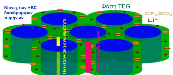
Σχήμα 4.5. Σχηματική αναπαράσταση της εξαγωνικής μοναδιαίας κυψελίδας για τα υπό διερεύνηση HBC-TEG/LiCF 3 SO 3 . Τα κάθετα βέλη δείχνουν τις φάσεις που είναι υπεύθυνες για την ηλεκτρονιακή και ιοντική αγωγιμότητα. Από την αναφορά [31].
