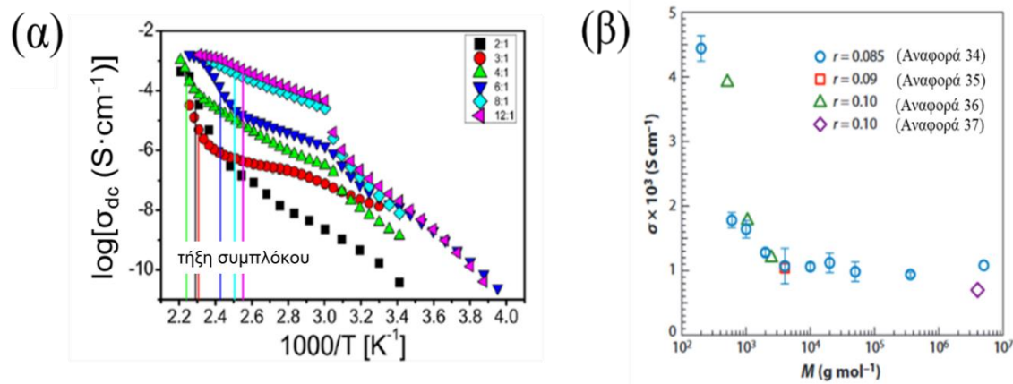
Σχήμα 1.8. (α) Θερμοκρασιακή εξάρτηση της dc-ιοντικής αγωγιμότητας για το σύστημα PEO/LiCF 3 SO 3 (με M_w PEO = 14 kg·mol -1 ) με συγκεντρώσεις [EO]:[Li + ] μεταξύ 12:1 και 2:1. Από την αναφορά [30]. (β) Ιοντική αγωγιμότητα ως συνάρτηση του μοριακού βάρους PEO για διάφορες συγκεντρώσεις άλατος LiN(CF 3 SO 3 ) 2 (LiTFSI), r = [Li]:[EO] . Από την αναφορά [33].
