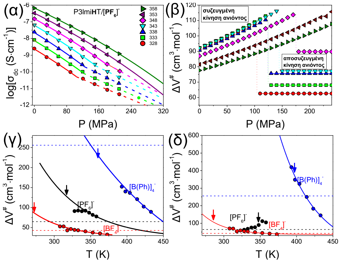
Σχήμα 8.26. (α) Εξάρτηση από την πίεση της dc -αγωγιμότητας για τον πολυηλεκτρολύτη P3ImiHT/[PF_6]^- στο θερμοκρασιακό εύρος από 328 έως 358 K με βήμα 5 K, κατά την ψύξη. (β) “Φαινόμενο” όγκος ενεργοποίησης ως συνάρτηση της πίεσης στις ίδιες θερμοκρασίες. Οι διακεκομμένες και συνεχείς γραμμές είναι προσομοιώσεις της VFT εξίσωσης (Εξ. 8.1) και της Arrhenius, αντίστοιχα. (γ, δ) “Φαινόμενο” όγκος ενεργοποίησης σε πίεση P = 0.1 MPa (γ) και P = 220 MPa (δ). Οι διακεκομμένες γραμμές αναπαριστούν μοριακούς όγκους που αντιστοιχούν στα ανιόντα: [BF_4]^- (κόκκινη γραμμή), [PF_6]^- (μαύρη γραμμή) και [B(Ph)_4]^- (μπλε γραμμή). Τα βέλη δείχνουν τις αντίστοιχες θερμοκρασίες υάλου σε πίεση (γ) P = 0.1 MPa και (δ) P = 220 MPa. Από την αναφορά [8].
