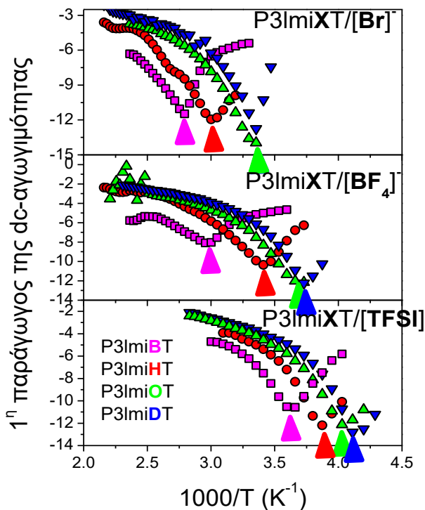
Σχήμα 8.14. Πρώτη παράγωγος της ιοντικής dc-αγωγιμότητας για τους πολυηλεκτρολύτες βασιζόμενους σε ΠΙΥ με διαφορετικά μήκη της πλευρικής ομάδας: n = 4 (ματζέ-ντα τρίγωνα), n = 6 (κόκκινοι κύκλοι), n = 8 (πράσινα πάνω-τρίγωνα) και n = 10 (μπλε κάτω-τρίγωνα) και σταθερά ανιόντα: (πάνω) [Br] - , (μέση) [BF 4 ] - και (κάτω) [TFSI] - , κατά τη θέρμανση. Τα αντίστοιχα βέλη υποδηλώνουν τη θερμοκρασία της μετάβασης, T_{\sigma 0} . Από την αναφορά [8].
