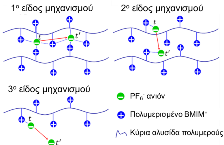
Σχήμα 3.17. Σχηματική αναπαράσταση των τριών ειδών μηχανισμών μεταφοράς του ιόντος που προτάθηκαν μέσω ατομιστικών προσομοιώσεων. Από την εργασία των Mogurampelly, Keith και Ganesan [44].
