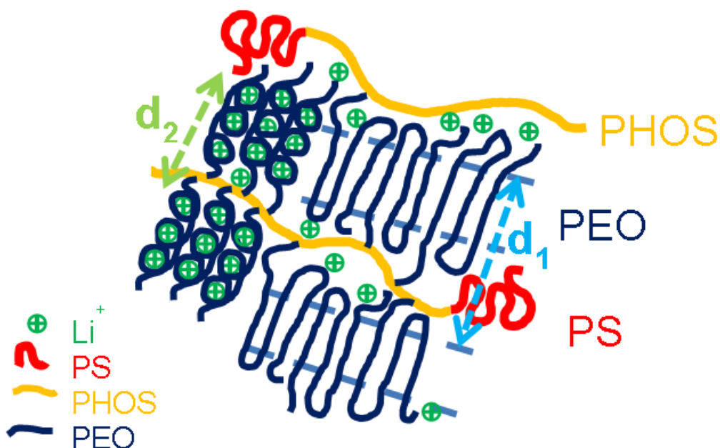
Σχήμα 7.7. Σχηματική απεικόνιση της δομής των πολυηλεκτρολυτών \text{PS-b-(PHOS-g-PEO)/LiCF}_3\text{SO}_3 με το κρυσταλλικό σύμπλοκο (αριστερά) και τις κρυσταλλικές περιοχές του PEO (δεξιά). Οι διακεκομμένες γραμμές δείχνουν την περιοχή του κρυσταλλικού PEO. Τα βέλη δείχνουν τις χαρακτηριστικές αποστάσεις συσχέτισης μεταξύ των κρυστάλλων του PEO ( d_1 ) και μεταξύ των κρυστάλλων του συμπλόκου ( d_2 ). Από την αναφορά [4].
