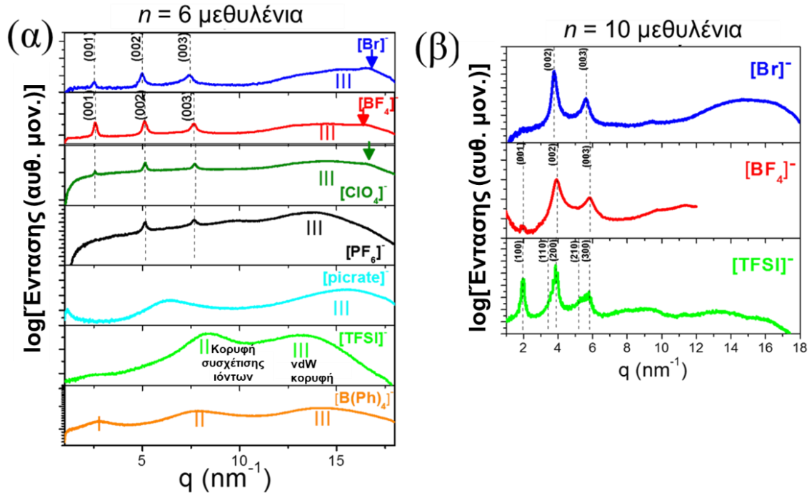
Σχήμα 8.16. Διαγράμματα WAXS για τους πολυμερικούς ηλεκτρολύτες με μήκος πλευρικής ομάδας (α) n = 6 και (β) n = 10 που φέρουν διαφορετικά μεγέθη ανιόντων: [Br]^- (μπλε), [BF_4]^- (κόκκινο), [ClO_4]^- (σκούρο πράσινο), [PF_6]^- (μαύρο), [picrate]^- (κυανό), [TFSI]^- (πράσινο) και [B(Ph)_4]^- (πορτοκαλί), σε θερμοκρασία 353 K. Οι διακεκομμένες γραμμές δίνουν τις θέσεις και τους (hkl) δείκτες από τις ανακλάσεις Bragg που αντιστοιχούν σε φυλλοειδή ή εξαγωνική μορφολογία. Τα βέλη δηλώνουν τη θέση της \pi^*-\pi^* στοίβαξης.
