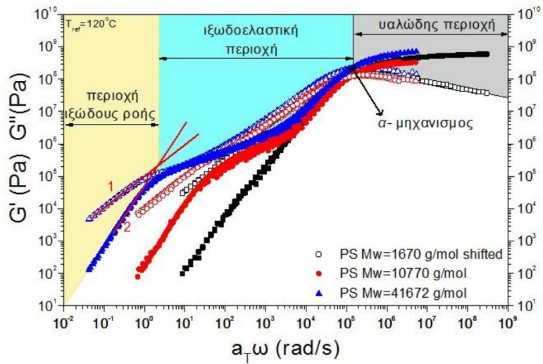
Σχήμα 5.31. Πραγματικό G' (κλειστά σημεία) και φανταστικό G'' (ανοιχτά σημεία) μέρος του μέτρου διάτμησης για πολυστυρένιο (PS) με διαφορετικά μοριακά βάρη. Διακρίνονται τρεις περιοχές: (δεξιά) υαλώδης, (μέση) ιξωδοελαστική και (αριστερά) περιοχή ιξώδους ροής. Ο άξονας των συχνοτήτων έχει μετατοπισθεί με παράγοντα, a_T(T) , ως προς τον \alpha -μηχανισμό. Από την αναφορά [30].
