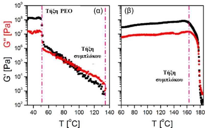
Σχήμα 1.10. Μέτρο αποθήκευσης (τετράγωνα) και απωλειών (κύκλοι) για τα συστήματα (α) (PEO)_{12}LiCF_3SO_3 και (β) (PEO)_4LiCF_3SO_3 ως συνάρτηση της θερμοκρασίας. Ο ρυθμός θέρμανσης είναι 2 K \cdot min^{-1} και η γωνιακή συχνότητα \omega = 10 rad \cdot s^{-1} . Από την αναφορά [30].
