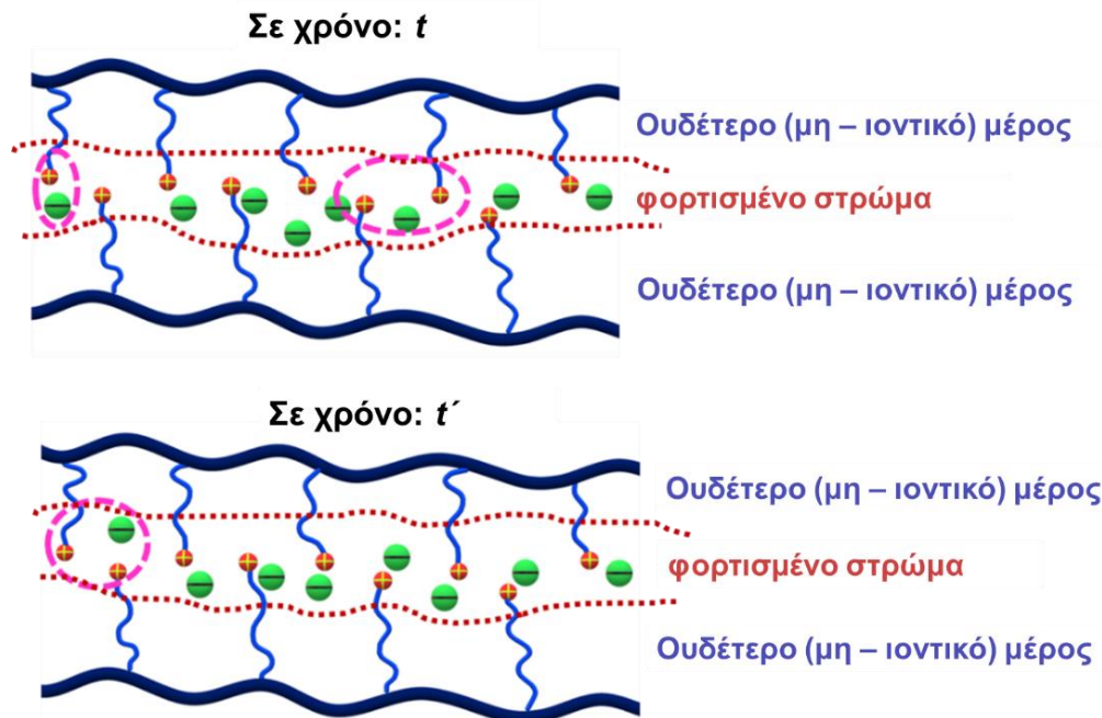
Σχήμα 8.29. Σχηματική απεικόνιση του μηχανισμού της κίνησης του ιόντος. Την χρονική στιγμή t , το ανιόν είναι συμπλεγμένο (“κολλημένο”) με το κατιόν για συγκεκριμένους τα χρόνους. Σε χρόνο t' , το ανιόν αποσυσχετίζεται από το κατιόν και πηδά σε μία απόσταση d_H/2 εντός του φορτισμένου στρώματος αυξάνοντας την dc -αγωγιμότητα. Από την αναφορά [8].
