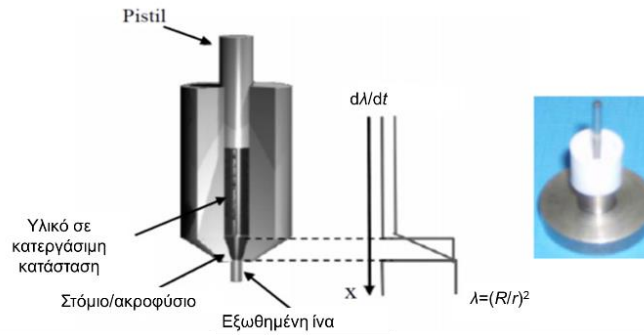
Σχήμα 5.23. Σχηματική απεικόνιση της διάταξης εξώθησης για την παραγωγή π.χ. προσανατολισμένων ιών δισκόμορφων υγρών κρυστάλλων. (δεξιά) Φωτογραφία του εξωθητή.
