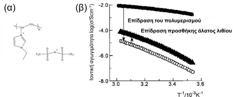
Σχήμα 3.4. (α) Χημική δομή του N -βινυλο-3-αιθυλο ιμιδαζόλιο εμπλουτισμένο με [TFSI] - . (β) Ιοντική αγωγιμότητα του ΙΥ (γεμάτοι κύκλοι), του ΠΙΥ (άδειοι κύκλοι) και ενός ισομοριακού ΠΙΥ εμπλουτισμένο με LiTFSI (γεμάτα πάνω-τρίγωνα). Από την αναφορά [7].
