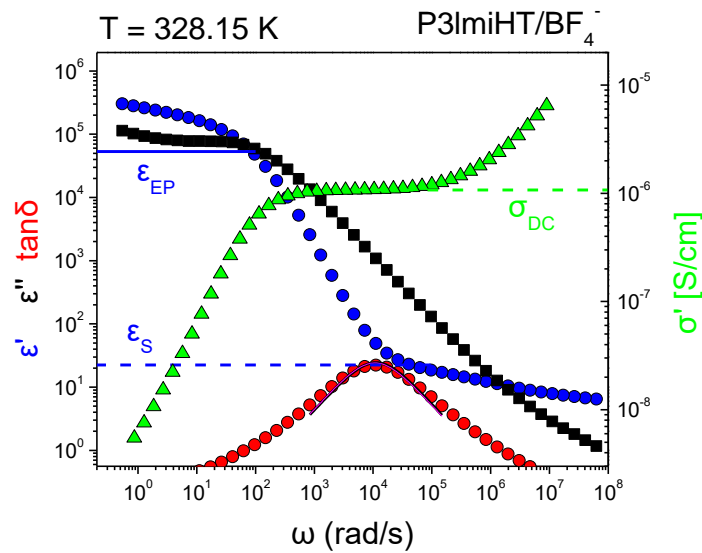
Σχήμα Α.1. Πραγματικό (μπλε κύκλοι) και φανταστικό (μαύρα τετράγωνα) μέρος της διηλεκτρικής διαπερατότητας, πραγματικό μέρος της μιγαδικής αγωγιμότητας (πράσινα πάνω- τρίγωνα) και η εφαπτομένη απωλειών (κόκκινοι κύκλοι) σαν συνάρτηση της γωνιακής συχνότητας. Οι συνεχείς, διακεκομμένες και με τελείες γραμμές δείχνουν τα \epsilon_{EP} , \epsilon_s και \sigma_{DC} , αντίστοιχα.
