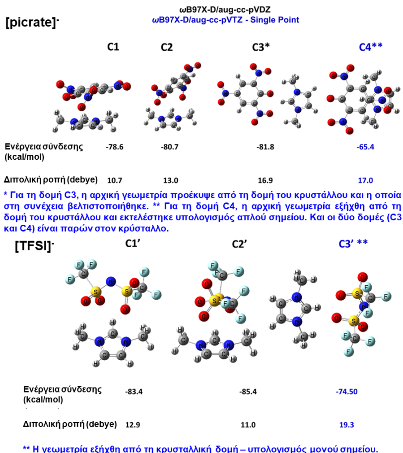
Σχήμα 8.4. Η εικονική αναπαράσταση, οι ενέργειες σύνδεσης και οι διπολικές ροπές των βελτιστοποιημένων δομών των ιοντικών ζευγών [\text{dmim}][\text{picrate}] και [\text{dmim}][\text{TFSI}] . Από την αναφορά [8].
