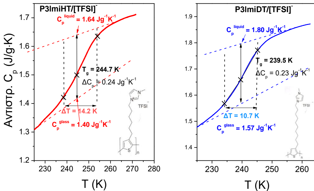
Σχήμα 5.21. Θερμοκρασιακή εξάρτηση της αντιστρεπτής συνιστώσας της θερμοχωρητικότητας για δύο πολυηλεκτρολύτες (αριστερά) P3ImiHT/[TFSI] και (δεξιά) P3ImiDT/[TFSI]. Η χημική δομή των ηλεκτρολυτών απεικονίζεται στο ένθετο. Από το μοντέλο του Donth 23 υπολογίστηκε η χαρακτηριστική κλίμακα μήκους που σχετίζεται με τη θερμοκρασία υάλου (Εξ. 5.57), όπως θα αναφέρουμε στο Κεφάλαιο 8.
