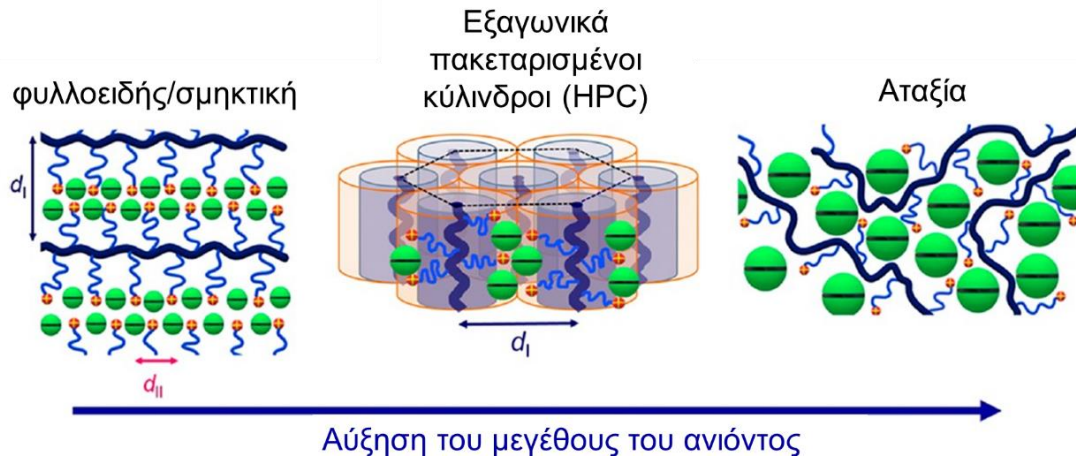
Σχήμα 8.17. Σχηματική αναπαράσταση της (α) φυλλοειδούς και (β) εξαγωγικής μοναδιαίας κοψελίδας. Επίσης απεικονίζονται το πάχος της νανοδομής, d_I , και η απόσταση συσχέτισης μεταξύ των ιόντων ίδιου φορτίου ( d_{II} ). Από την αναφορά [8].
