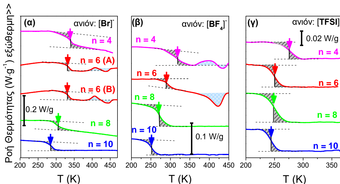
Σχήμα 8.7. Θερμογραφήματα \Delta\Theta\Sigma για τους πολυμερικούς ηλεκτρολύτες βασιζόμενους σε ΠΙΥ με κύρια αλυσίδα από πολυθειοφαινίου με διαφορετικά μήκη των πλευρικών ομάδων ( n = 4, 6, 8 and 10 ) και σταθερό ανιόν: (α) [\text{Br}]^- , (β) [\text{BF}_4]^- και (γ) [\text{TFSI}]^- . Οι μετρήσεις αναφέρονται στο δεύτερο κύκλο θέρμανσης με ρυθμό 10 \text{ K}\cdot\text{min}^{-1} . Τα θερμογραφήματα είναι μετατοπισμένα κατακόρυφα. Τα βέλη υποδεικνύουν τη θερμοκρασία υάλου. Από τις αναφορές [7,8].
