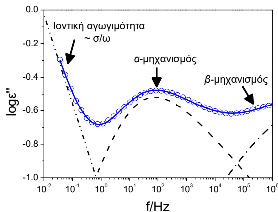
Σχήμα 5.15: Το φανταστικό μέρος ( \epsilon'' , O) της σύνθετης διηλεκτρικής συνάρτησης, \epsilon^*(\omega) , συναρτήσει της συχνότητας για το καθαρό HBC-TEG6, στους T = 243 K. Ο \beta -μηχανισμός εμφανίζεται στις υψηλότερες συχνότητες. Σε πιο χαμηλές συχνότητες εμφανίζεται ο \alpha -μηχανισμός, και σε ακόμη πιο χαμηλές συχνότητες εμφανίζεται η ιοντική αγωγιμότητα ( \sim \sigma/\omega ). Η συνεχής γραμμή είναι το άθροισμα δύο μηχανισμών τύπου HN και της συνεισφοράς της αγωγιμότητας.
