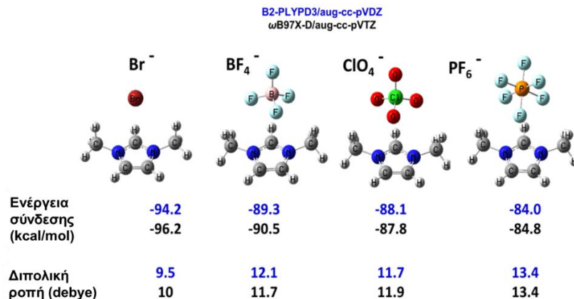
Σχήμα 8.3. Εικονογραφημένη αναπαράσταση, οι ενέργειες σύνδεσης και οι διπολικές ροπές των βελτιστοποιημένων δομών των ιοντικών ζευγών [\text{dmim}][\text{Br}] , [\text{dmim}][\text{BF}_4] , [\text{dmim}][\text{ClO}_4] and [\text{dmim}][\text{PF}_6] . Από την αναφορά [8].
