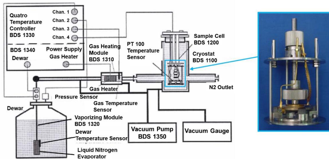
Σχήμα 5.10: (αριστερά) Η πειραματική διάταξη του συστήματος διηλεκτρικής φασματοσκοπίας με μεταβαλλόμενη θερμοκρασία υπό ατμοσφαιρική πίεση, μαζί με το σύστημα ελέγχου θερμοκρασίας, (δεξιά) μεγέθυνση τμήματος της κυψελίδας με τα δύο ηλεκτρόδια.
