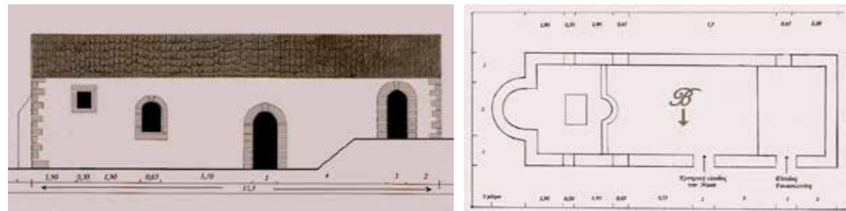
Εικόνα 42, 43. Όψη της βόρειας πλευράς και κάτοψη του Αγίου Γεωργίου. Πηγή: Ο ναός του Αγίου Γεωργίου, βιβλίο του Ιωάννη Θεριανού, Δήμος Λευκάδας 2013
