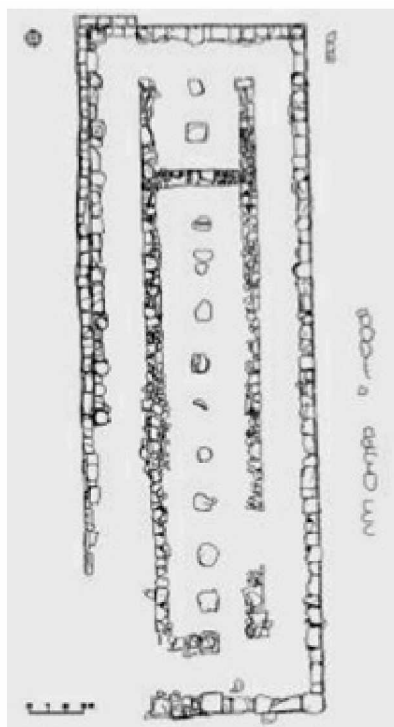
Εικ. 15. α. Ο πρώτος ναός του Απόλλωνος (τελευταίο τέταρτο του 7 ου αι. π.Χ.) β. Ο ναός του Απόλλωνος μετά από την προσθήκη περιστυλίου, τέλη 3 ου - αρχές 2 ου αι. π.Χ.
