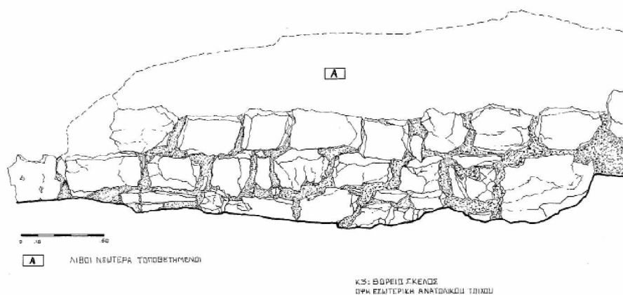
Εικ. 22. Κτίσμα Κ3. Τμήμα εσωτ. όψης ανατολικού τοίχου (σχ. Ελ. Μπούσδρα).
