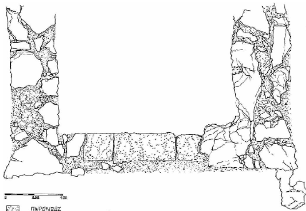
Εικ. 23. Κτίσμα Κ3. Κάτοψη νότιας στενής πλευράς (σχ. Ελ. Μπούσδρα).
