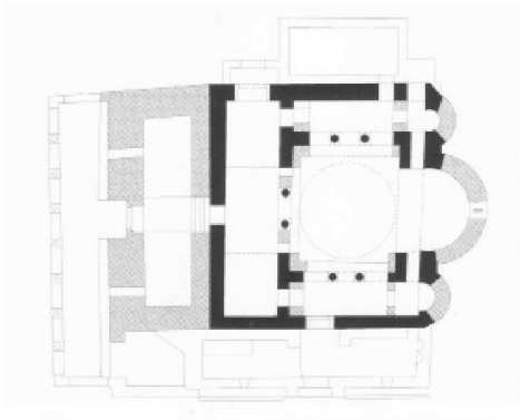
Εικ. 1. Άνω Λάμποβο, ναός της Κοιμήσεως της Θεοτόκου. Κάτοψη (Curcic, 2010, 320).
