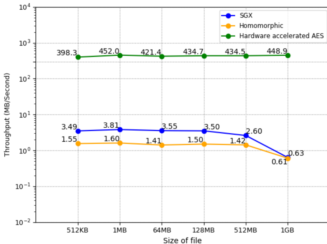
Σχήμα 5.2: Ρυθμαπόδοση κρυπτογράφησης.
