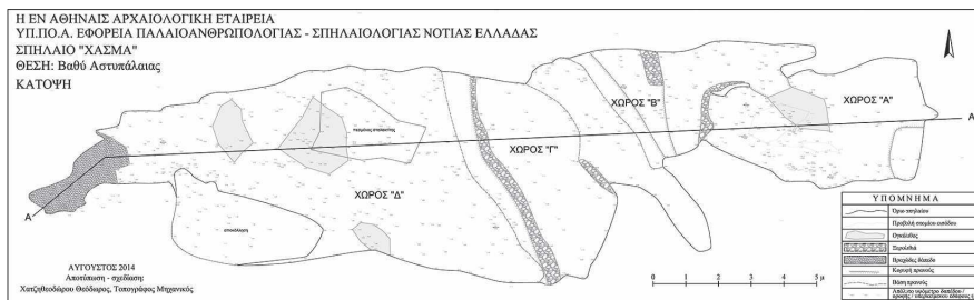
Εικ. 40. Σπηλαιοβάραθρο Χάσμα. Σχεδιαστική αποτύπωση Θ. Χατζηθεοδώρου
