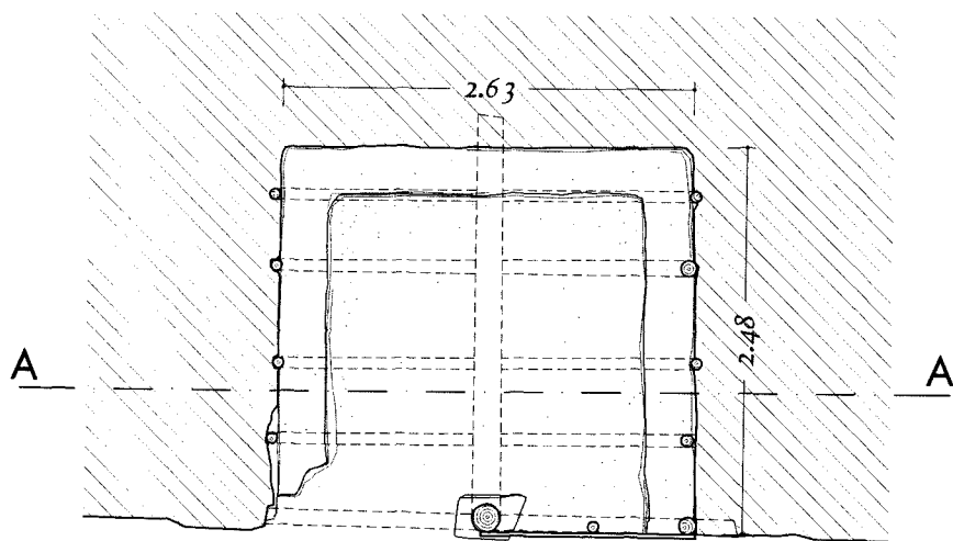
ΚΑΤΟΨΗ
