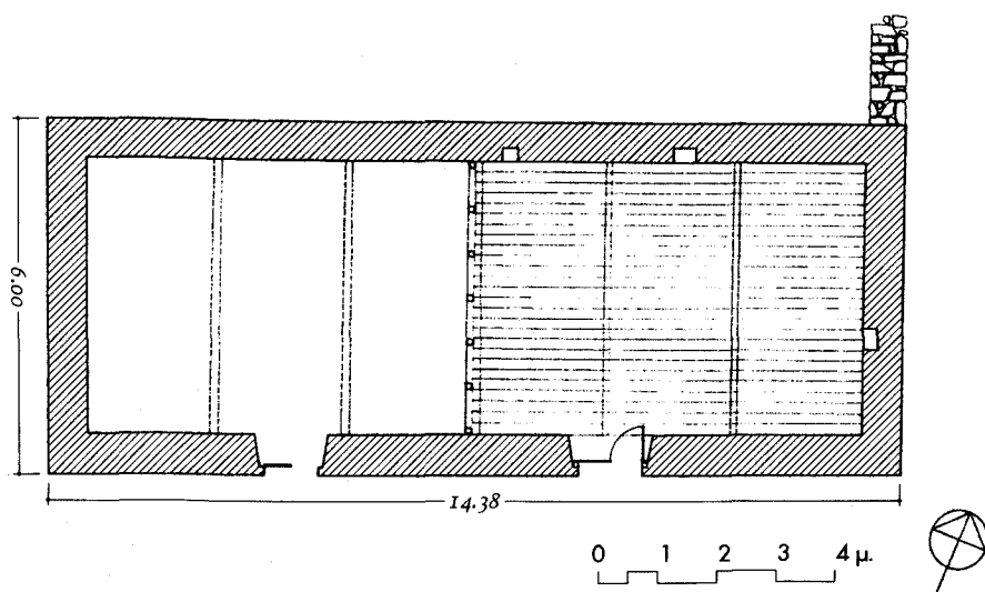
18. Κάτοψη χαμοκέλας στο Λεσοβίτι (σπίτι 13α).
