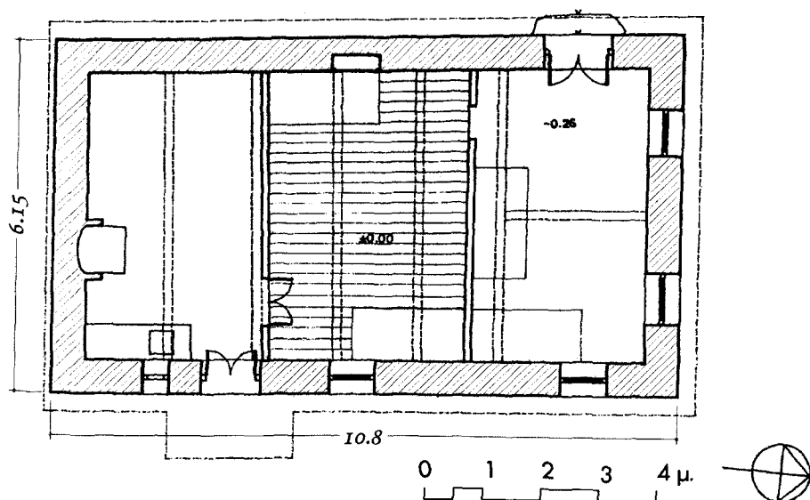
20. Κάτοψη νεότερου καλυβιού στους Παιδεμένους (σπίτι 49).
