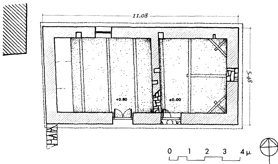
19. Κάτοψη χαμοκέλας στο Λυκουδέσι (σπίτι 32).
