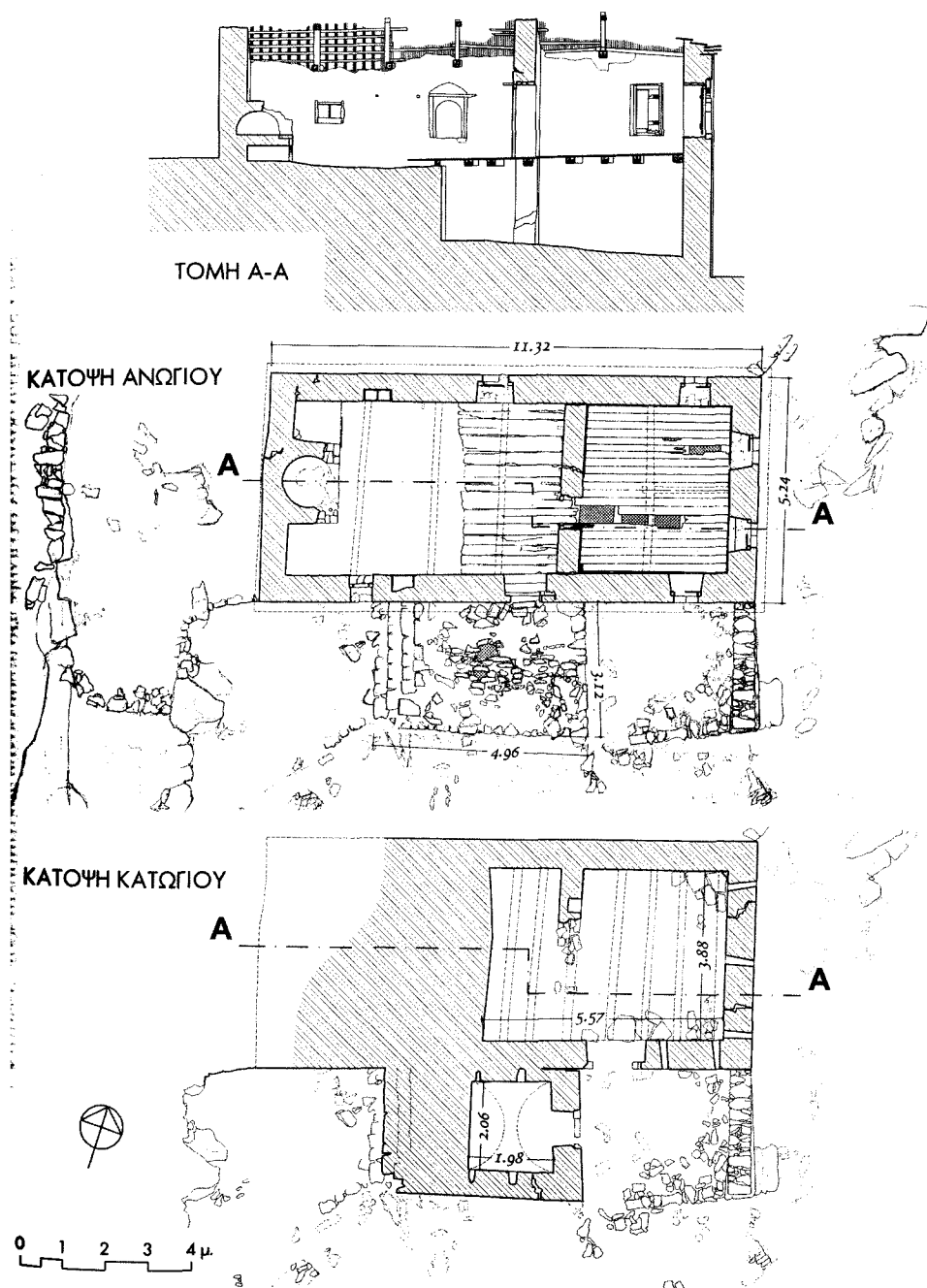
24. Κατόψεις και τομή προεπαναστατικού μακριναριού στην Ποταμιά (σπίτι 8).
