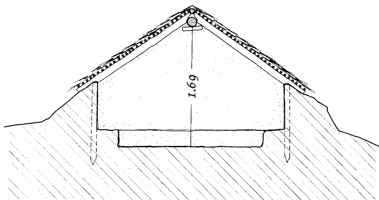
ΤΟΜΗ Α-Α
