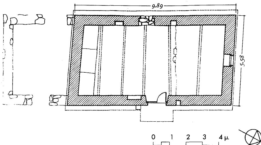
17. Κάτοψη καλύβιού στου Παιδεμένου (σπίτι 77α).
