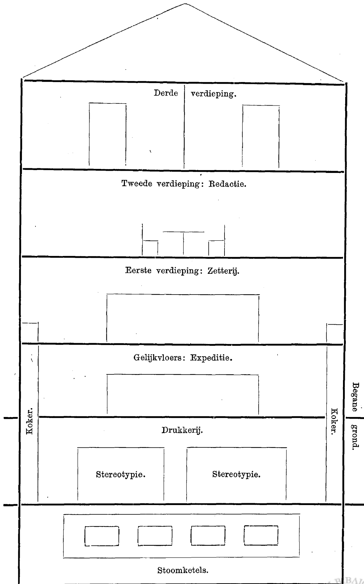
Doorsnede van het gebouw.
