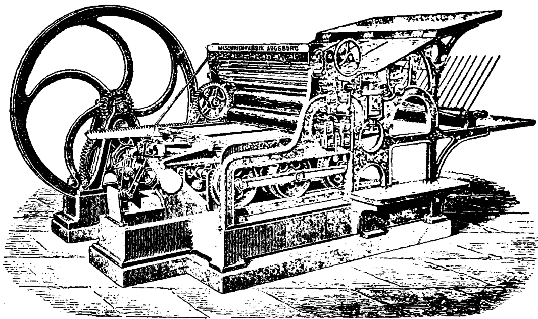
Gewone handsneijpers voor boekwerk en kleine nieuwsbladen met beperkte oplaat. Deze is voor één vorm ingericht en heeft slechts één drukcilinder, benevens een zelfwerkenden uitlegger. Zij levert per uur 1000 à 1500 afdrucken. (Fabr. Maschinenfabrik „Augsburg“ te Augsburg).
