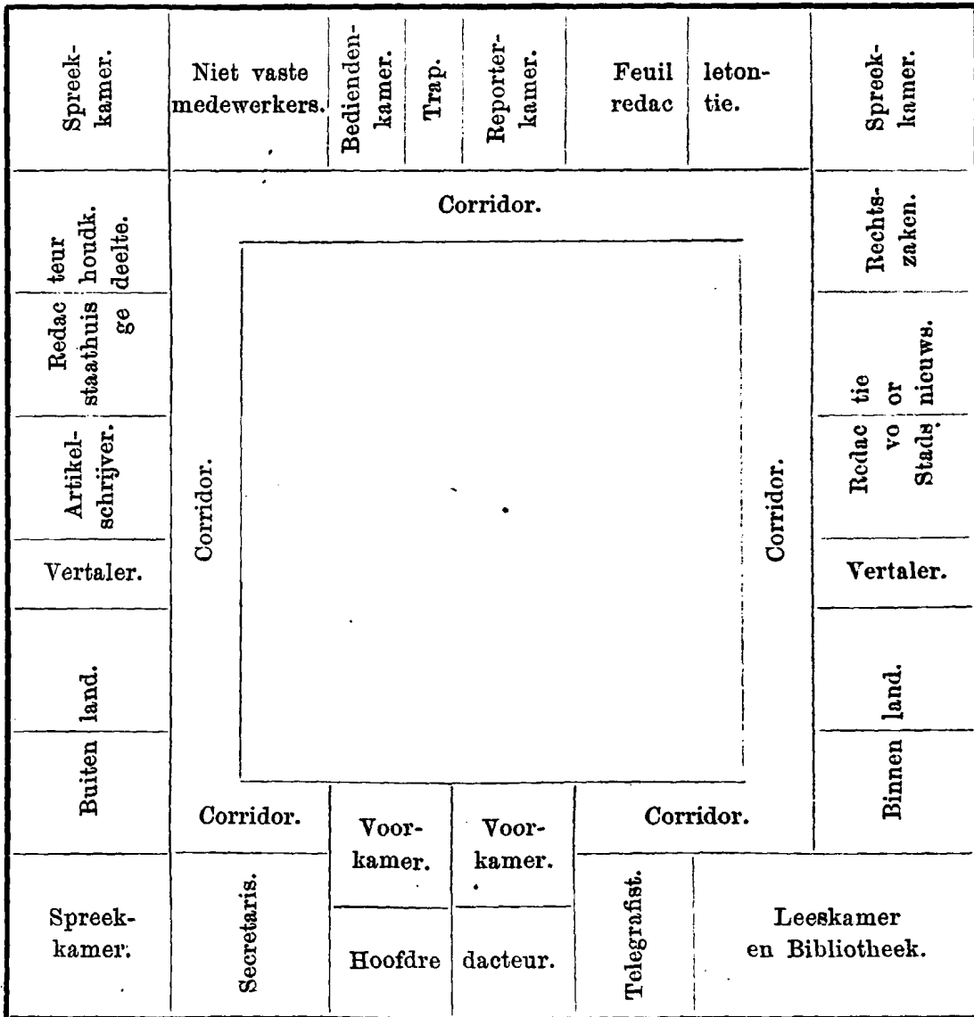
Plattegrond van de tweede verdieping.
