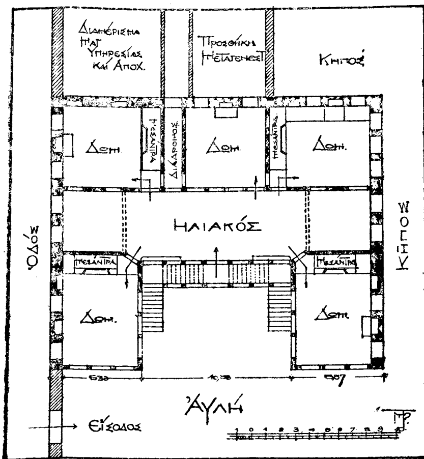
Εἰκ. 1. — Κάτοπις οἰκίας Μίσιου.
