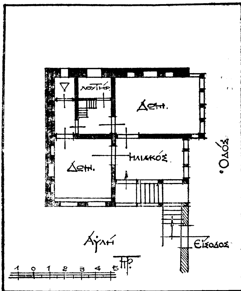
Εἰκ. 2. — Κάτοψις μικρᾶς οἰκίας.
