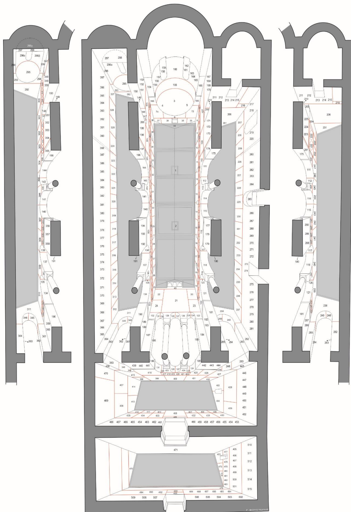
Καθολικά, Κοίμηση της Θεοτόκου, Προποικική άνοχη (σχ. Γ. Φουστέρη)
