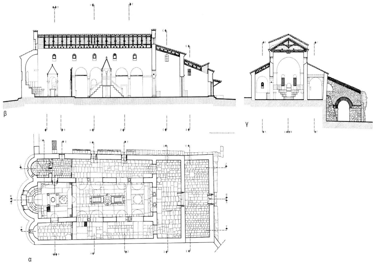
Καλαμπάκα, Κοίμηση της Θεοτόκου: α. κάτοψη, β. τομή κατά μήκος προς Ν και γ. τομή κατά πλάτος προς Α. (σχέδια Σ. Βογιατζή, βλ. V. Sythiakakis-Kritsimallis- S. Voyadjis, «Redating the Basilica of Dormition, Kalambaka, Thessaly», Jahrbuch der Österreichischen Byzantinistik 61 (2011) fig. 3, 4, 14).
