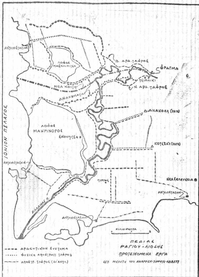
Σχεδιάγραμμα ἀλλαγῆς κοίτης Καλαμᾶ
