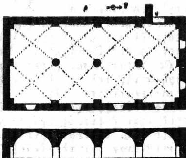
Εἰκ. 1.—Κάτοψη καὶ κατὰ μῆκος τομὴ τῆς ἀνατολικῆς δεξαμενῆς
