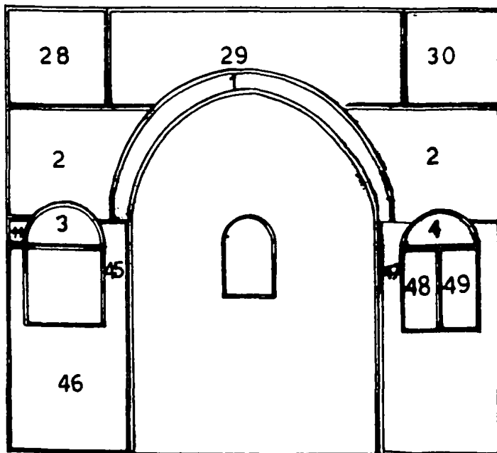
Ανατολικός Τοίχος
