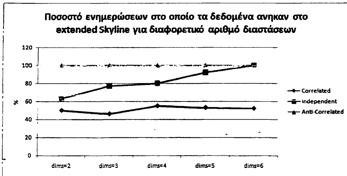
Σχήμα 6.14 Ποσοστό Ενημερώσεων στο οποίο τα Δεδομένα ανήκαν στο extended Skyline για Διαφορετικό Αριθμό Διαστάσεων.
