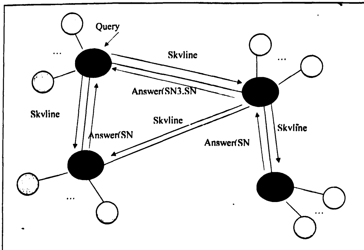
Σχήμα 3.2 Δρομολόγηση Skyline Ερωτήσεων
