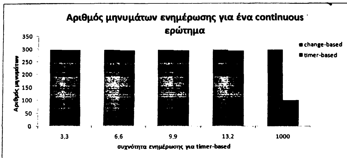
Σχήμα 6.18 Αριθμός Μηνυμάτων Ενημέρωσης για ένα Continuous Ερώτημα
