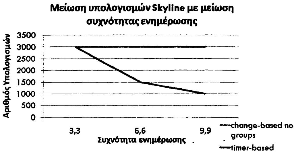
Σχήμα 6.19 Αριθμός Skyline Υπολογισμών
