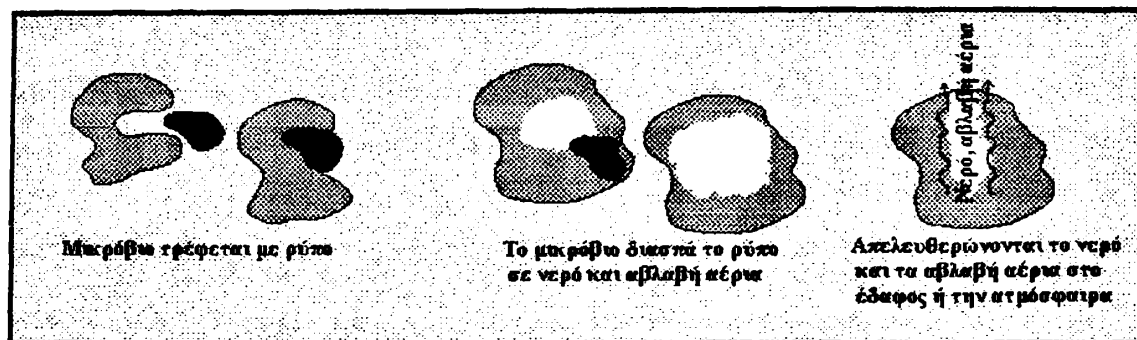
Σχήμα 1.8 Αναπαράσταση της βιοδιάσπασης φυτοφαρμάκων από μικροοργανισμούς
