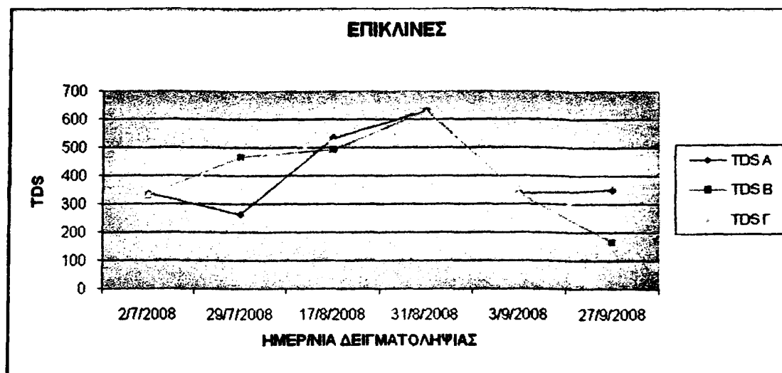
Γράφημα 6.18 Διακύμανση TDS νερού στο επικλινές τεμάχιο
