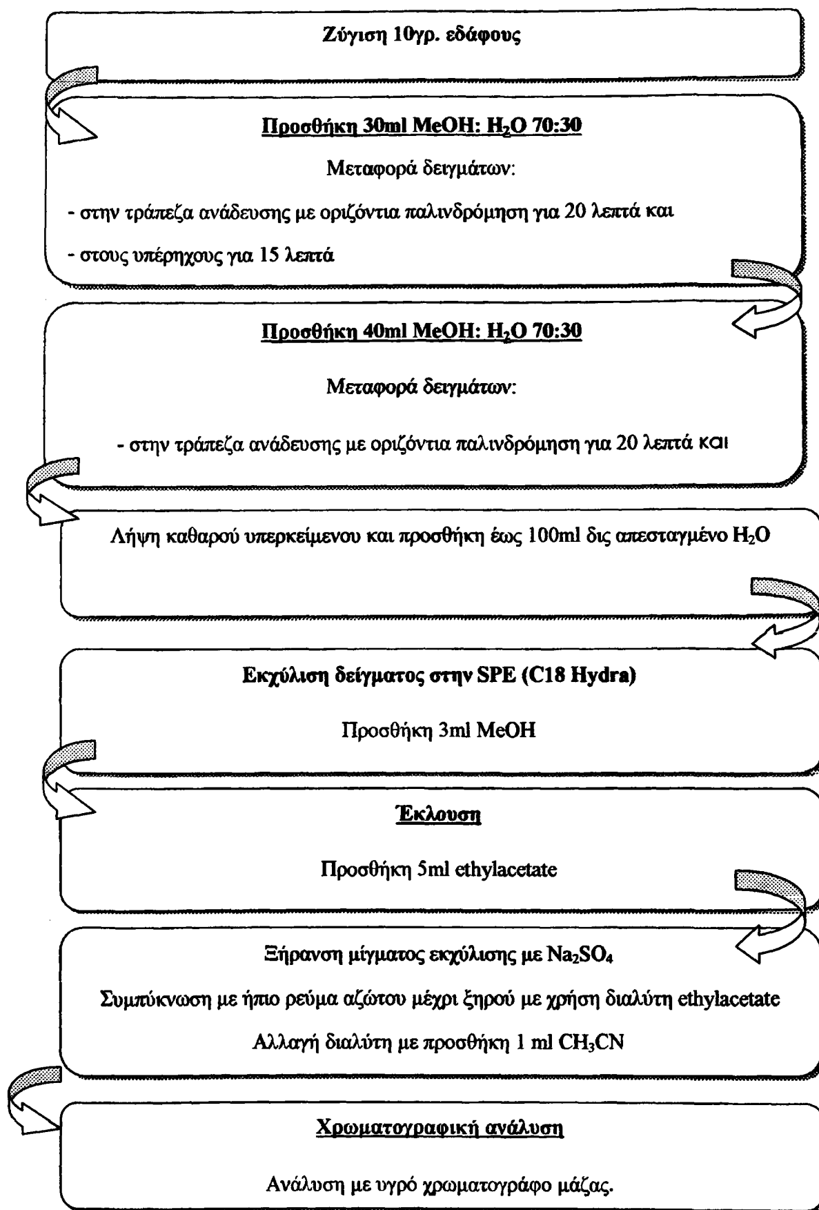
Σχήμα 7.4 Διάγραμμα πειραματικής πορείας ανάλυσης εδαφικών δειγμάτων
