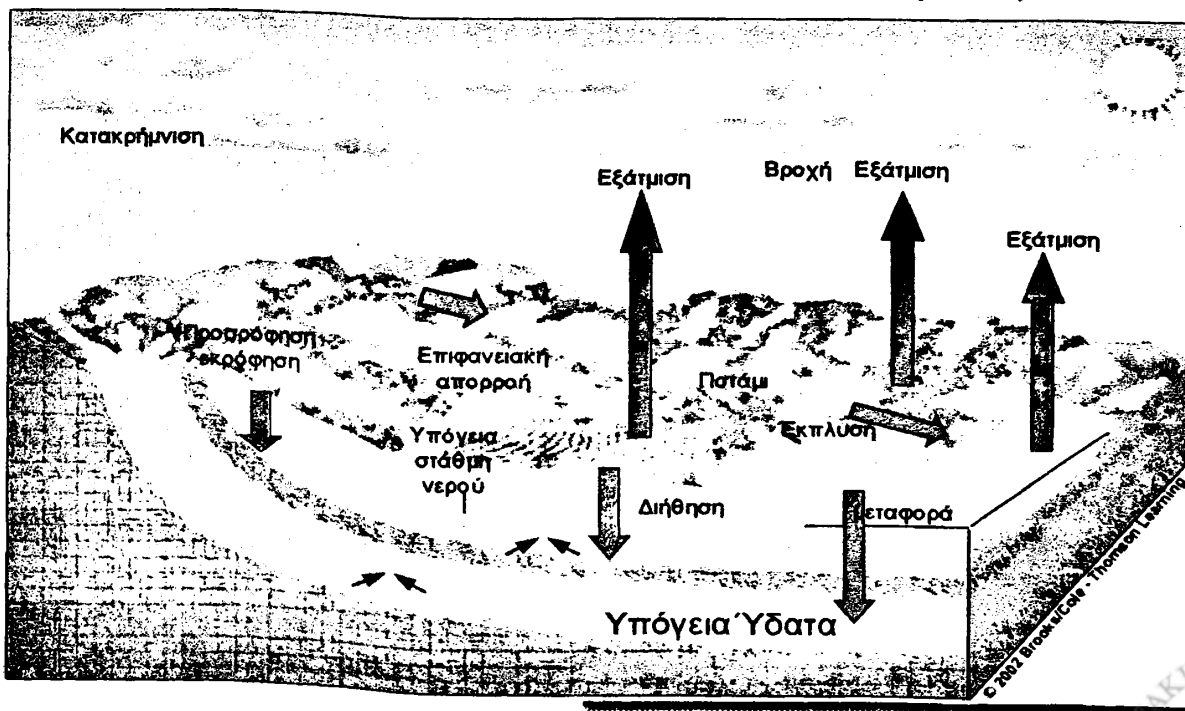
Εικόνα 1.5 Υδρολογικός κύκλος (προσαρμογή από τον Gray, 1994)
