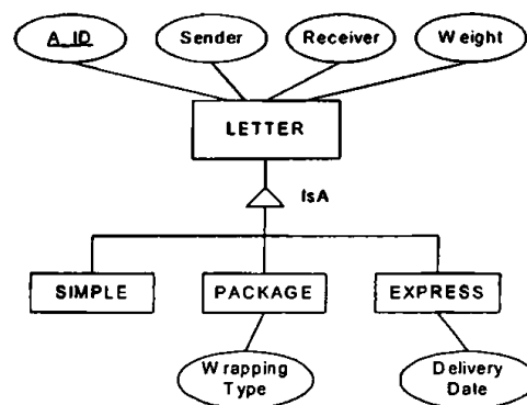
Σχήμα 4.39 Αναπαράσταση του παραδείγματος στο ER μοντέλο.
