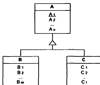
Σχήμα 4.40 Αναπαράσταση σε UML της γενικής περίπτωσης IsA.
