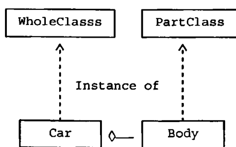
Σχήμα 2.3 Αναπαράσταση της προσέγγισης δύο μετακλάσεων [σχ. 16, [3]].
