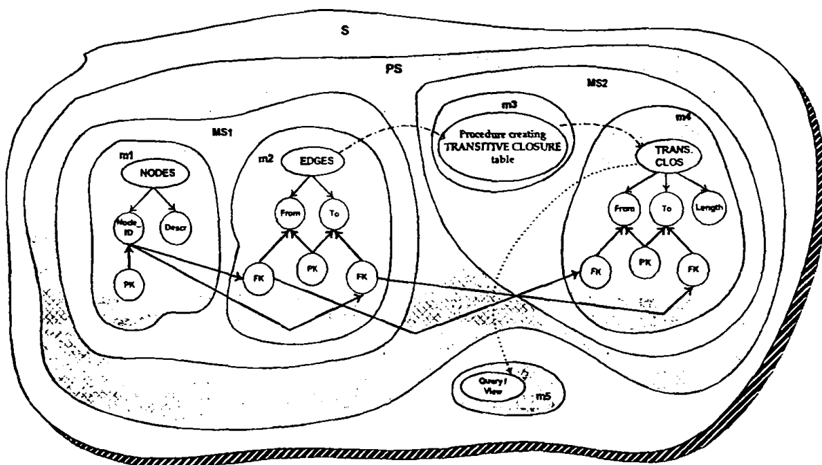
Σχήμα 5.21 Αναπαράσταση της σχεδιαστικής λύσης, όπου κατασκευάζεται πίνακας αναδρομικής κλειστότητας με την μέθοδο του κεφαλαίου 4 ενότητα 4.5.
