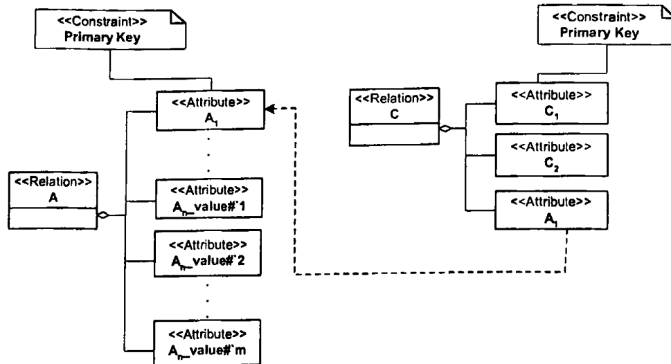
Σχήμα 4.58 Αναπαράσταση δομής σχήματος της γενικής περίπτωσης materialization με χρήση της δεύτερης σχεδιαστικής λύσης (ξεχωριστά πεδία για κάθε τιμή των μεταγνωρισμάτων).
