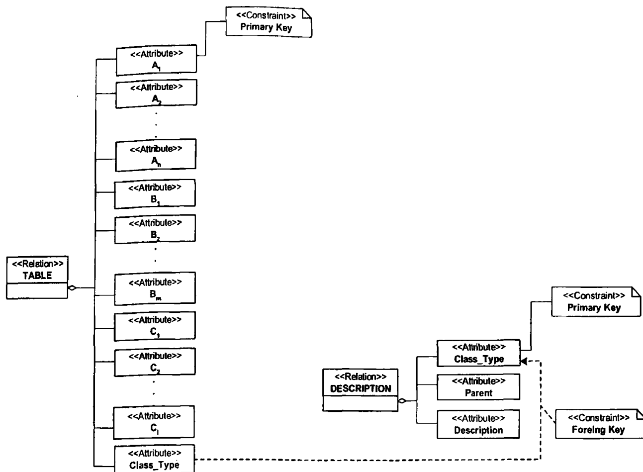
Σχήμα 4.41 Αναπαράσταση δομής σχήματος της γενικής περίπτωσης IsA εφαρμόζοντας την πρώτη σχεδιαστική λύση (ένας πίνακας να περιλαμβάνει τα γνωρίσματα όλων των κλάσεων).
