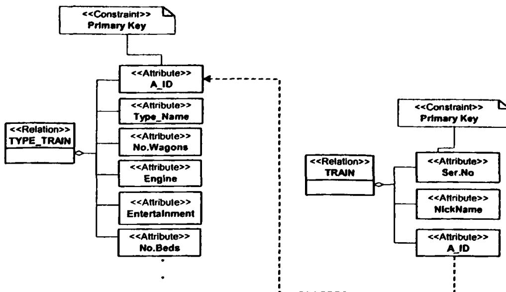
Σχήμα 4.54 Αναπαράσταση δομής του σχήματος της δεύτερης σχεδιαστικής λύσης (ξεχωριστά πεδία για κάθε τιμή των μεταγλωσσισμάτων).
