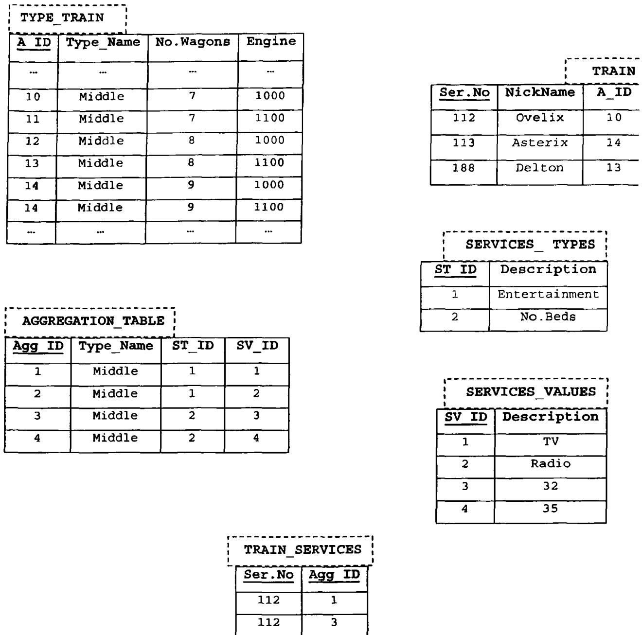
Σχήμα 4.53 Αναπαράσταση στιγμιότυπων των πινάκων της πρώτης σχεδιαστικής λύσης.
