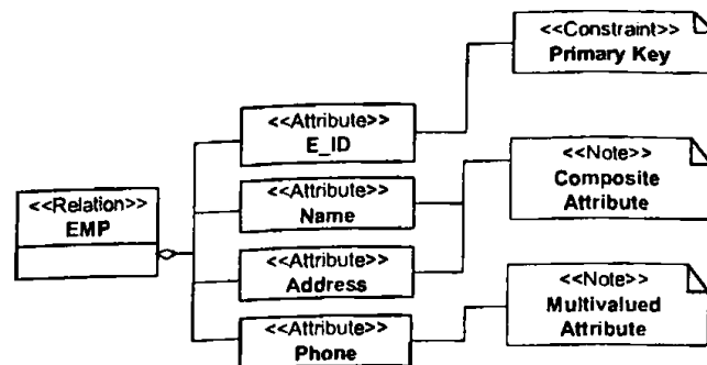
Σχήμα 4.8 Αναπαράσταση δομής του σχήματος της βάσης του παραδείγματος, στο οποίο παραβιάζεται η 1NF.
