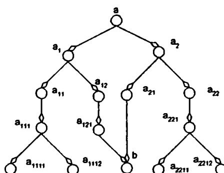
Σχήμα 4.37 Γράφος αναπαράστασης του aggregation.
