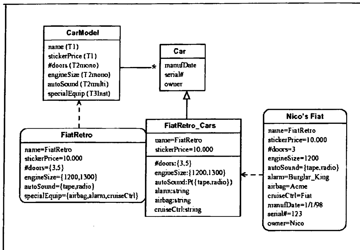
Σχήμα 2.8 Αναπαράσταση παραδείγματος materialization ως two-faceted κατασκευή [σχ.3, [2]].
