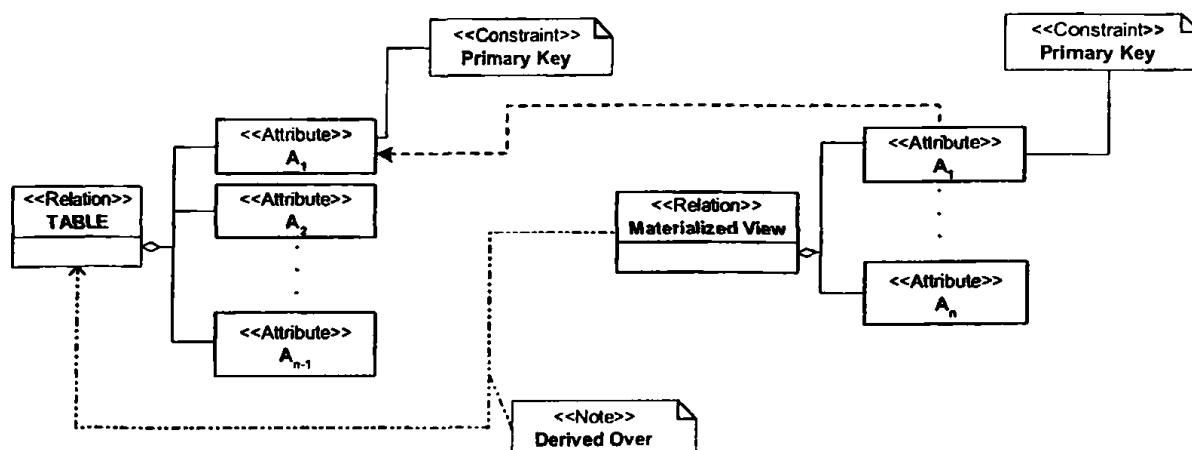
Σχήμα 4.30 Αναπαράσταση δομής γενικού σχήματος της δεύτερης σχεδιαστικής λύσης, με δημιουργία materialized view.
