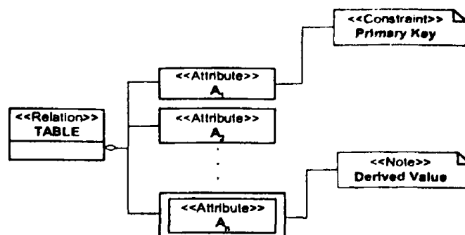
Σχήμα 4.28 Αναπαράσταση δομής γενικού σχήματος της πρώτης σχεδιαστικής λύσης, με εισαγωγή επιπλέον πεδίου, για το παραγόμενο γνώρισμα.
