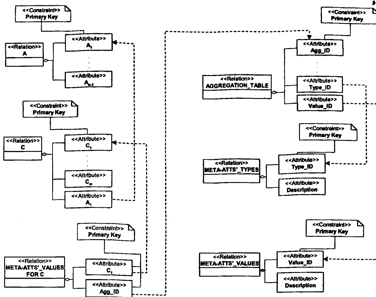
Σχήμα 4.57 Αναπαράσταση δομής σχήματος της γενικής περίπτωσης materialization με χρήση της πρώτης σχεδιαστικής λύσης (ξεχωριστοί πίνακες των μεταγνωρισμάτων της Abstract κλάσης και ένας συναθροιστικός βοηθητικός πίνακας).
