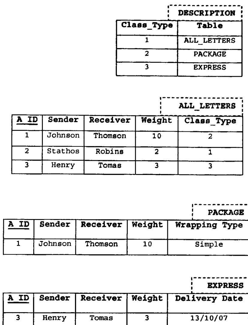
Σχήμα 4.50 Αναπαράσταση στιγμιότυπου του παραδείγματος με χρήση της πέμπτης σχεδιαστικής μεθόδου.
