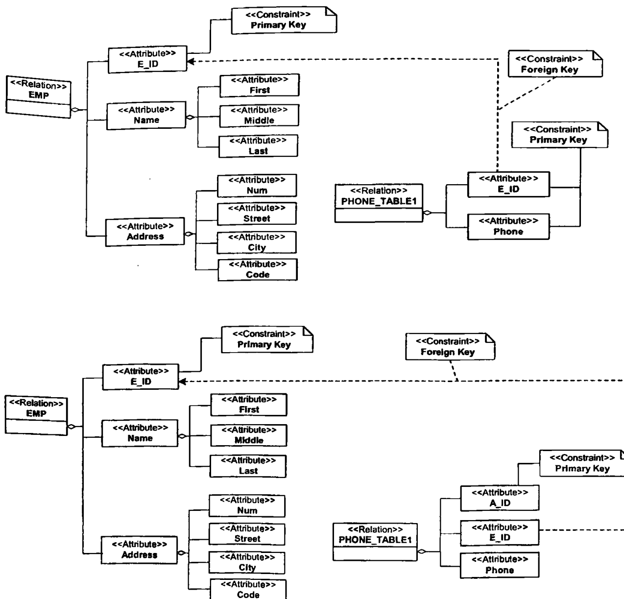
Σχήμα 4.9 Δύο εναλλακτικές αναπαραστάσεις της δομής του σχήματος της βάσης του παραδείγματος όπως προκύπτει μετά την κανονικοποίηση σε 1NF.
