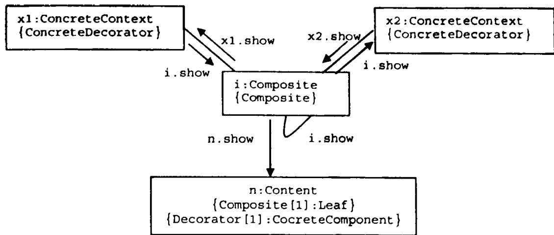
Σχήμα 2.7 Αναπαράσταση σύνθεσης των κλάσεων Component και Content με την μέθοδο tagged pattern annotation [σχ. 6, [4]].
