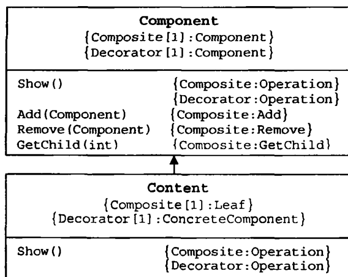
Σχήμα 2.6 Αναπαράσταση δομής των κλάσεων Component και Content με την μέθοδο tagged pattern annotation [σχ. 5, [4]].
