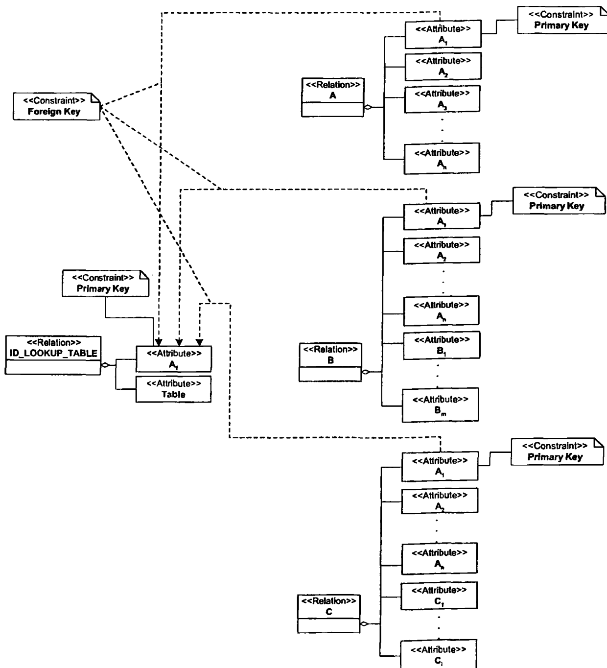
Σχήμα 4.47 Αναπαράσταση δομής σχήματος της γενικής περίπτωσης IsA εφαρμόζοντας την τέταρτη σχεδιαστική λύση (ξεχωριστοί πίνακες για κάθε κλάση με περιορισμούς αναφορικής ακεραιότητας σε έναν βοηθητικό πίνακα).
