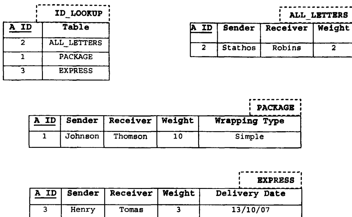
Σχήμα 4.48 Αναπαράσταση στιγμιότυπου του παραδείγματος με χρήση της τέταρτης σχεδιαστικής μεθόδου.
