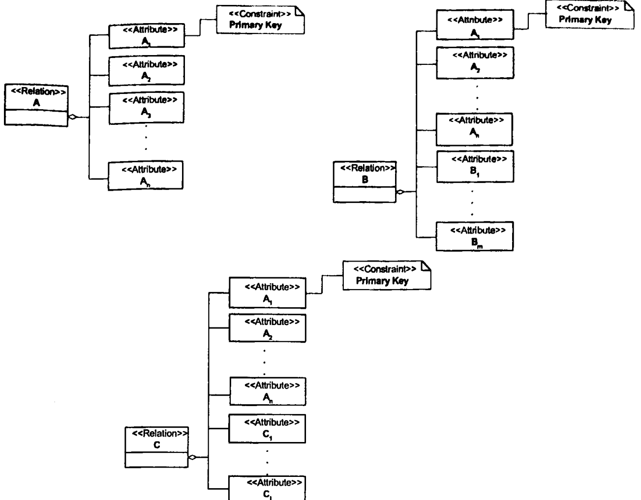
Σχήμα 4.45 Αναπαράσταση δομής σχήματος της γενικής περίπτωσης IsA εφαρμόζοντας την τρίτη σχεδιαστική λύση (δημιουργία ξεχωριστών πινάκων για κάθε κλάση χωρίς περιορισμούς αναφορικής ακεραιότητας).
