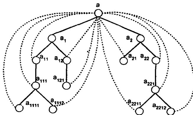
Σχήμα 4.35 Γράφος αναπαράστασης της αναδρομικής κλειστότητας.
