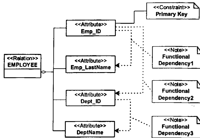
Σχήμα 4.17 Αναπαράσταση του σχήματος του πίνακα του παραδείγματος που δεν βρίσκεται σε 3NF.
