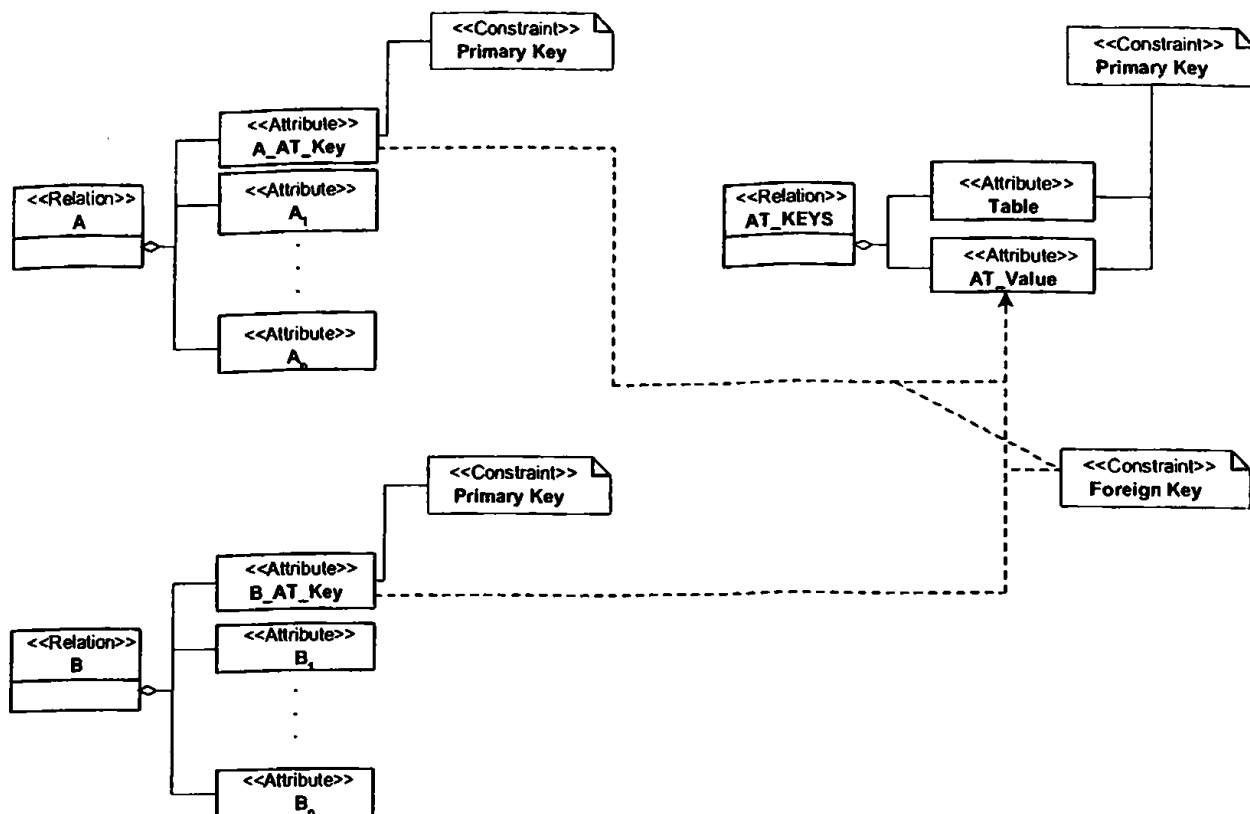
Σχήμα 4.4 Αναπαράσταση δομής με την δημιουργία συμβουλευτικού πίνακα καταχώρησης της μέγιστης τιμής του τεχνητού κλειδιού κάθε πίνακα.
