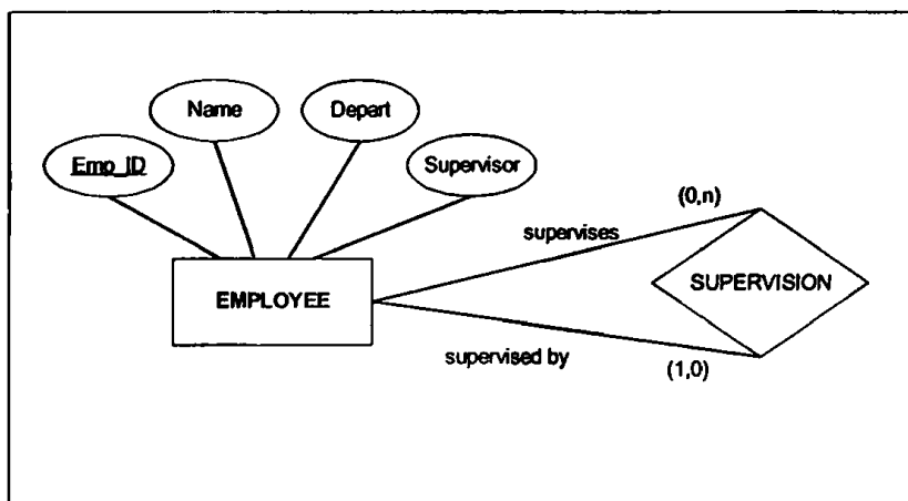
Σχήμα 4.33 Αναπαράσταση του παραδείγματος στο ER μοντέλο.
