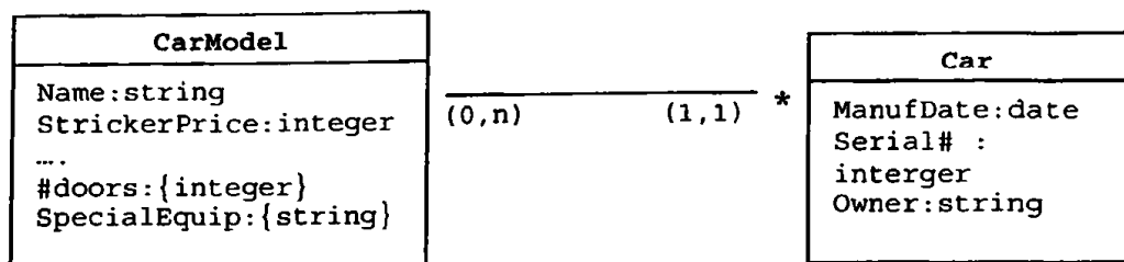
Σχήμα 2.1 Αναπαράσταση παραδείγματος materialization [σχ.2, [3]].
