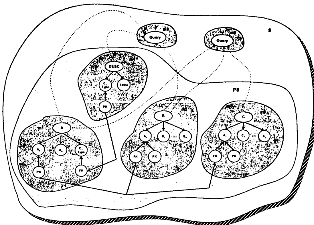
Σχήμα 5.25 Αναπαράσταση της 2 ης σχεδιαστικής λύσης, όπου κατασκευάζεται ένας πίνακας για την υπερκλάση, A, βοηθητικός για την αναζήτηση, και ένας πίνακας για κάθε υποκλάση.
