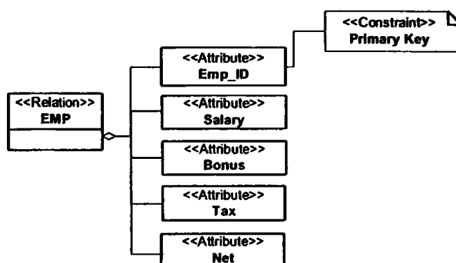
Σχήμα 4.22 Αναπαράσταση του σχήματος του παραδείγματος με χρήση του προτύπου flat design.
