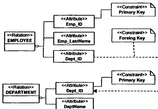
Σχήμα 4.18 Αναπαράσταση του σχήματος του πίνακα του παραδείγματος μετά την κανονικοποίηση σε 3NF.
