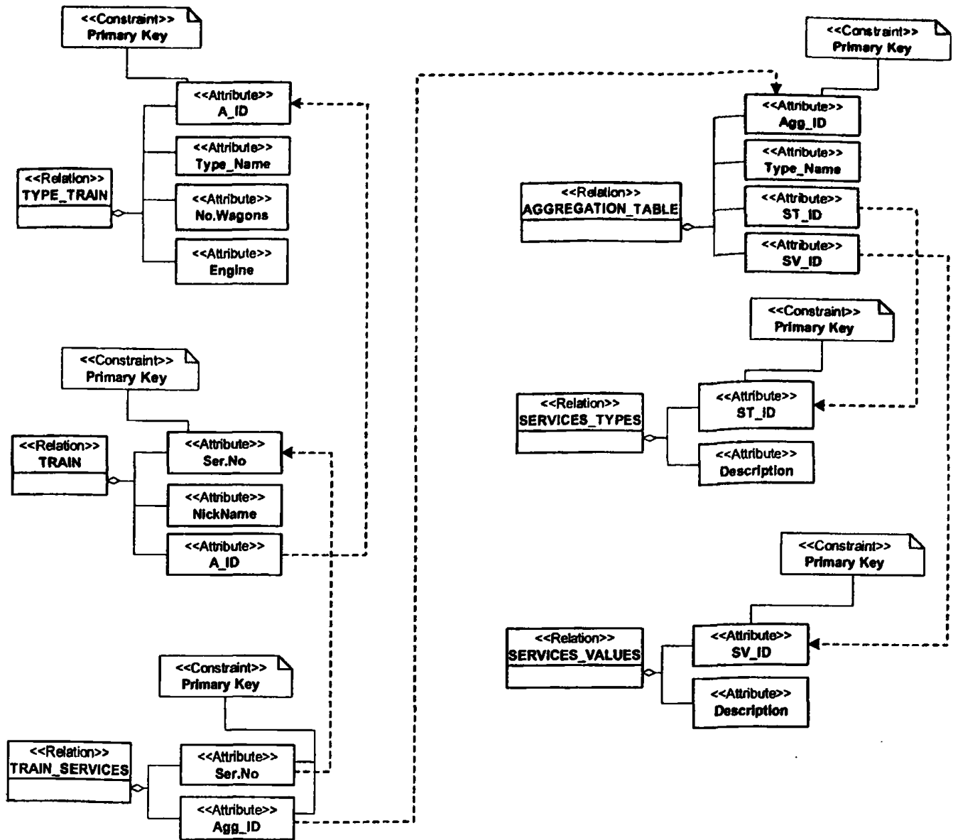
Σχήμα 4.52 Αναπαράσταση δομής σχήματος της πρώτης σχεδιαστικής λύσης (ξεχωριστοί πίνακες των μεταγγνωρισμάτων της Abstract κλάσης και ένας συναθροιστικός βοηθητικός πίνακας).
