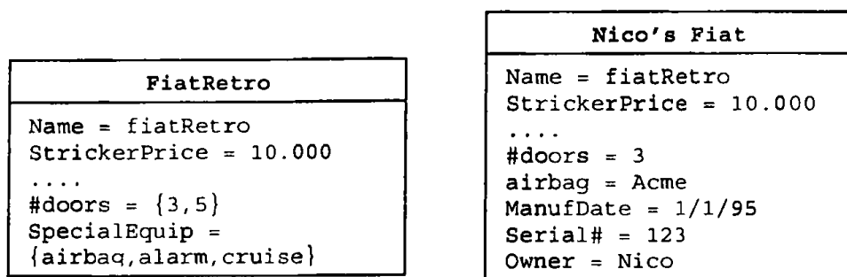
Σχήμα 2.2 Αναπαράσταση στιγμιότυπου του παραδείγματος materialization [σχ3, [3]].
