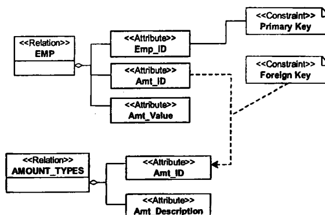
Σχήμα 4.22 Αναπαράσταση του σχήματος του παραδείγματος με χρήση του προτύπου flat design.
