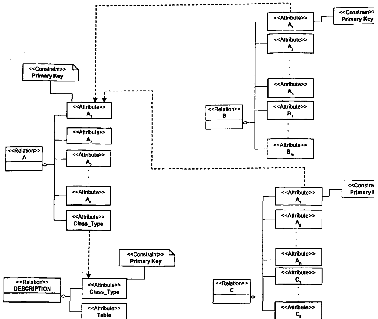
Σχήμα 4.49 Αναπαράσταση δομής σχήματος της γενικής περίπτωσης IsA εφαρμόζοντας την πέμπτη σχεδιαστική λύση (δημιουργία ξεχωριστών πινάκων για κάθε υποκλάση με περιορισμούς αναφορικής ακεραιότητας στον πίνακα της υπερκλάσης, και ενός βοηθητικού πίνακα).
