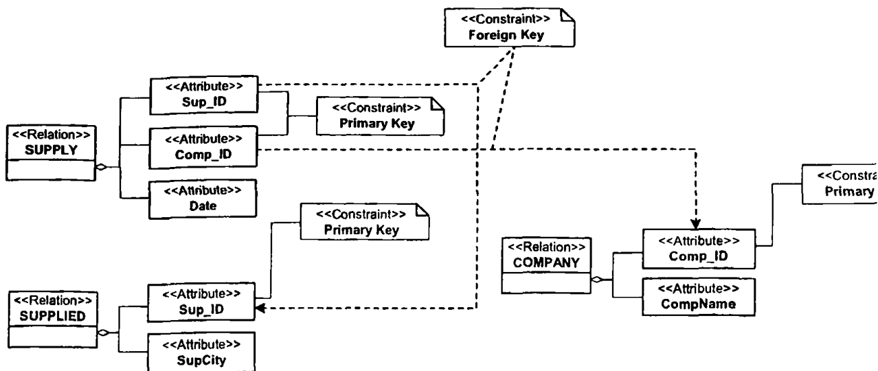
Σχήμα 4.14 Αναπαράσταση του σχήματος των πινάκων που προκύπτουν μετά την κανονικοποίηση σε 2NF του αρχικού πίνακα του παραδείγματος.
