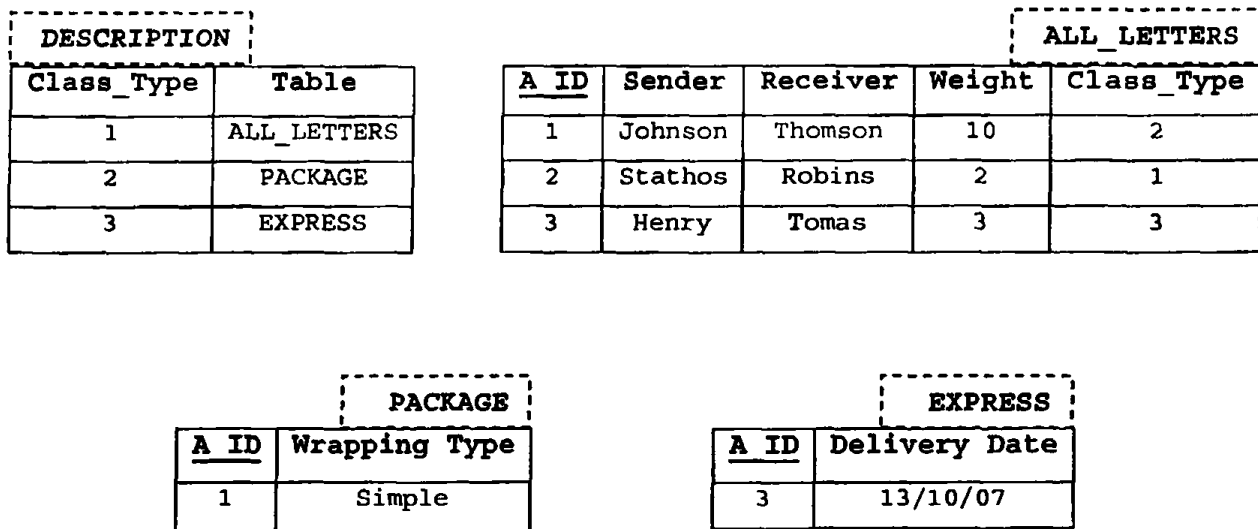
Σχήμα 4.44 Αναπαράσταση στιγμιότυπου του παραδείγματος με χρήση της δεύτερης σχεδιαστικής μεθόδου.
