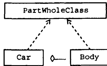
Σχήμα 2.4 Αναπαράσταση της προσέγγισης μιας μετακλάσης [σχ. 16, [3]].
