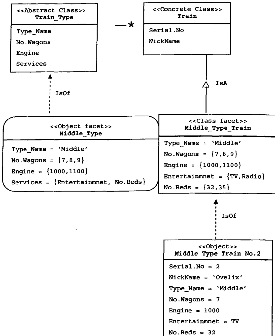
Σχήμα 4.51 Αναπαράσταση του σχήματος του παραδείγματος σε UML, με βάση την προσέγγιση του [2].
