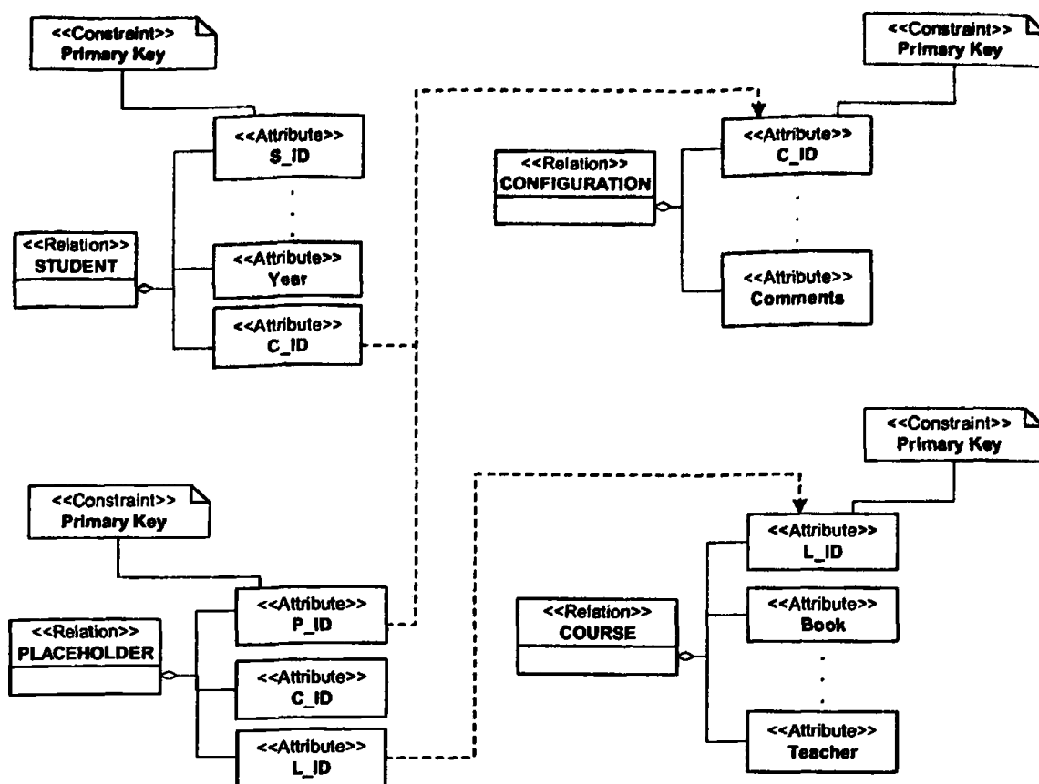
Σχήμα 4.59 Αναπαράσταση δομής σχήματος του προτύπου Configuration για το παράδειγμα της γραμματείας ενός τμήματος πανεπιστημίου.
