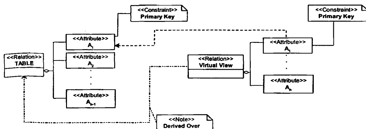
Σχήμα 4.31 Αναπαράσταση δομής γενικού σχήματος της τρίτης σχεδιαστικής λύσης, με δημιουργία virtual view.
