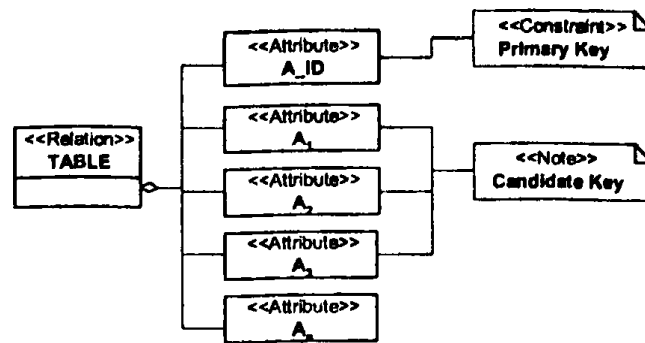
Σχήμα 4.1 Αναπαράσταση δομής σχήματος ενός τυχαίου πίνακα μιας βάσης δεδομένων, ο οποίος περιλαμβάνει ως υποψήφια κλειδιά είτε ένα string, είτε συνδυασμό γνωρισμάτων.
