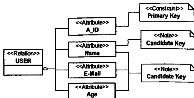
Σχήμα 4.2 Αναπαράσταση δομής σχήματος της βάσης του παραδείγματος με την εισαγωγή τεχνητού κλειδιού.
