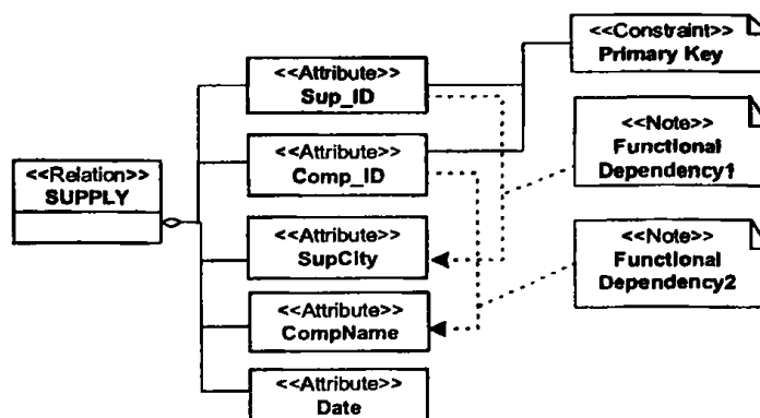
Σχήμα 4.13 Αναπαράσταση του σχήματος του πίνακα του παραδείγματος που δεν βρίσκεται σε 2NF.
