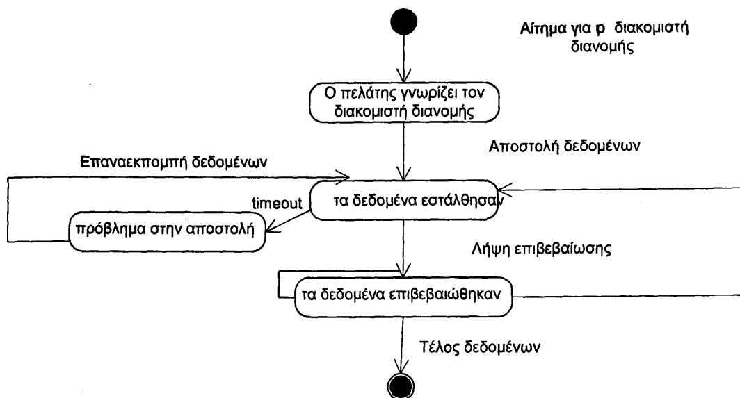
Σχήμα 4.2: Διάγραμμα ροής δεδομένων
