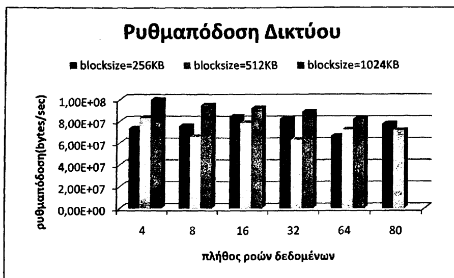
Σχήμα 6.1: Υπολογίζεται η ρυθμαπόδοση του δικτύου σε συνάρτηση με το πλήθος των ταυτόχρονων ροών δεδομένων που υπάρχουν στο σύστημα. Επίσης, εμφανίζονται για κάθε πλήθος ροών δεδομένων μια ράβδο για κάθε διαφορετική τιμή μπλοκ που επιλέχθηκε.
