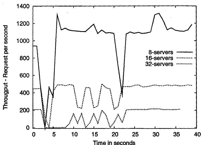
Σχήμα 6.6: Αποτυχία Επικεφαλής Διακομιστή
