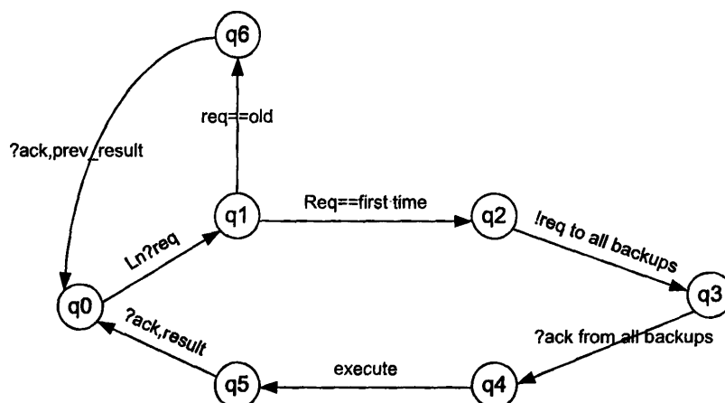
Σχήμα 4.5: Διάγραμμα Καταστάσεων του Επικεφαλής Διακομιστή
