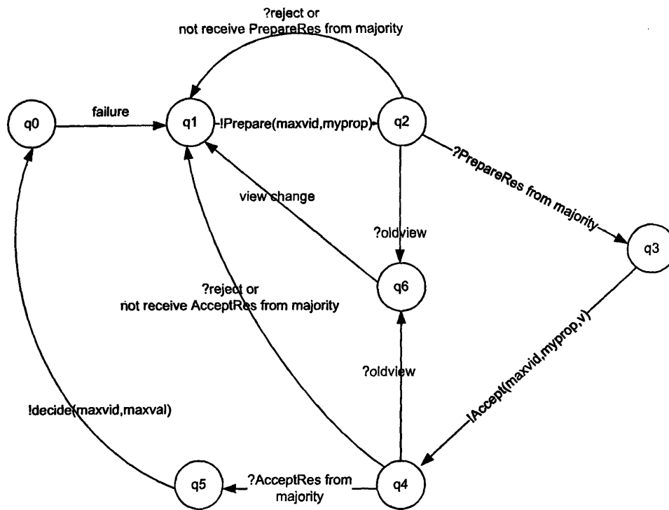
Σχήμα 5.1: Διάγραμμα Καταστάσεων του Αποστολέα μηνυμάτων του Paxos
