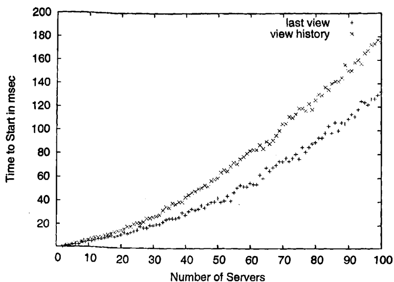
Σχήμα 6.4: Χρόνος Εκκίνησης Διακομιστή
