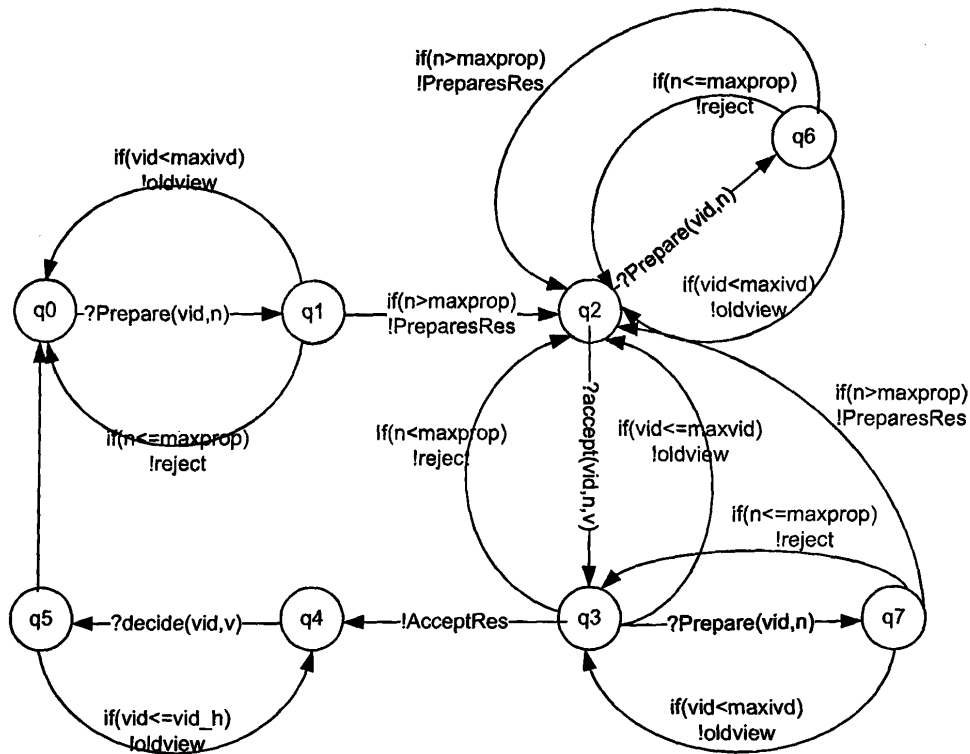
Σχήμα 5.2: Διάγραμμα Καταστάσεων του Αποδέκτη μηνυμάτων του Paxos
