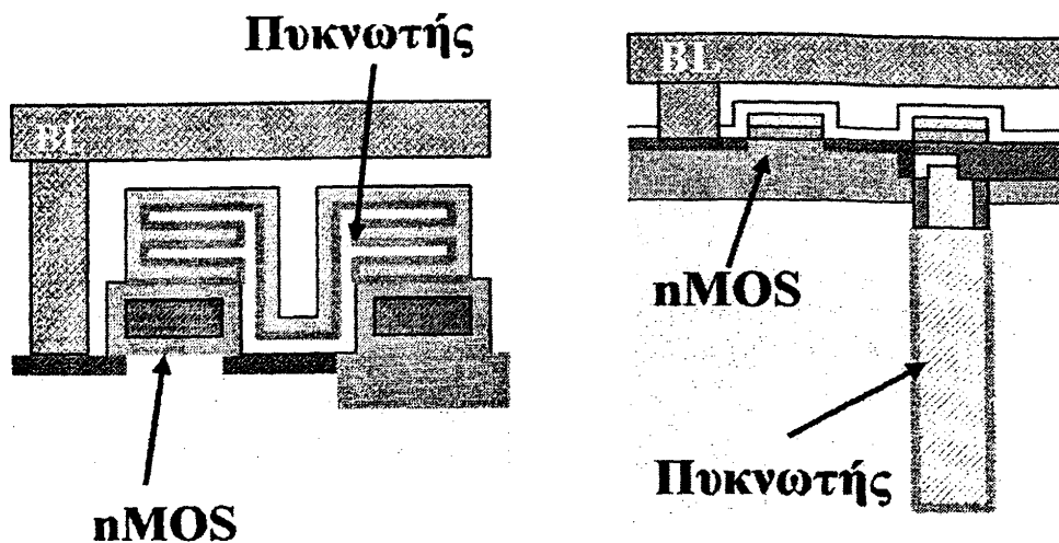
Σχήμα 2.2 Οι Δύο Τύποι Πυκνωτών
