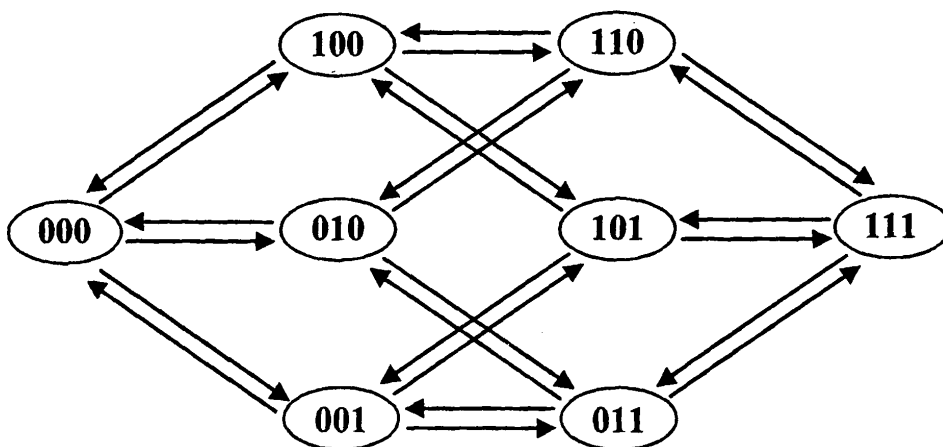
Σχήμα 3.1 Ο Γράφος του Euler για 3 - bit
