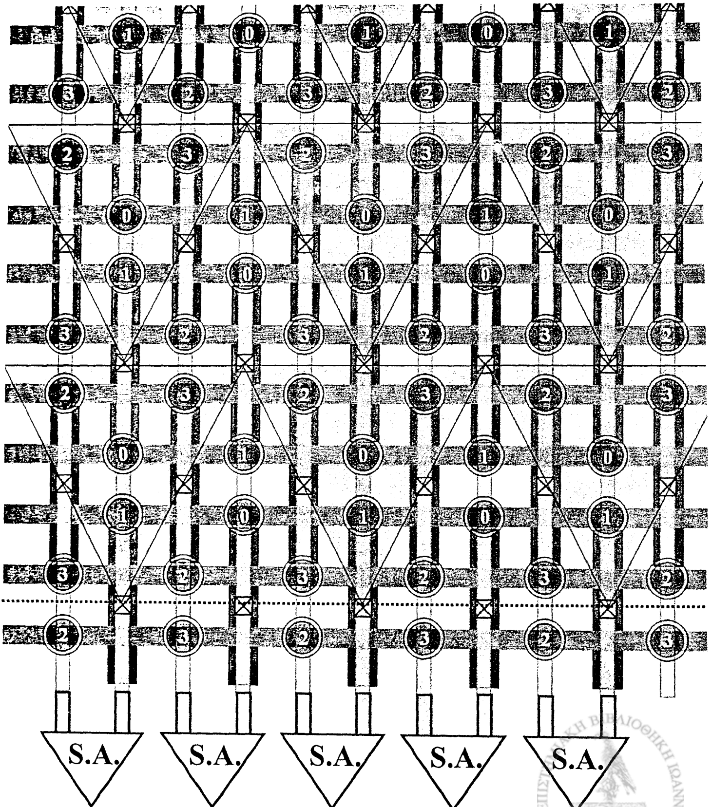
Σχήμα 5.2 Η Τύπου - Α Γειτονιά
