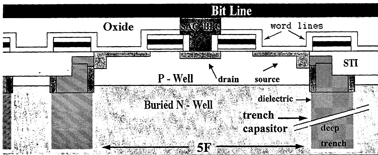
Σχήμα 5.1 Κάθετη Τομή Μνήμης με Πυκνωτή Τύπου Πηγαδιού
