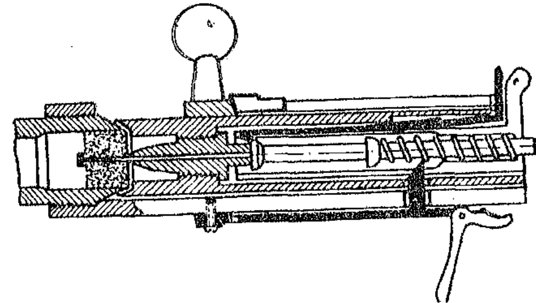
Σχῆμα 5. Τυφέκιον Γράισε. Ὀπισθογεμῆς μετὰ κλείστρου, σφύρας καὶ ἐπικρουστήρος.
