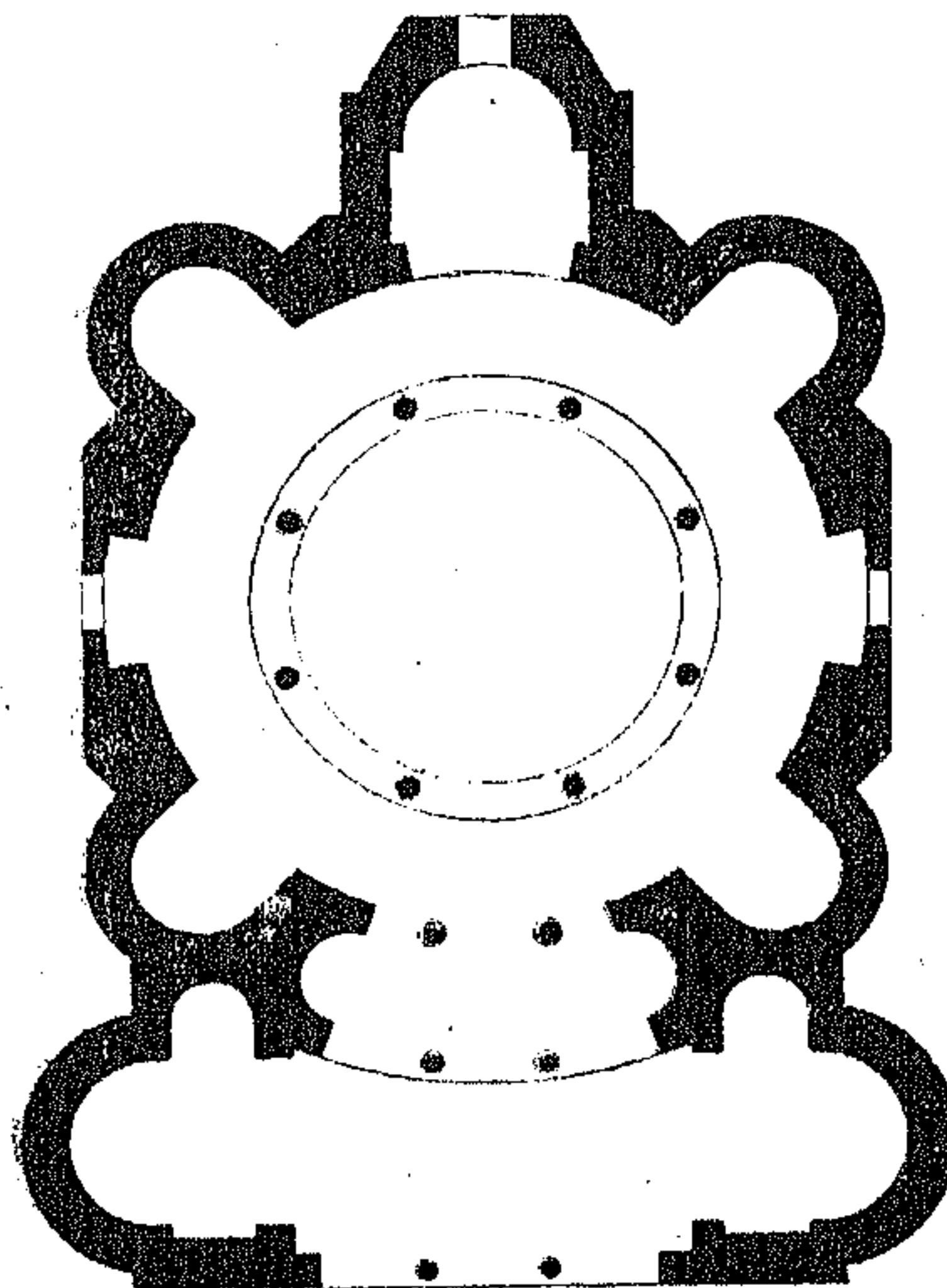
Κάτοψις τοῦ κυκλωτεροῦ ναοῦ.
