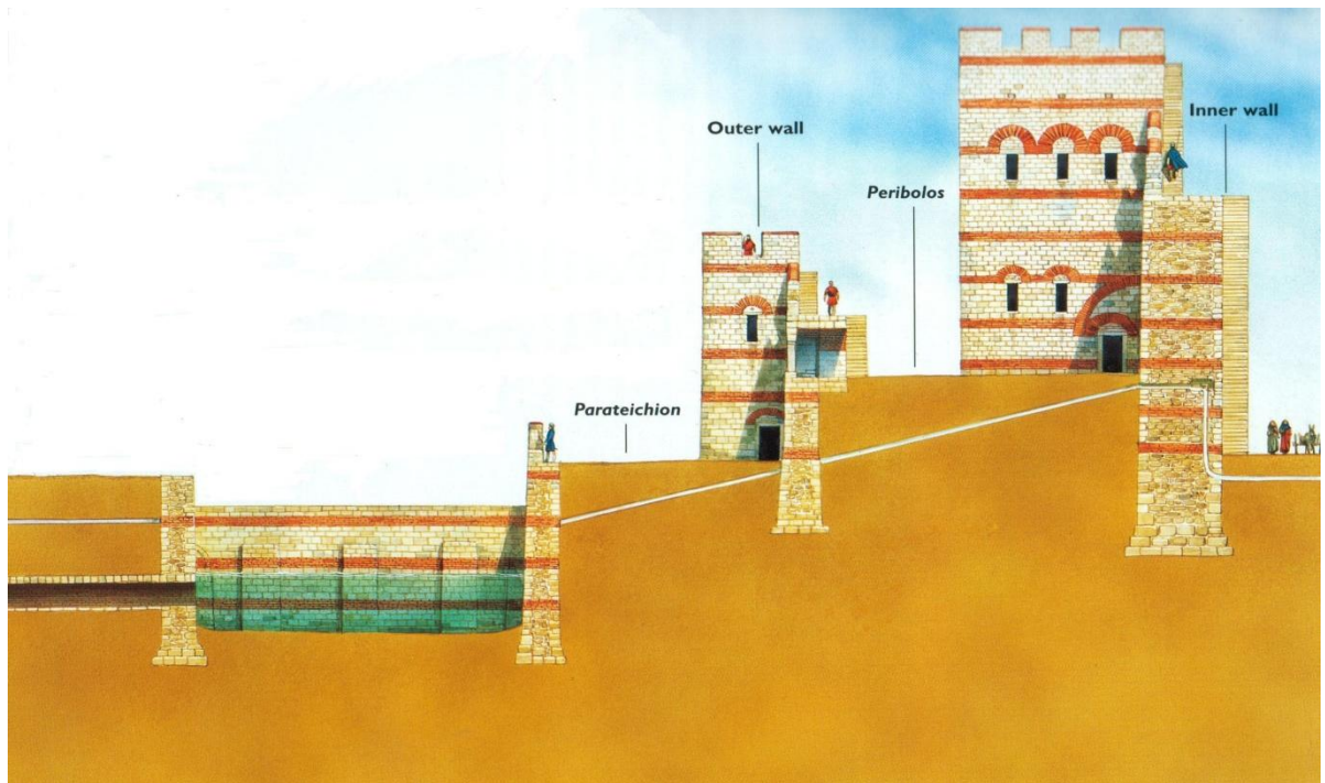
(Σκαρίφημα του τριπλού τείχους της Κωνσταντινούπολης και της τάφρου, S. Turnbull, Walls of Constantinople , Osprey Publishing, 2004).
