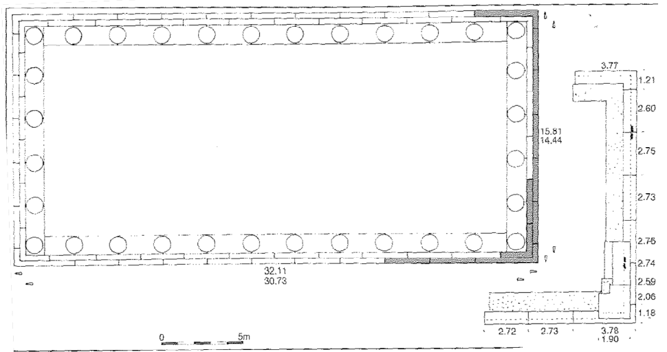
Εικ. 8: Κάτοψη του ελληνιστικού ναού των Φερών (E. Østby, Υπέρεια Α 1990)
