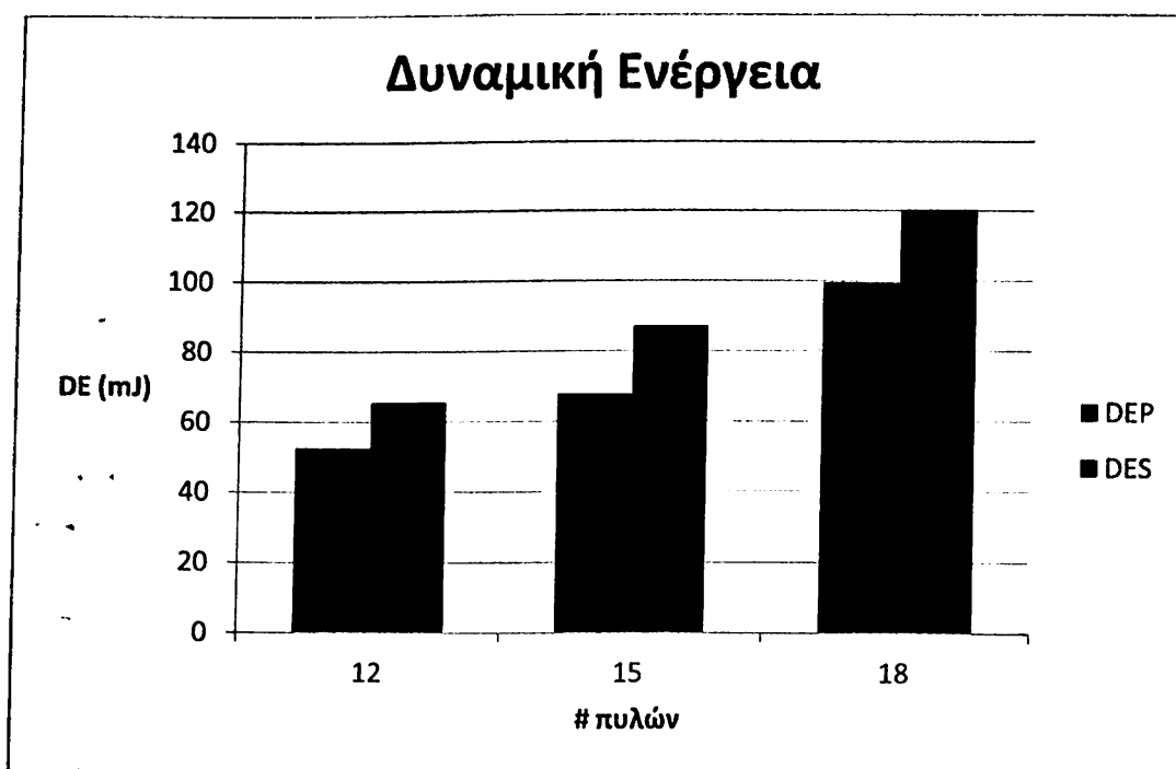
Σχήμα 6.28. Δυναμική Κατανάλωση για την Τριγωνική Κατανομή σε Σχέση με το Μέγιστο Αριθμό Πυλών
