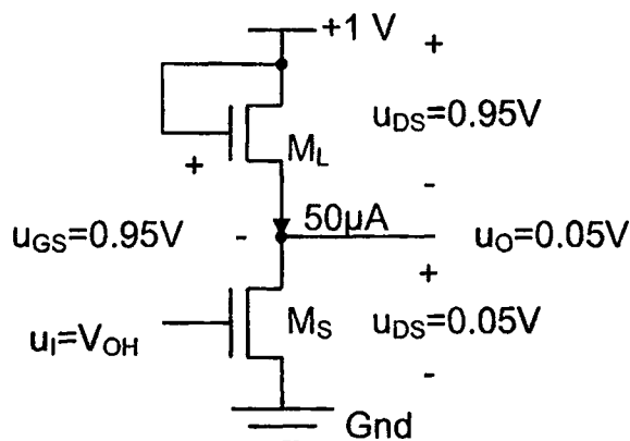
Σχήμα 5.3. Παράδειγμα Κυκλώματος με Φόρτο σε Συνδεσμολογία Διόδου
