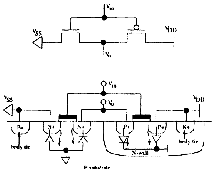
Σχήμα 2.3. Το Πλήρες Μοντέλο του CMOS Αναστροφέα
