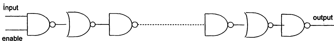
Σχήμα 6.15. Το κύκλωμα που Χρησιμοποιήθηκε στις Προσομοιώσεις σε Επίπεδο-Πύλης
