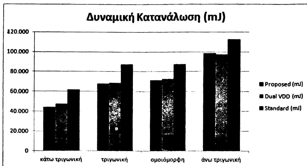
Σχήμα 6.21. Δυναμική Κατανάλωση για Διοδικό Τρανζίστορ με HV_i
