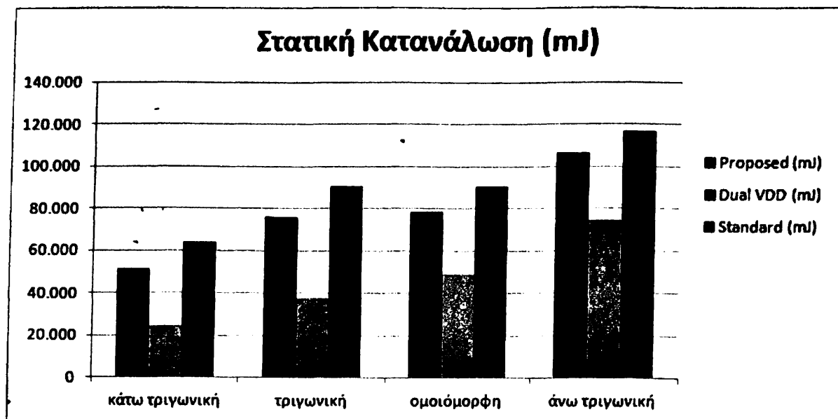
Σχήμα 6.22. Στατική Κατανάλωση για Διοδικό Τρανζίστορ με HV_i
