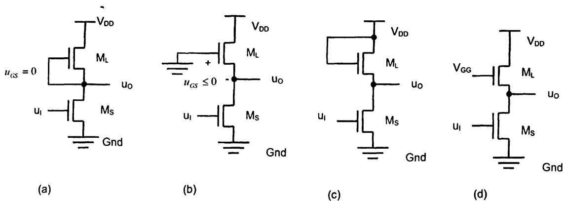
Σχήμα 5.2. (a) Αναστροφέας NMOS με την Πύλη του Στοιχείου Φόρτου Συνδεδεμένη με την Πηγή του (b) Αναστροφέας NMOS με Γειωμένη την Πύλη του Στοιχείου Φόρτου (c) Αναστροφέας με Τρανζίστορ σε Συνδεσμολογία Διόδου (d) Αναστροφέας με Γραμμικό Φόρτο
