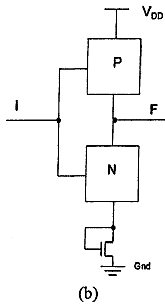
6.6. (a) Απλή Πύλη CMOS (b) Πύλη CMOS με την 7η Συνδεσμολογία
