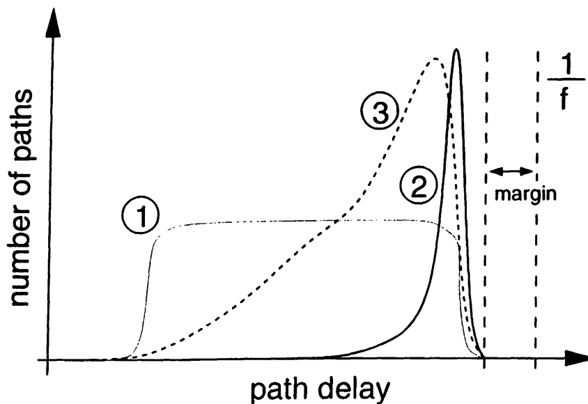
Σχήμα 3.3. Τρία Παραδείγματα Κατανομών της Καθυστερήσης Διάδοσης Σήματος Διαδρομής
