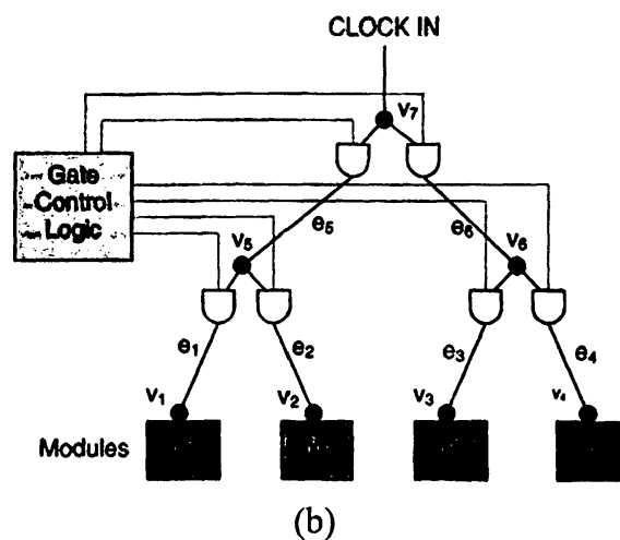
Σχήμα 3.13. (α) Μοντέλο ενός Δέντρου με Απενεργοποιημένο κατά Τμήματα Ρολόι (b) Τοπολογία ενός Δέντρου με Απενεργοποιημένο κατά Τμήματα Ρολόι [16]
