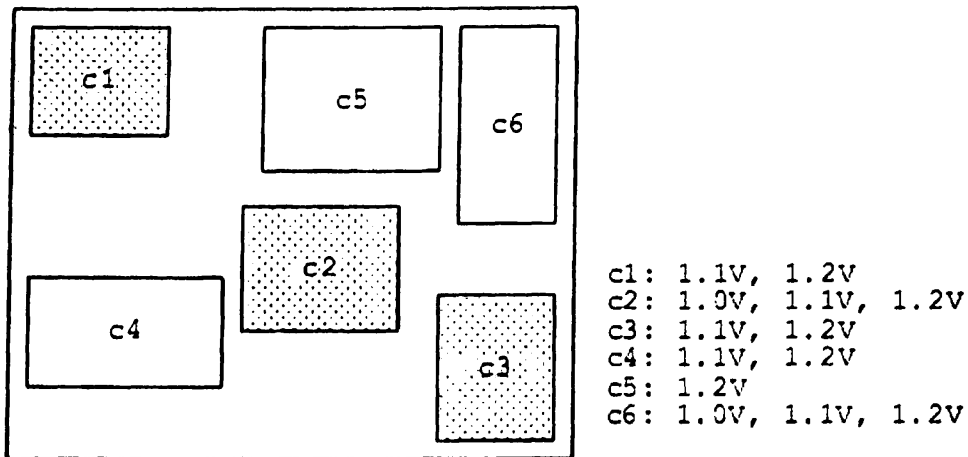
Σχήμα 3.10. Παράδειγμα SoC με τη Δημιουργία Τμημάτων Τάσης [13]
