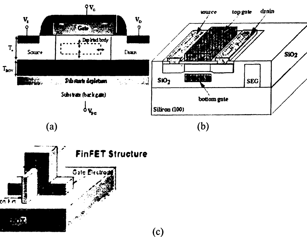
Σχήμα 4.4. (a) Τρανζίστορ Τεχνολογίας SOI (b) Τρανζίστορ SOI Διπλής Πύλης (c) FinFET Τρανζίστορ [20]
