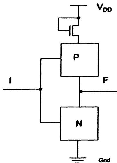
Σχήμα 6.16. Προτεινόμενη Τοπολογία που Χρησιμοποιήθηκε στις Προσομοιώσεις της Παρούσας Ενότητας
