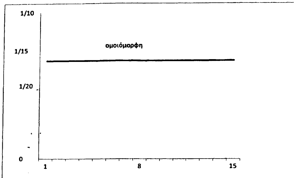
Σχήμα 6.18. Ομοιόμορφη Κατανομή
