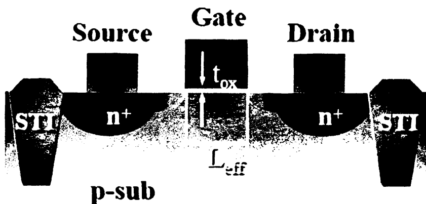
Σχήμα 2.4. Το ρεύμα στην Περιοχή Υποκατωφλίου ή Ρεύμα Ασθενούς Αναστροφής Ρέει στην Περιοχή κάτω από την Πύλη
