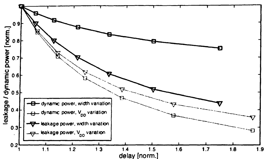
Σχήμα 3.4. Δυναμική και Στατική Κατανάλωση ενός Αναστροφέα με Χωρητικό Φορτίο 10 fF σε Συνάρτηση με την Καθυστερήση της Πύλης
