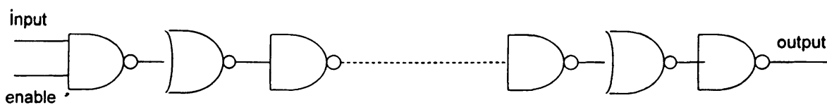
Σχήμα 6.9. Το κύκλωμα που Χρησιμοποιήσαμε στις Προσομοιώσεις σε Επίπεδο-Πύλης
