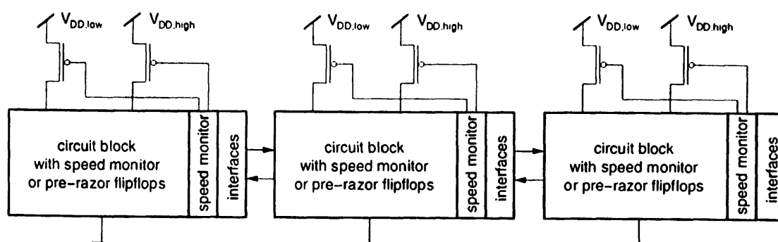
Σχήμα 3.7. Η Ιδέα των Δύο Διακοπών για Χαμηλή Κατανάλωση και Υψηλή Απόδοση Παραμέτρων [9]
