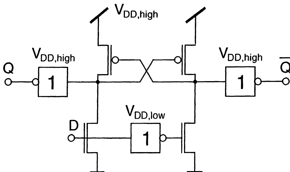
Σχήμα 3.5. Συμβατικό Ασύγχρονο Κύκλωμα Ανάκτησης Τάσης με Μέτρια Καθυστέρηση Διάδοσης Σήματος
