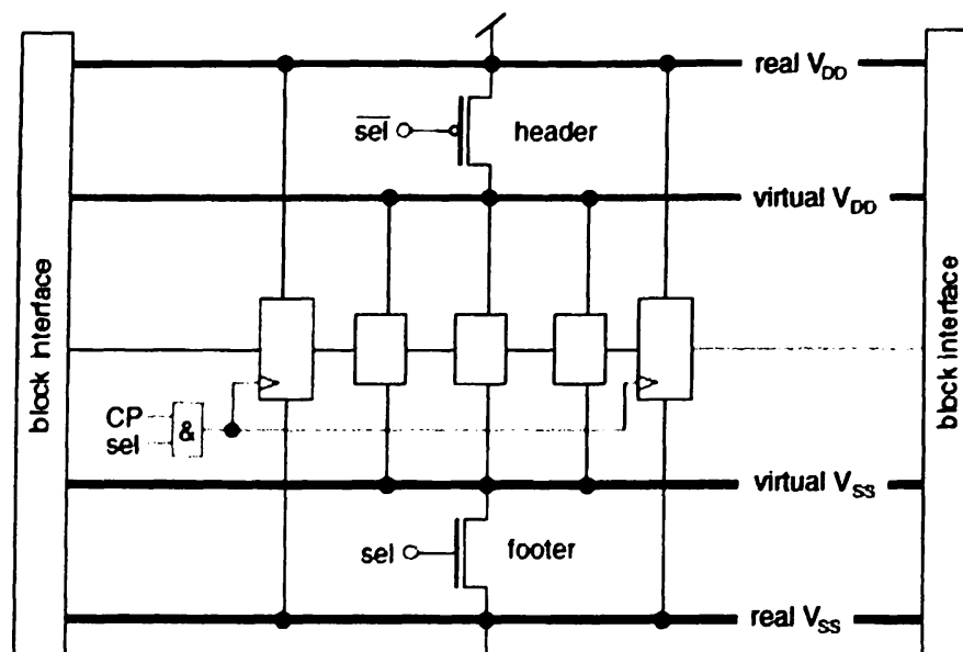
Σχήμα 4.2. Η Αρχή Λειτουργίας της Τεχνικής Απομόνωσης Ισχύος [18]
