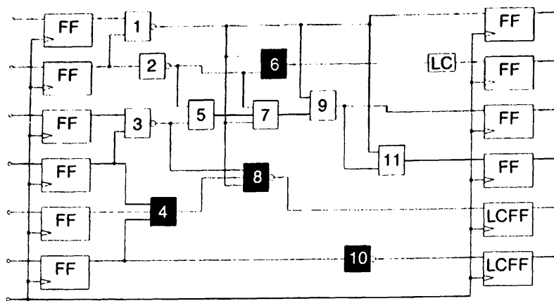
Σχήμα 3.1. Αρχή Λειτουργίας της Τεχνικής Πολλαπλών V_{DD} σε Επίπεδο Πύλης
