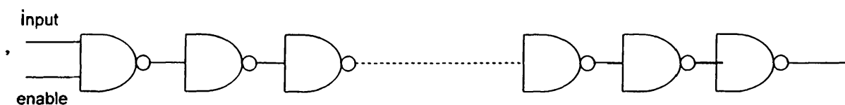
Σχήμα 6.11. Το Κύκλωμα που Χρησιμοποιήσαμε στις Προσομοιώσεις σε Επίπεδο-Πύλης
