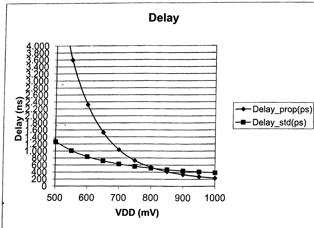
Σχήμα 6.13. Κλιμάκωση Τάσης για Προτεινόμενη και Standard Τεχνική
