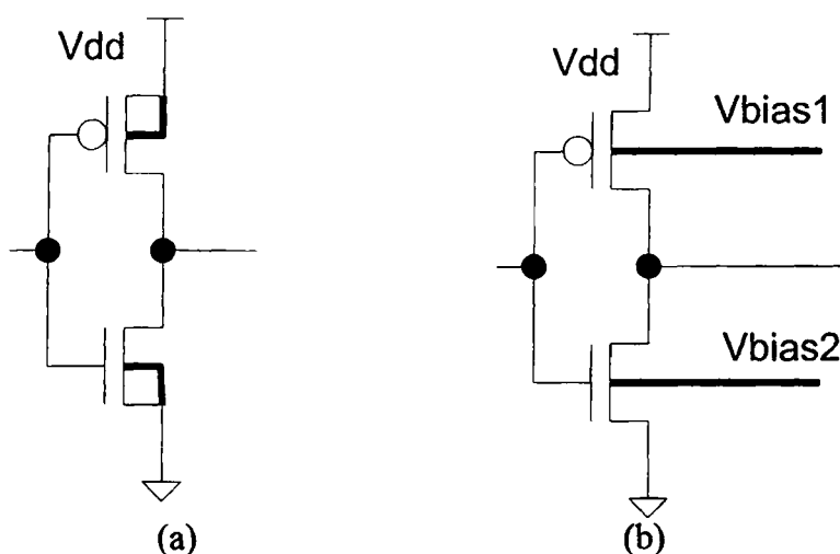
Σχήμα 4.3. (a) Γενική Σχεδίαση: Το Υπόστρωμα Συνδέεται στην Τροφοδοσία ή στη Γη. (b) Μεταβλητή Τάση Πόλωσης Υποστρώματος για να Μεταβάλλει την Τάση Κατωφλίου.
