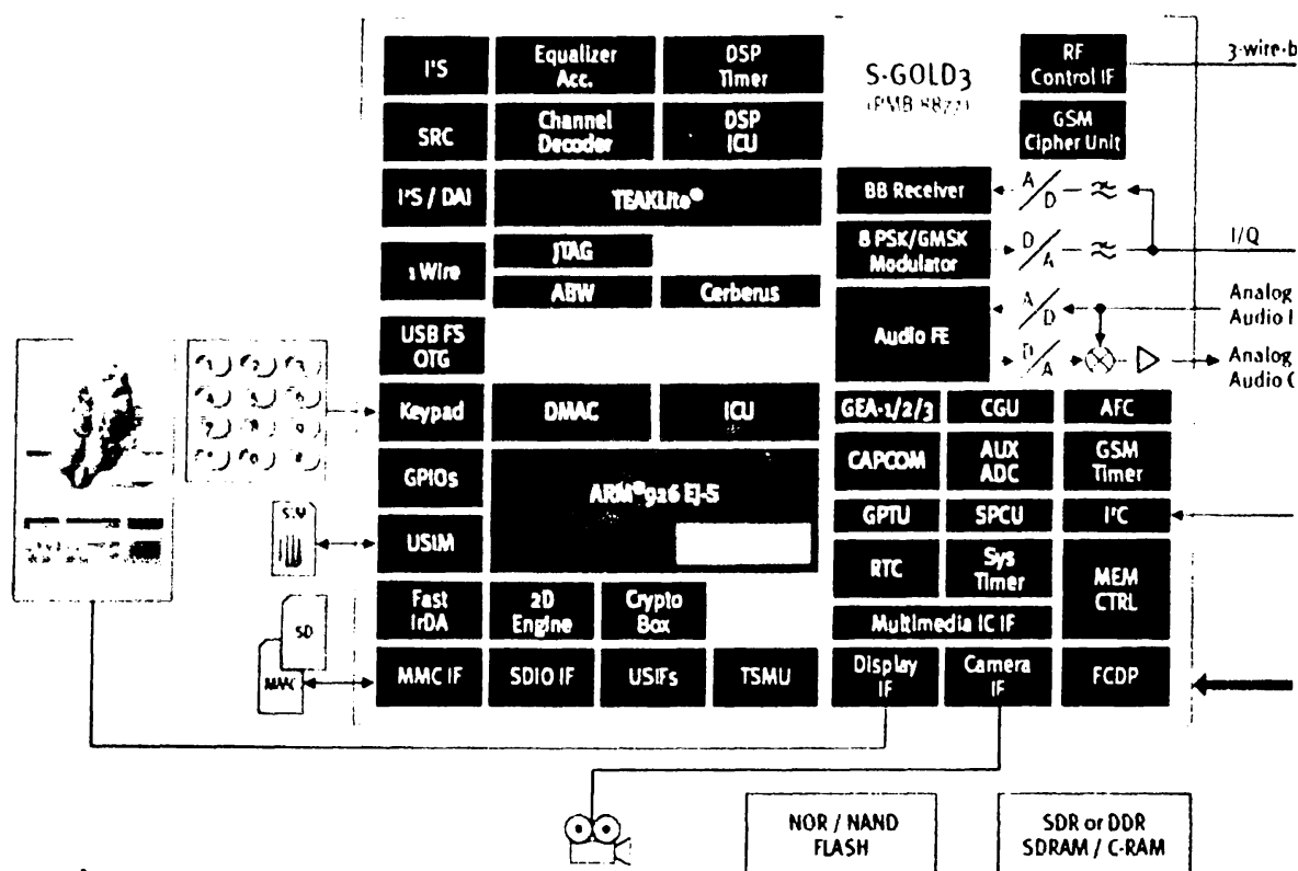
Σχήμα 4.1. Ο Επεξεργαστής Βασικής Ζώνης SGOLD3™ από τη Infineon Technologies
