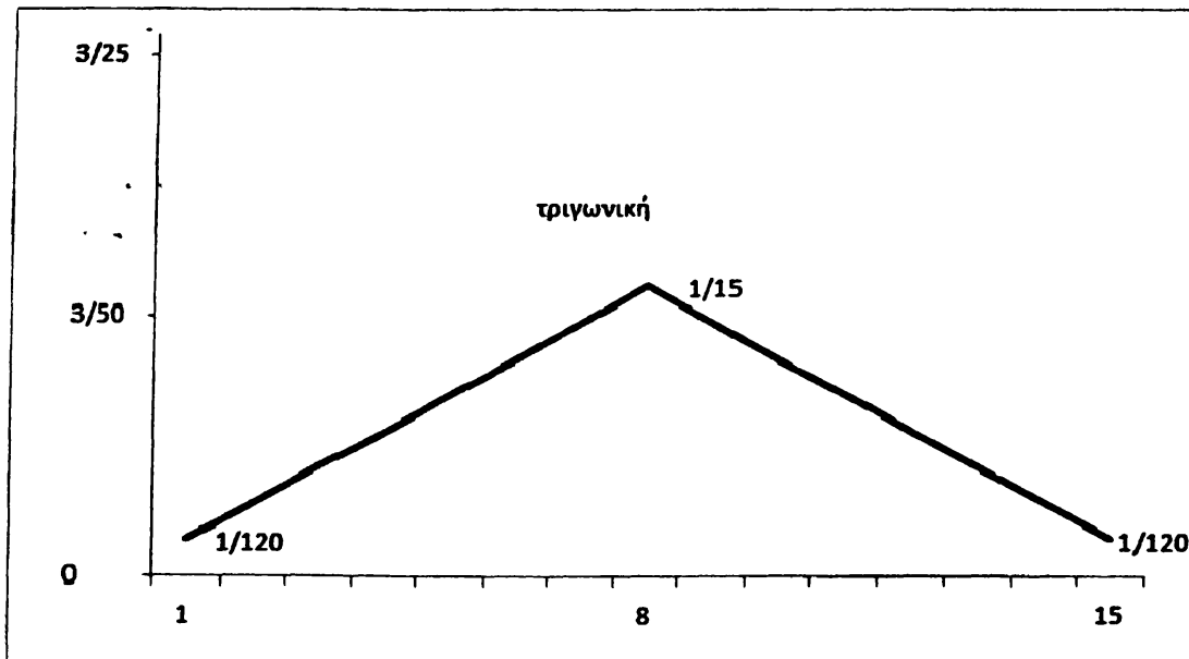
Σχήμα 6.20. Τριγωνική Κατανομή
