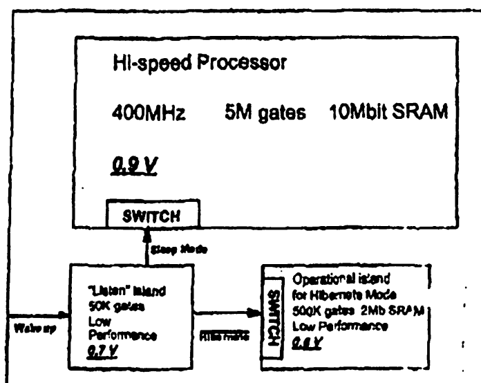
Σχήμα 3.9. Τμήμα Τάσης για Διάταξη Παροχής Ισχύος [12]
