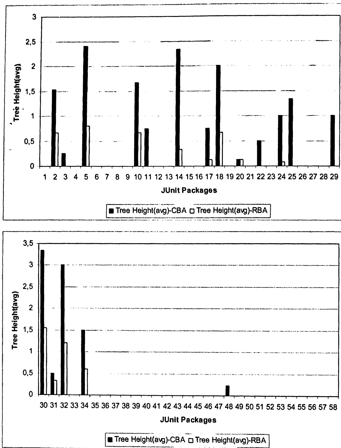
Σχήμα Α.27 Σύγκριση Μέσης Τιμής Ύψους Δένδρων CBA Average και RBA.
