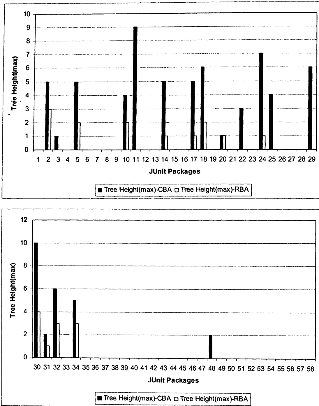
Σχήμα Α.25 Σύγκριση Μέγιστου Ύψους Δένδρων μεταξύ CBA Adaptive και RBA.
