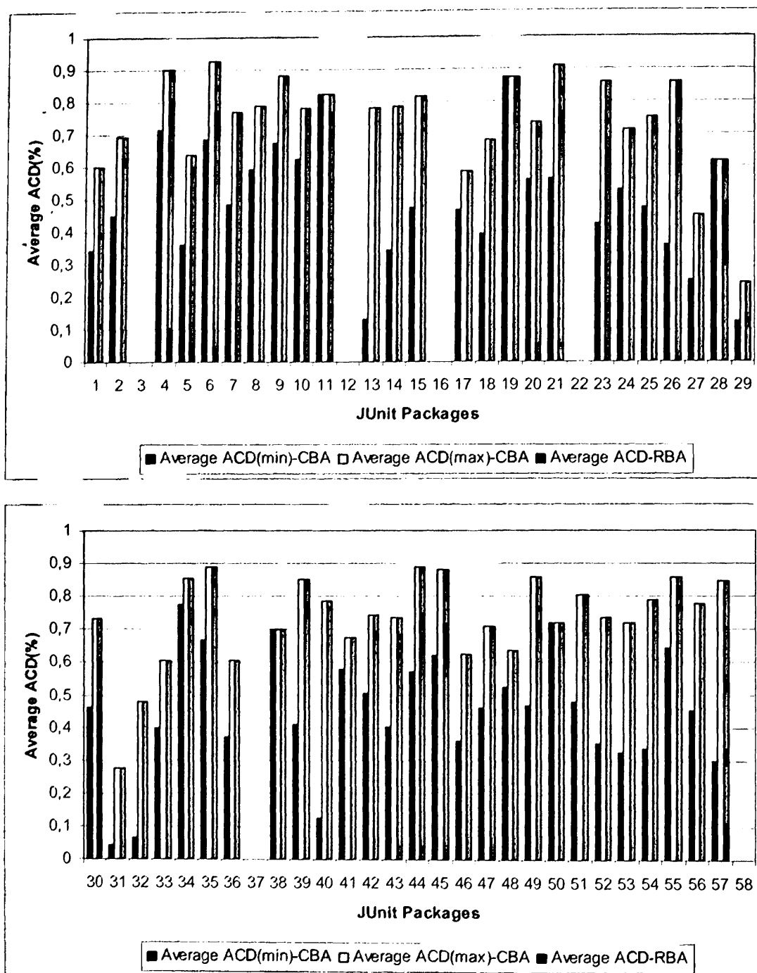
Σχήμα Α.1 Σύγκριση Μέσης Τιμής ACD μεταξύ CBA Single και RBA.
