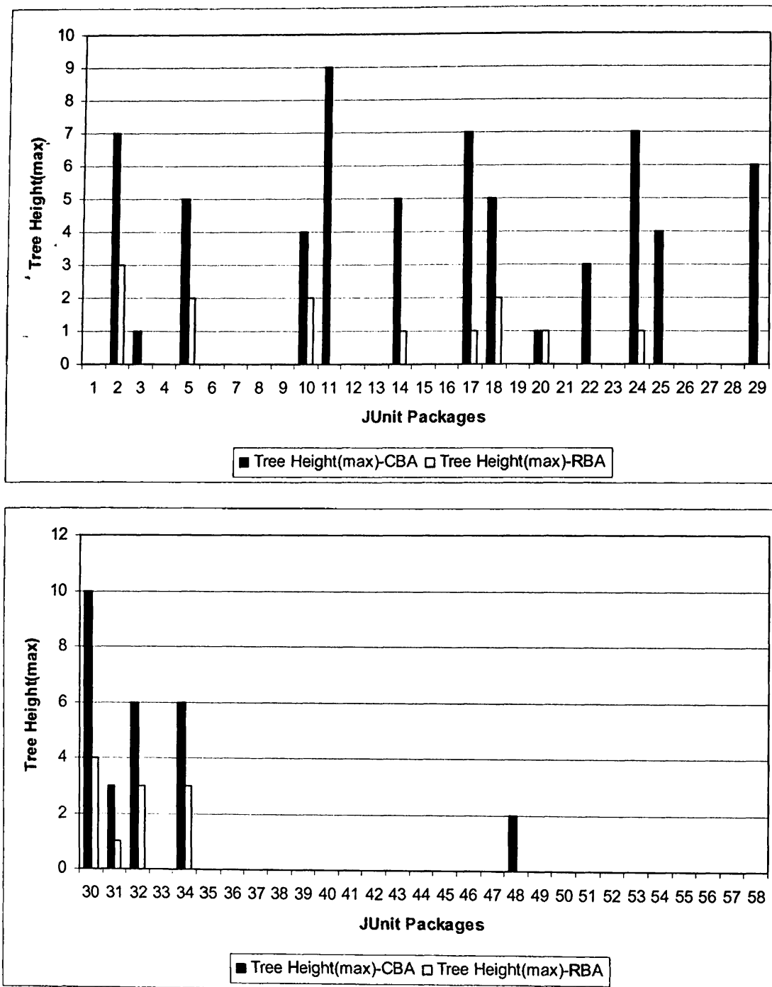
Σχήμα Α.21 Σύγκριση Μέγιστου Ύψους Δένδρων μεταξύ CBA Single και RBA.
