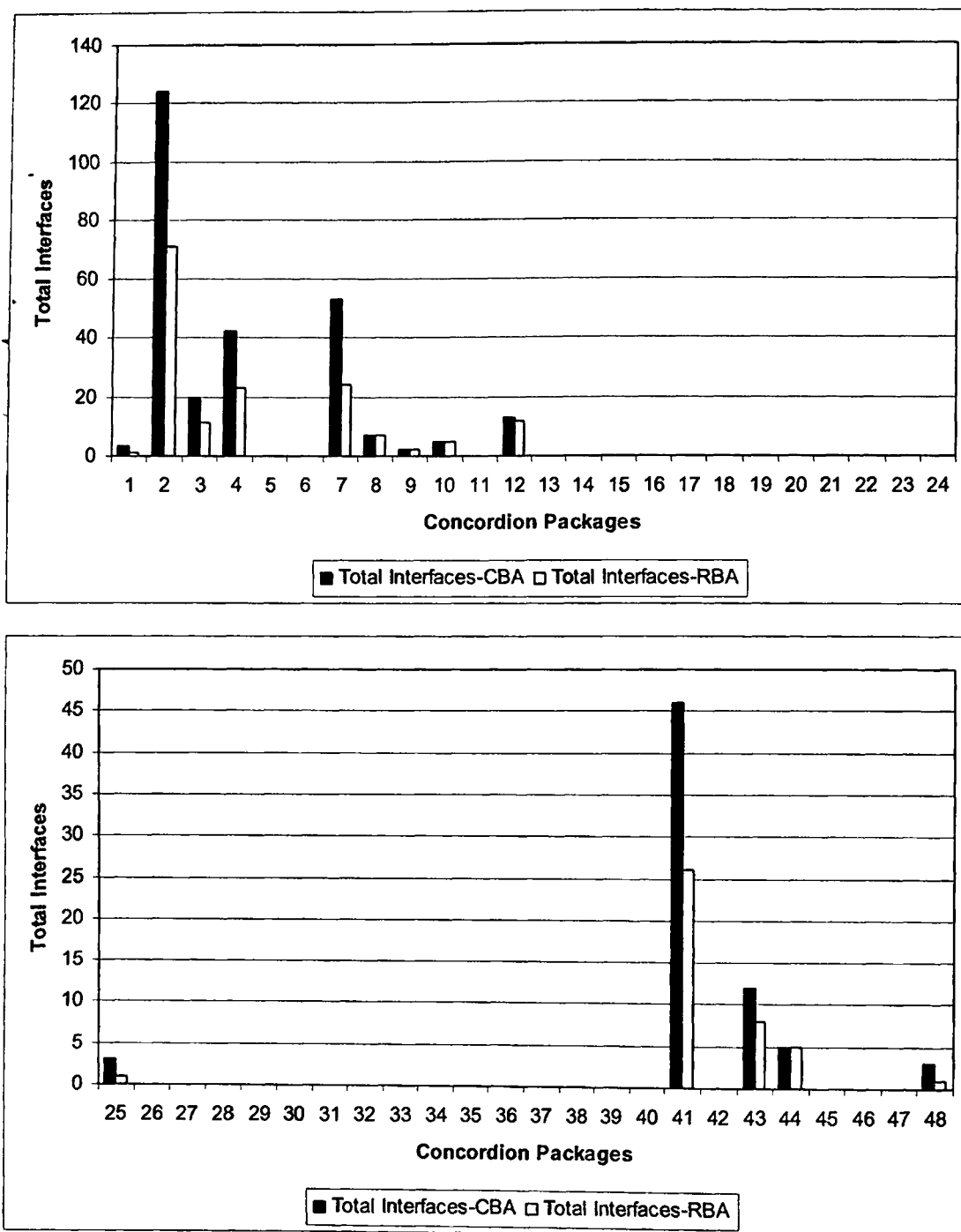
Σχήμα Β.11 Σύγκριση Συνολικού Πλήθους Διεπαφών μεταξύ CBA Single και RBA.
