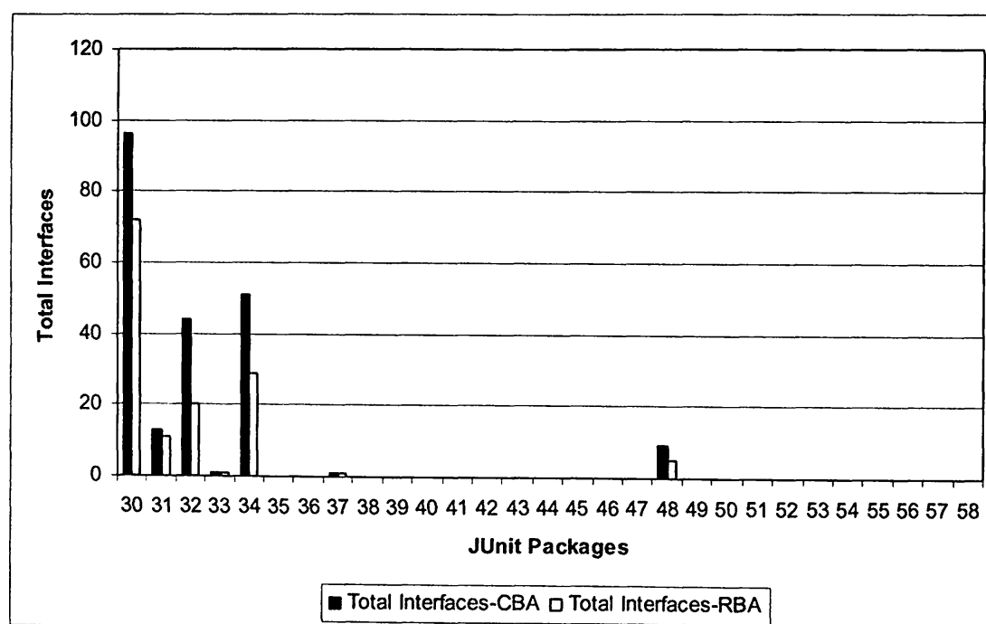
Σχήμα Α.12 Σύγκριση Συνολικού Πλήθους Διεπαφών μεταξύ CBA Average και RBA.
