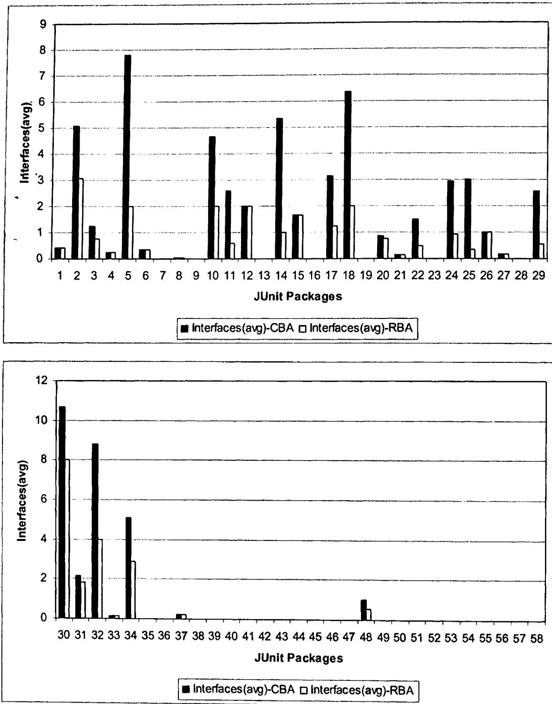
Σχήμα Α.20 Σύγκριση Μέσης Τιμής Πλήθους Διεπαφών μεταξύ CBA Adaptive και RBA.
