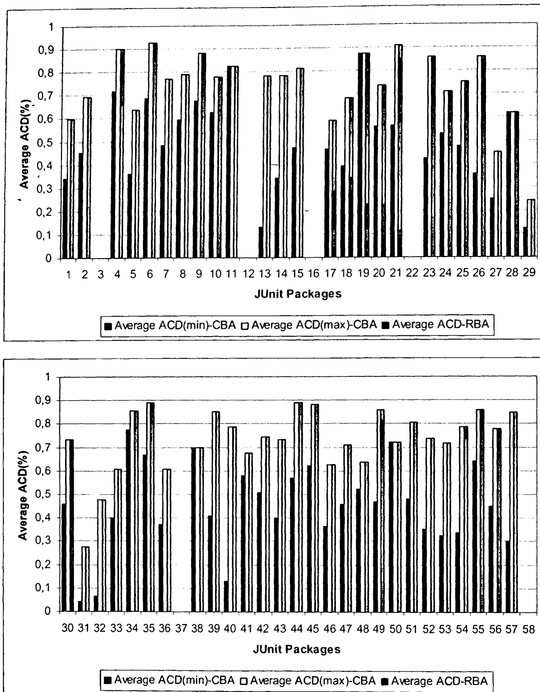
Σχήμα Α.5 Σύγκριση Μέσης Τιμής ACD μεταξύ CBA Adaptive και RBA.
