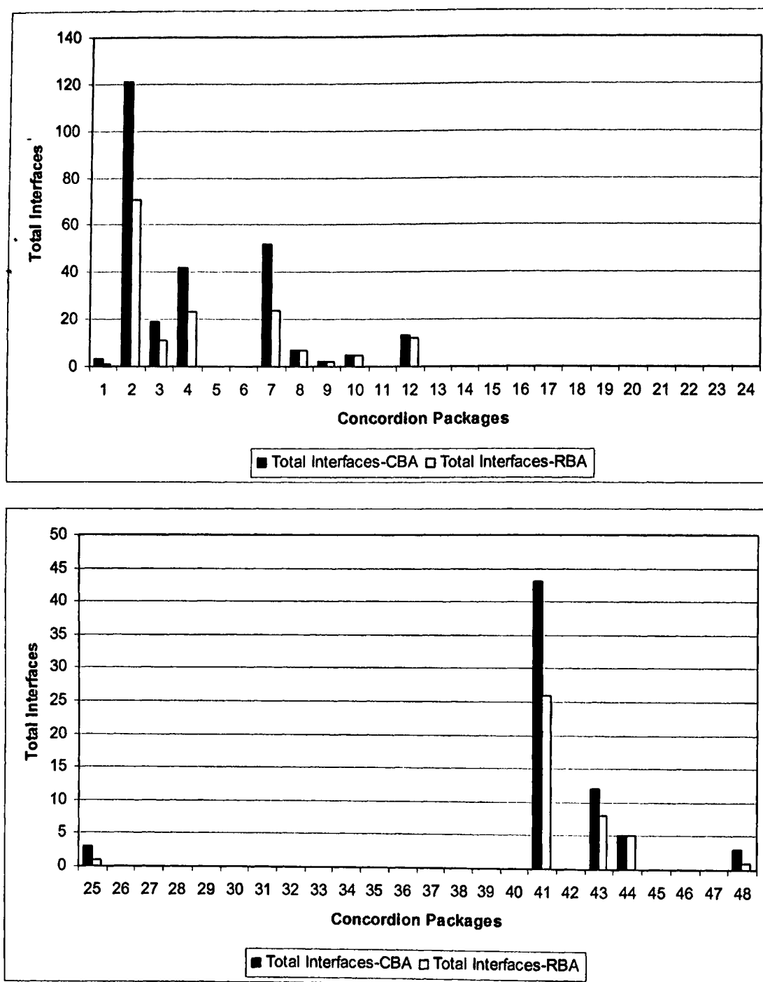
Σχήμα Β.14 Σύγκριση Συνολικού Πλήθους Διεπαφών μεταξύ CBA Median και RBA.
