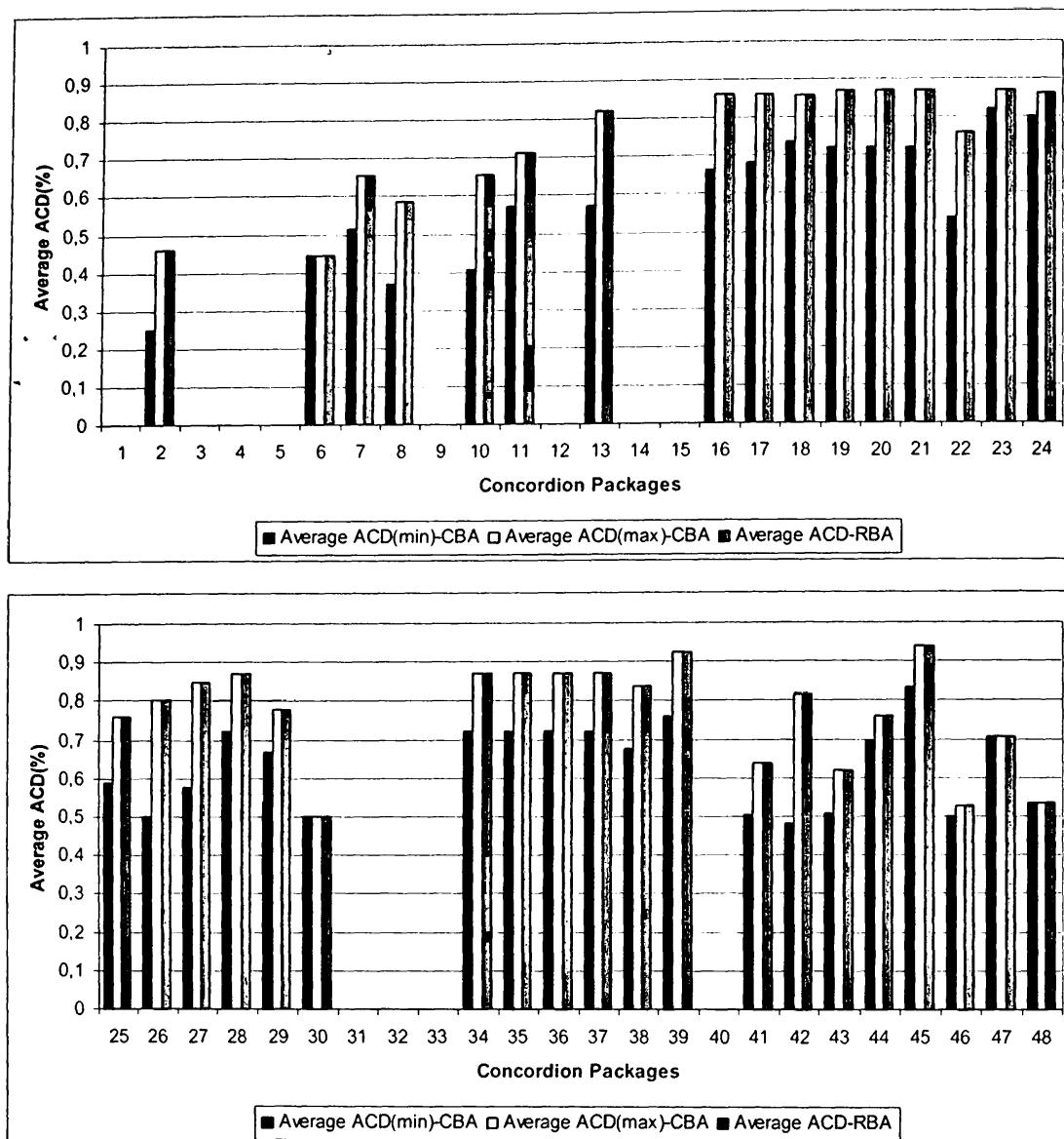
Σχήμα Β.4 Σύγκριση Μέσης Τιμής ACD μεταξύ CBA Median και RBA.
