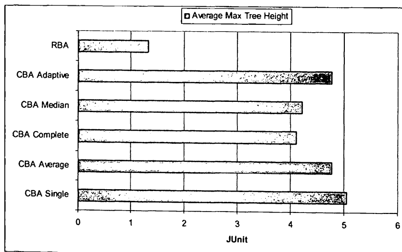
Σχήμα 5.3 Μέση τιμή Max Tree Height για το JUnit.
