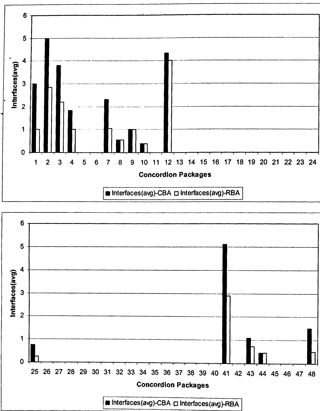
Σχήμα Β.16 Σύγκριση Μέσης Τιμής Πλήθους Διεπαφών μεταξύ CBA Single και RBA.
