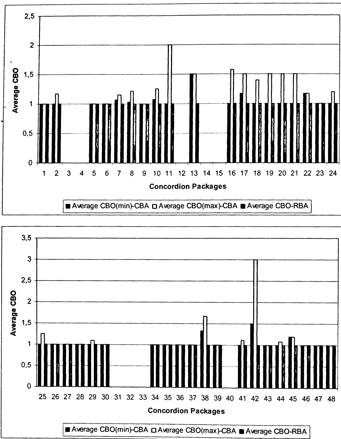
Σχήμα Β.9 Σύγκριση Μέσης Τιμής CBO μεταξύ CBA Median και RBA.
