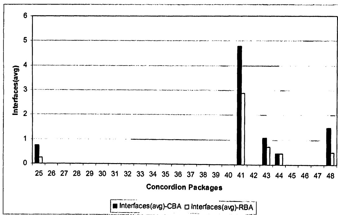
Σχήμα Β.19 Σύγκριση Μέσης Τιμής Πλήθους Διεπαφών μεταξύ CBA Median και RBA.
