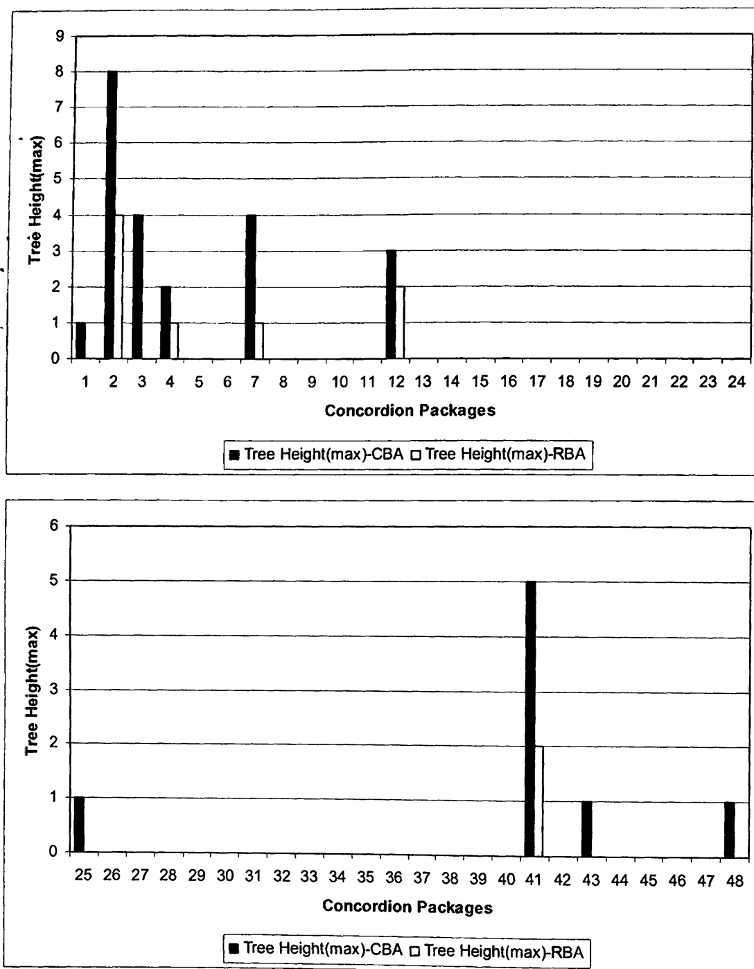
Σχήμα Β.22 Σύγκριση Μέγιστου Ύψους Δένδρων μεταξύ CBA Average και RBA.
