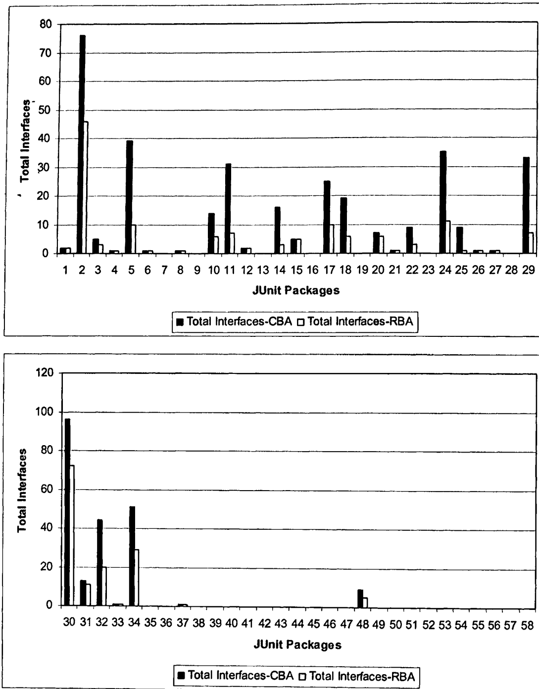
Σχήμα Α.11 Σύγκριση Συνολικού Πλήθους Διεπαφών μεταξύ CBA Single και RBA.
