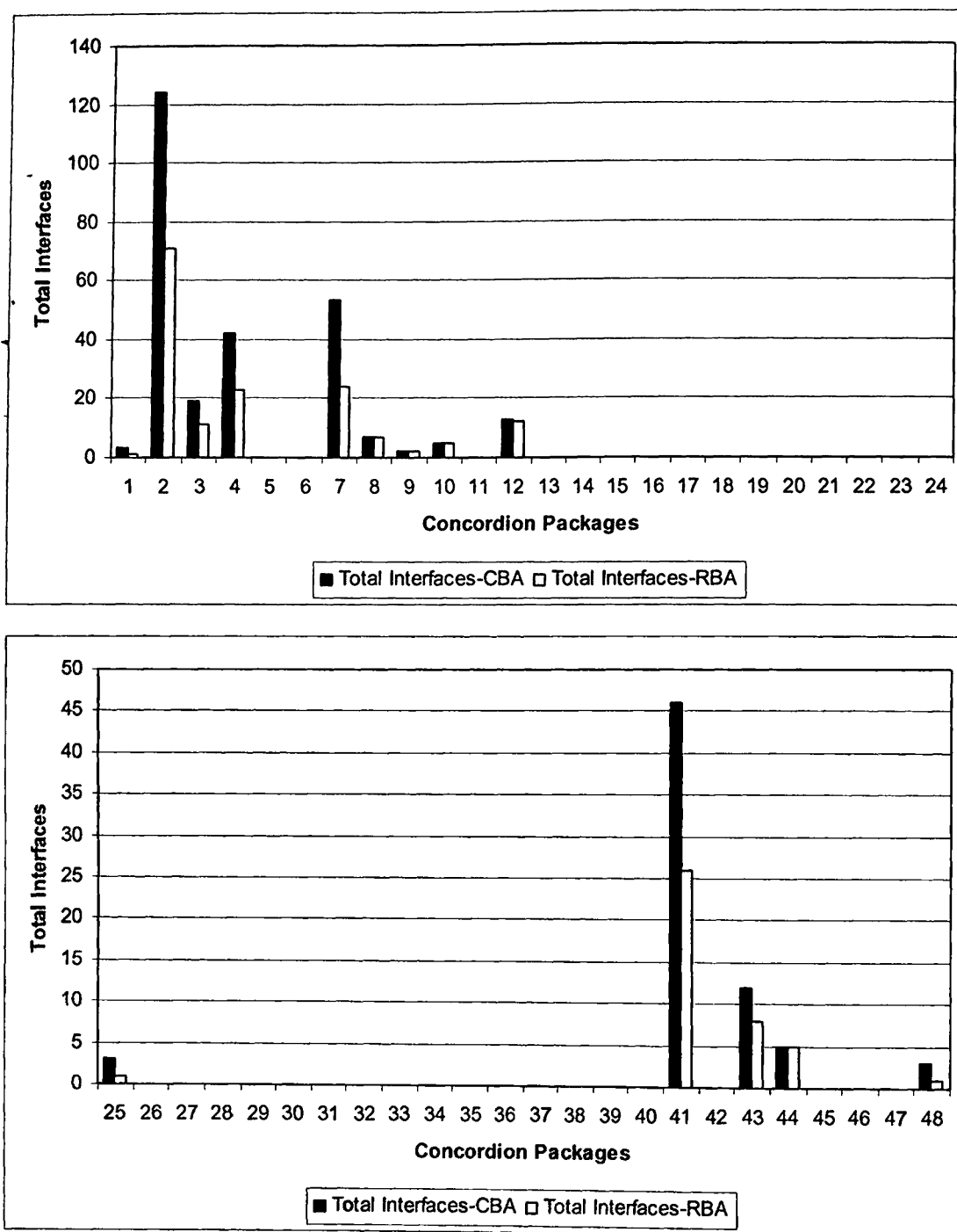
Σχήμα Β.12 Σύγκριση Συνολικού Πλήθους Διεπαφών μεταξύ CBA Average και RBA.
