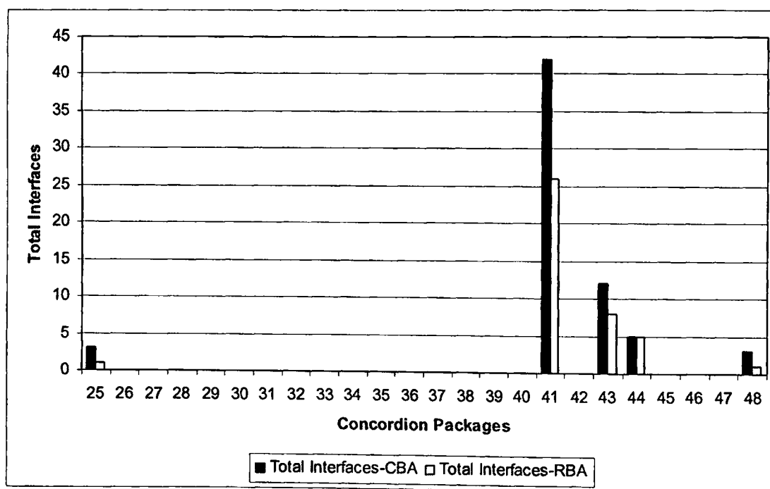
Σχήμα Β.13 Σύγκριση Συνολικού Πλήθους Διεπαφών μεταξύ CBA Complete και RBA.
