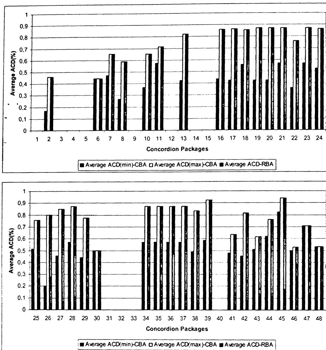
Σχήμα Β.5 Σύγκριση Μέσης Τιμής ACD μεταξύ CBA Adaptive και RBA.
