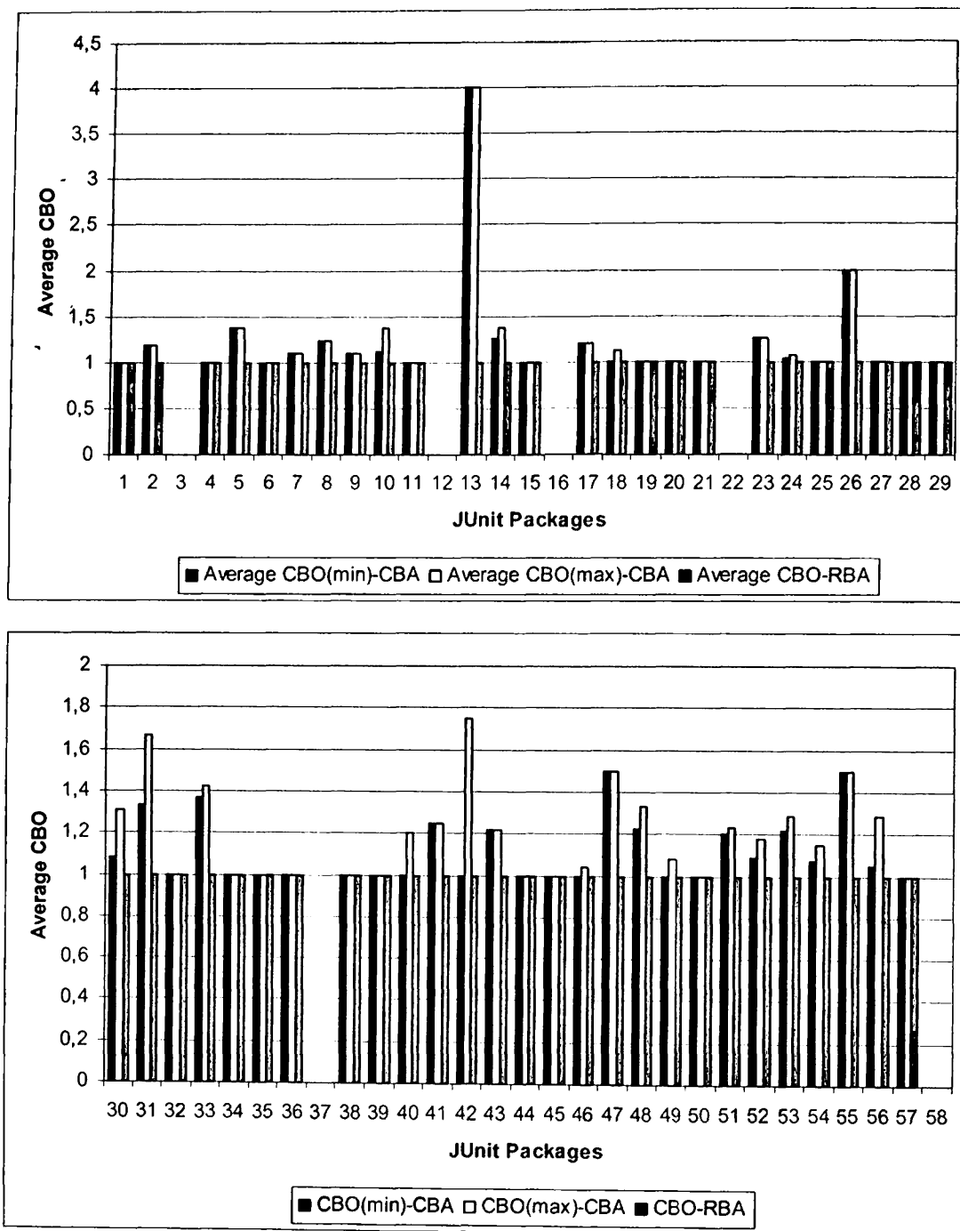
Σχήμα Α.8 Σύγκριση Μέσης Τιμής CBO μεταξύ CBA Complete και RBA.
