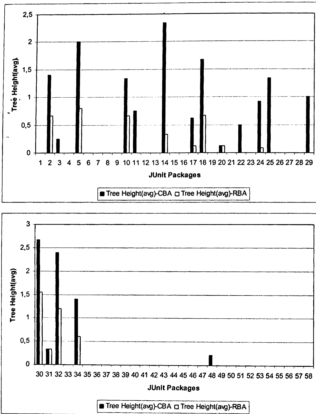
Σχήμα Α.29 Σύγκριση Μέσης Τιμής Ύψους Δένδρων CBA Median και RBA.
