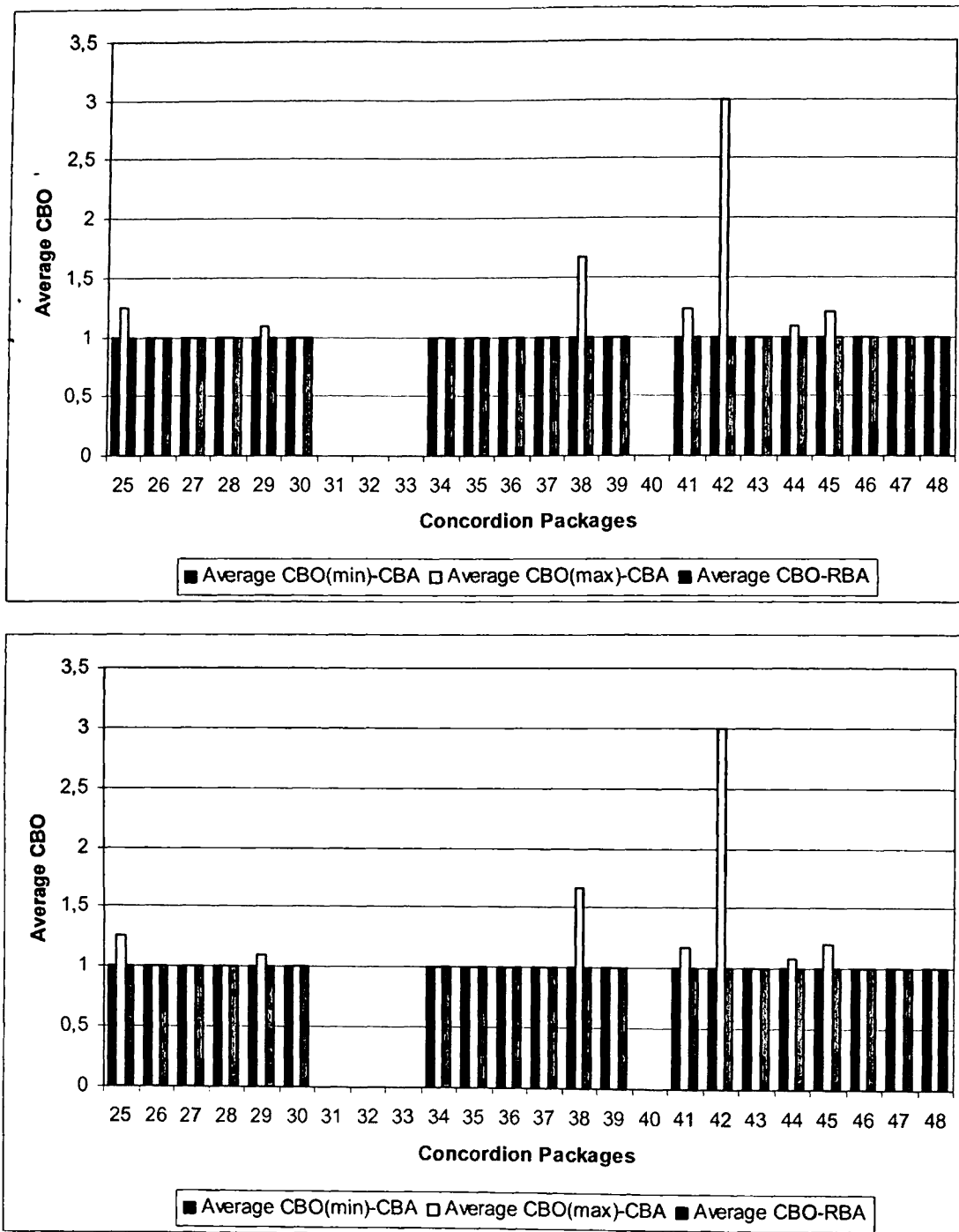
Σχήμα Β.7 Σύγκριση Μέσης Τιμής CBO μεταξύ CBA Average και RBA.
