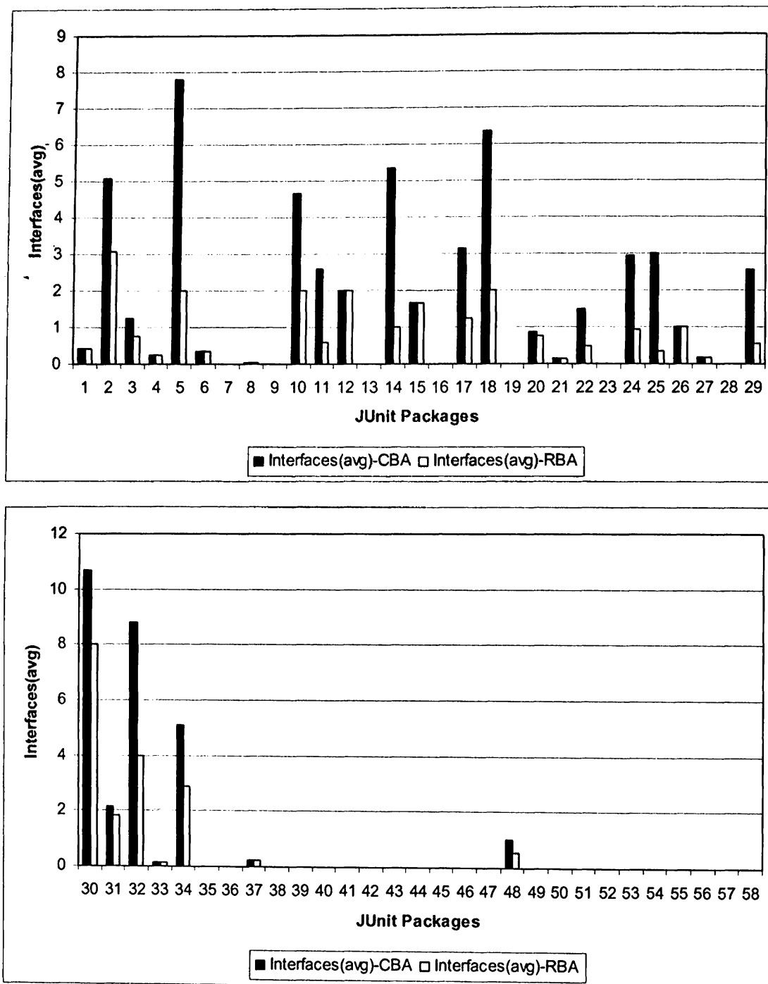
Σχήμα Α.17 Σύγκριση Μέσης Τιμής Πλήθους Διεπαφών μεταξύ CBA Average και RBA.
