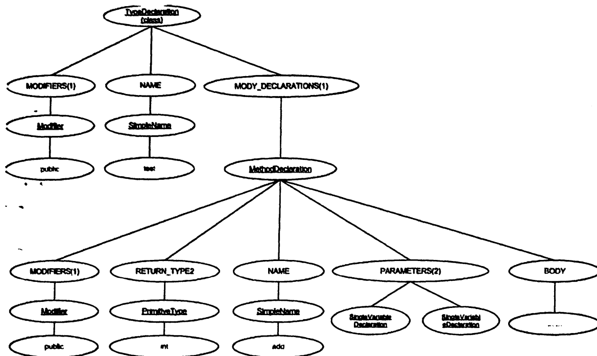
Σχήμα 4.9 Το αφηρημένο συντακτικό δένδρο για την κλάση Test.
