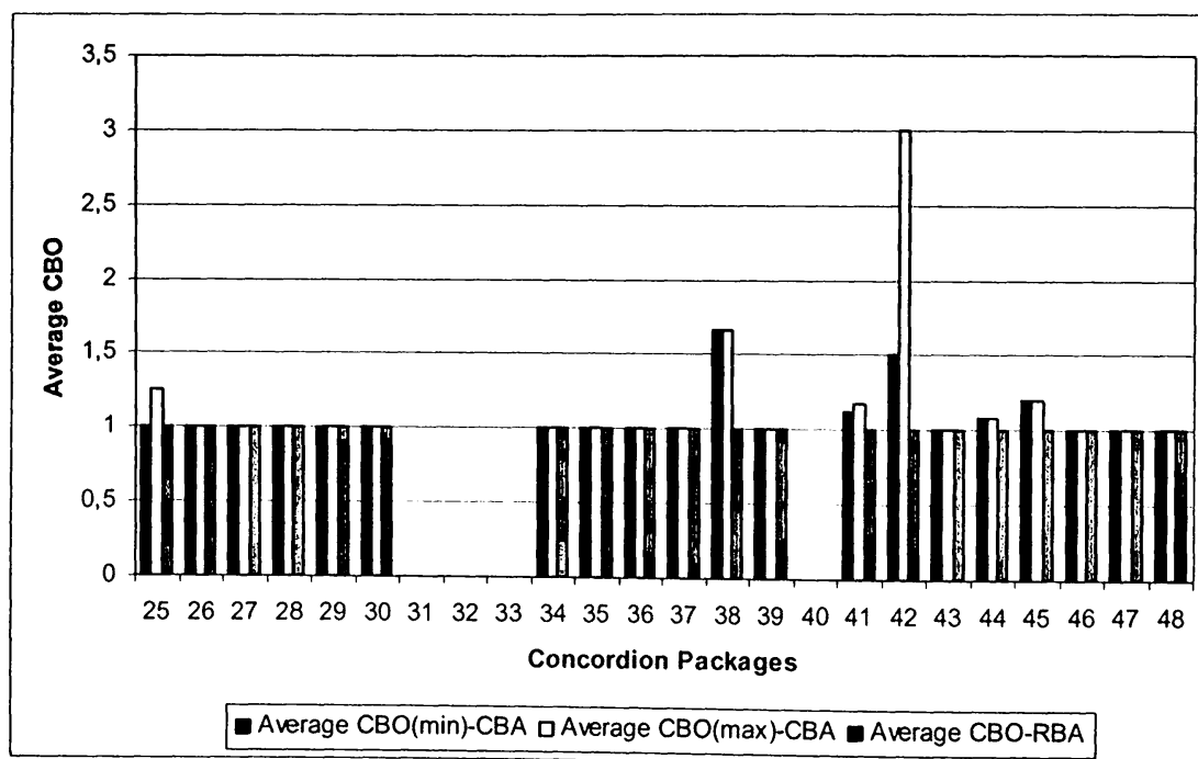
Σχήμα Β.8 Σύγκριση Μέσης Τιμής CBO μεταξύ CBA Complete και RBA.
