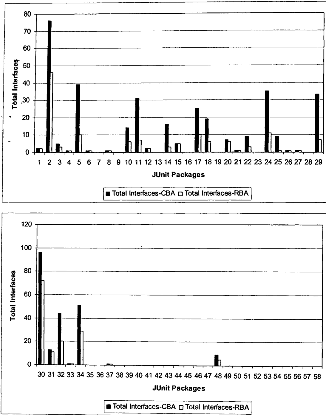
Σχήμα Α.15 Σύγκριση Συνολικού Πλήθους Διεπαφών μεταξύ CBA Adaptive και RBA.
