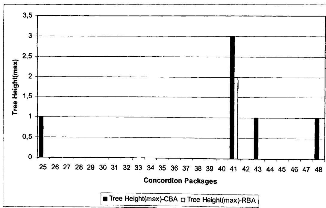
Σχήμα Β.24 Σύγκριση Μέγιστου Ύψους Δένδρων μεταξύ CBA Median και RBA.
