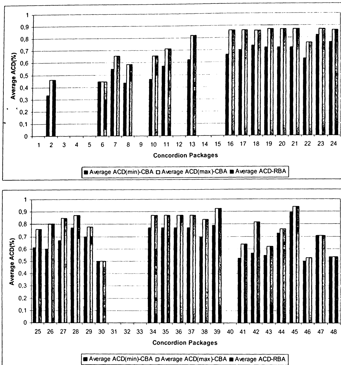
Σχήμα Β.3 Σύγκριση Μέσης Τιμής ACD μεταξύ CBA Complete και RBA.
