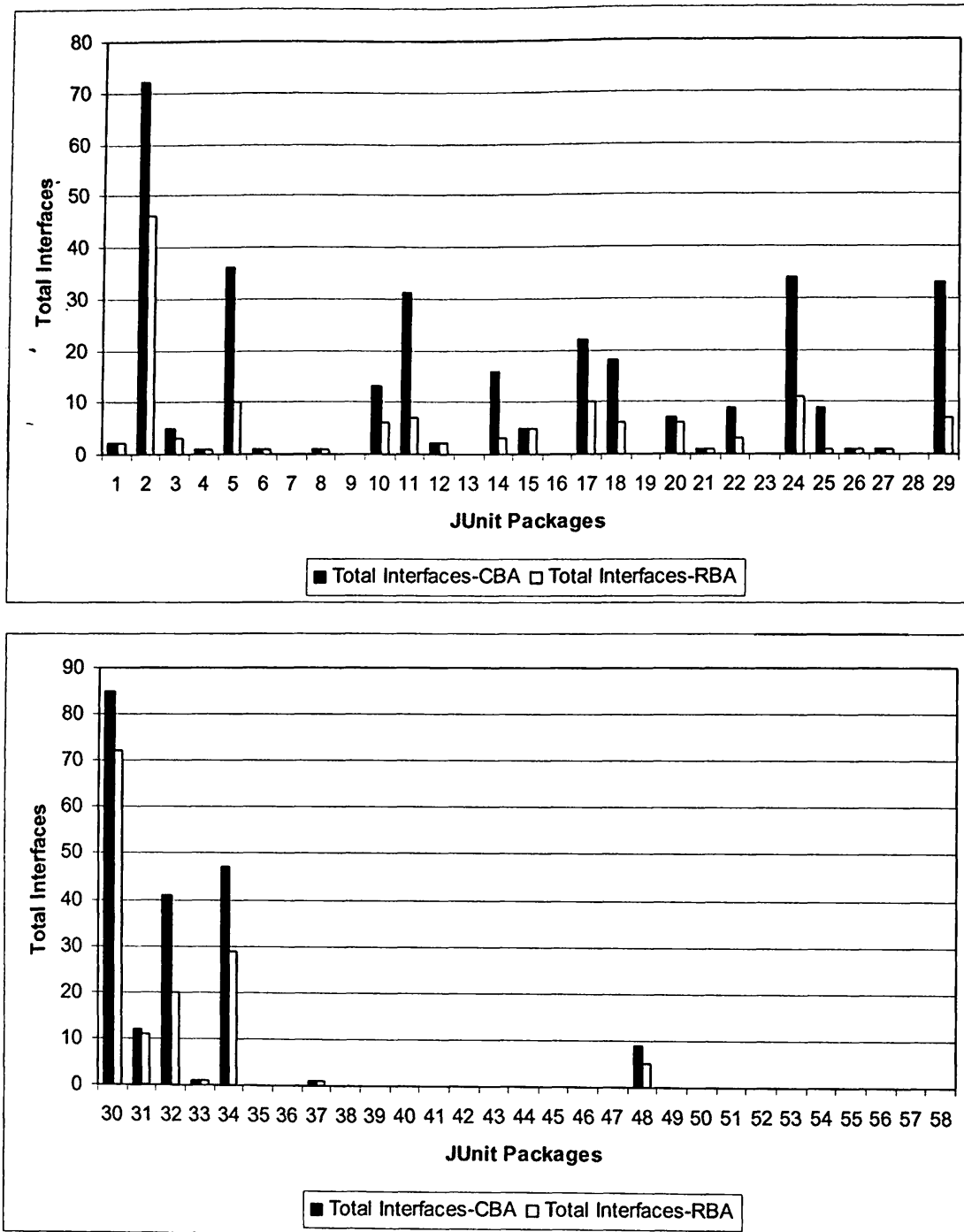
Σχήμα Α.13 Σύγκριση Συνολικού Πλήθους Διεπαφών μεταξύ CBA Complete και RBA.
