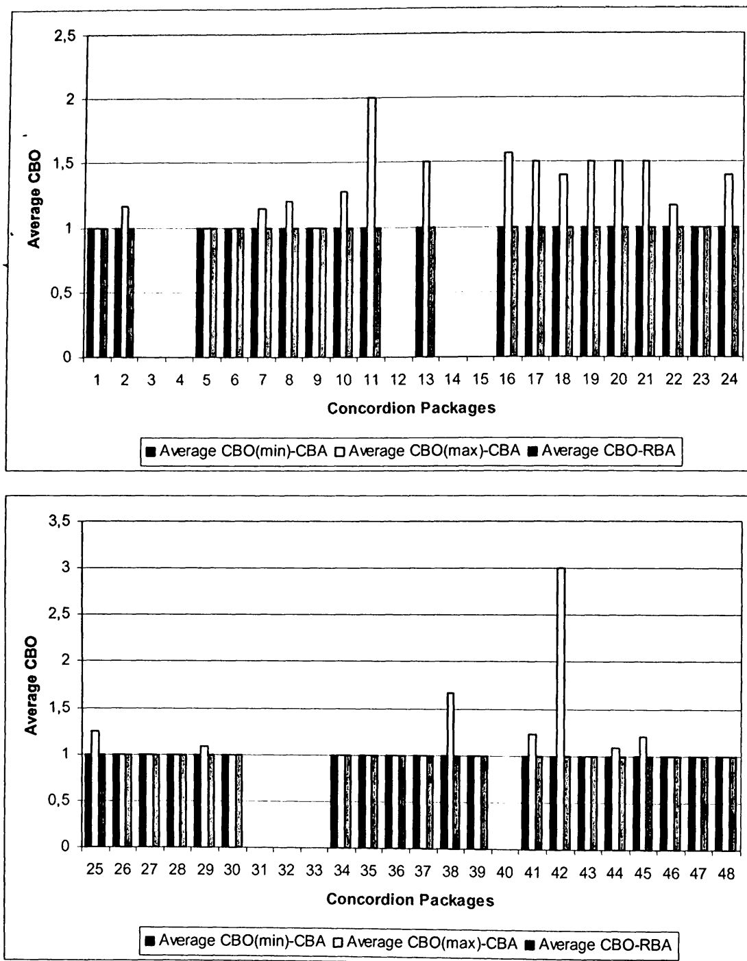
Σχήμα Β.10 Σύγκριση Μέσης Τιμής CBO μεταξύ CBA Adaptive και RBA.
