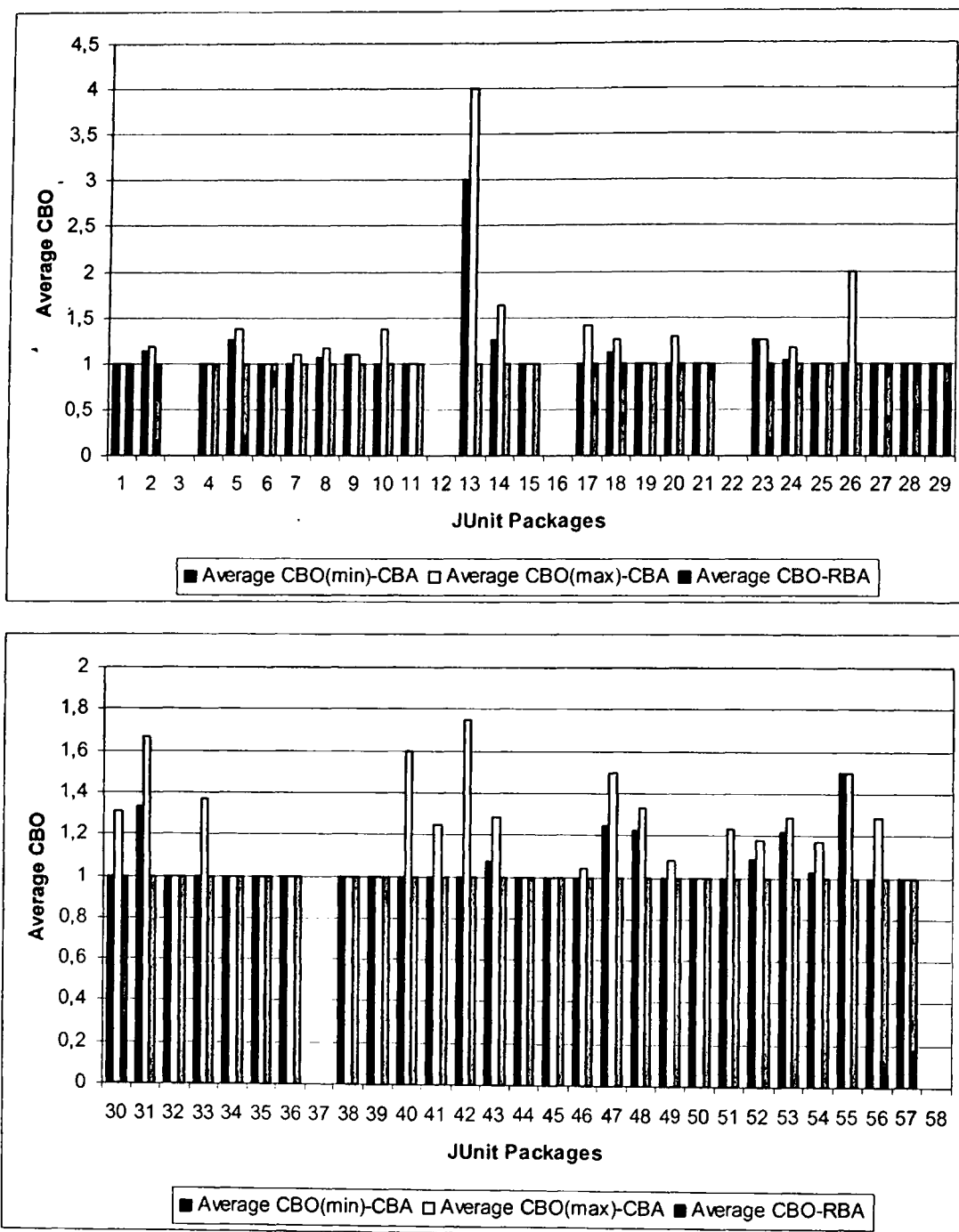
Σχήμα Α.9 Σύγκριση Μέσης Τιμής CBO μεταξύ CBA Median και RBA.
