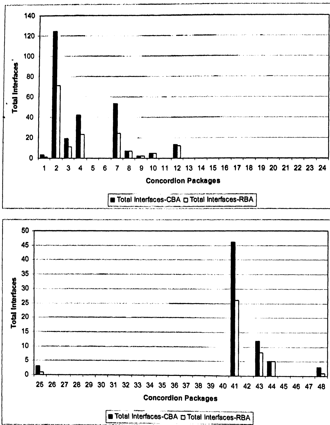
Σχήμα Β.15 Σύγκριση Συνολικού Πλήθους Διεπαφών μεταξύ CBA Adaptive και RBA.
