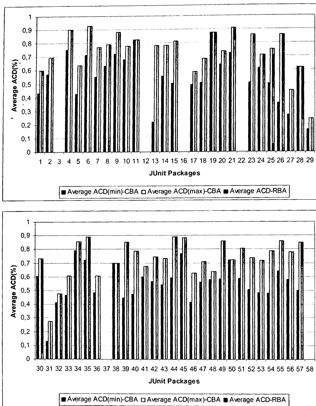
Σχήμα Α.4 Σύγκριση Μέσης Τιμής ACD μεταξύ CBA Median και RBA.
