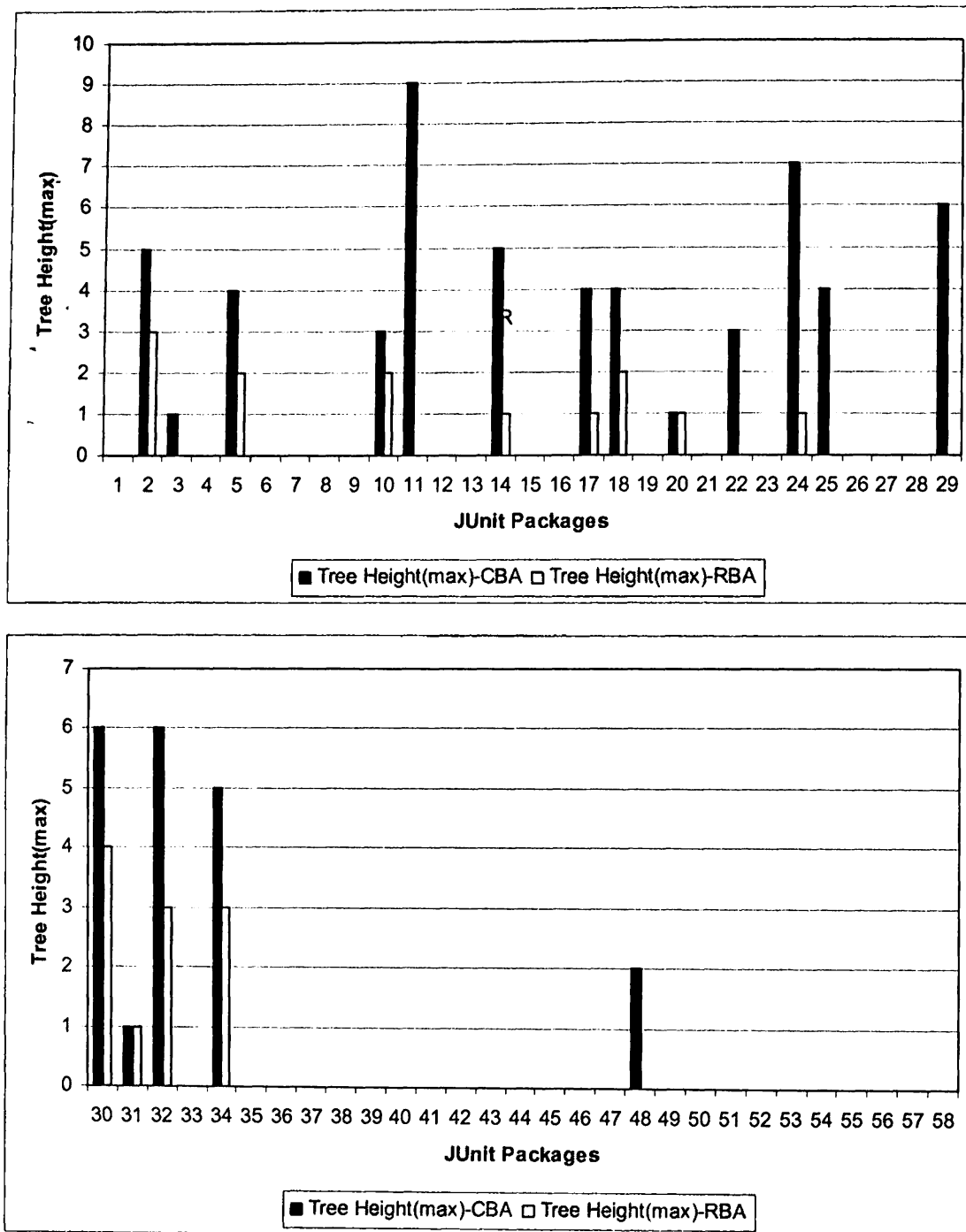
Σχήμα Α.24 Σύγκριση Μέγιστου Ύψους Δένδρων μεταξύ CBA Median και RBA.
