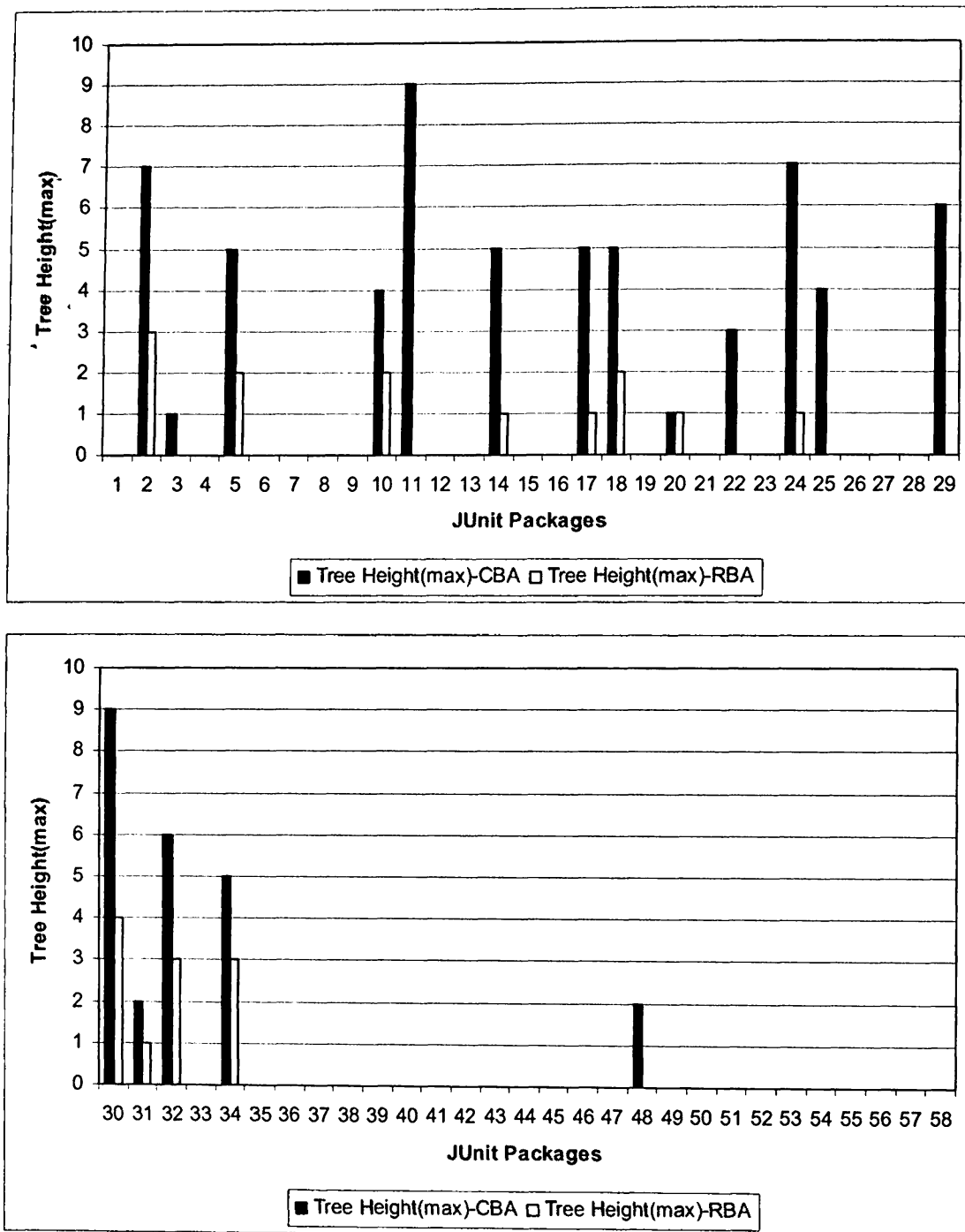
Σχήμα A.22 Σύγκριση Μέγιστου Ύψους Δένδρων μεταξύ CBA Average και RBA.
