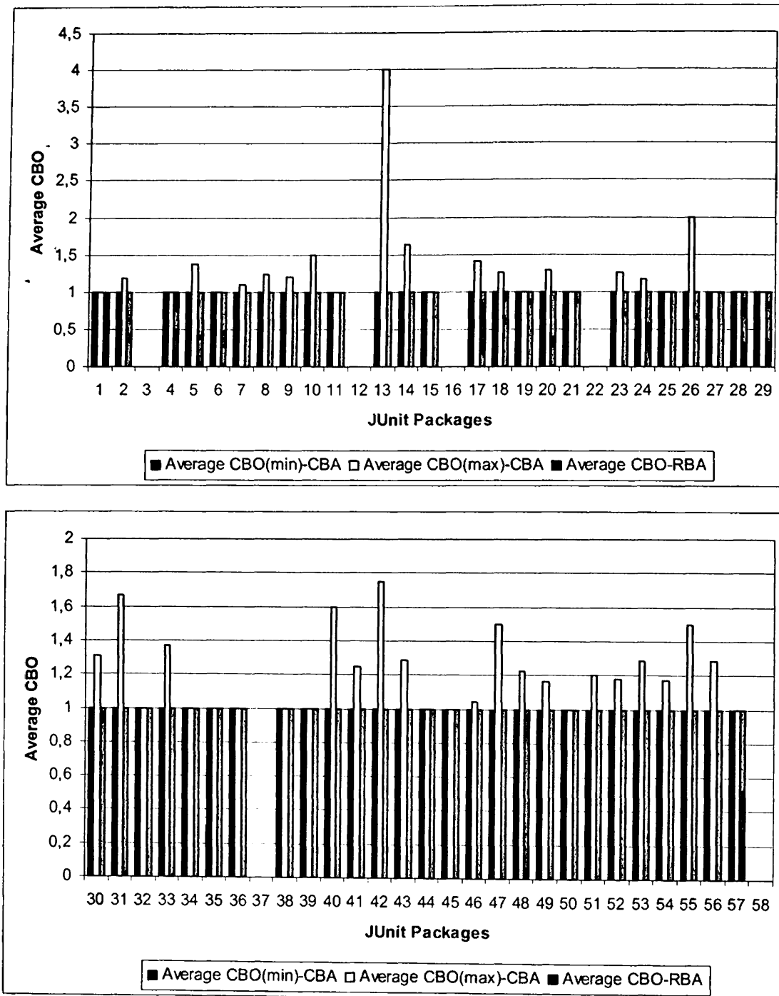
Σχήμα Α.10 Σύγκριση Μέσης Τιμής CBO μεταξύ CBA Adaptive και RBA.
