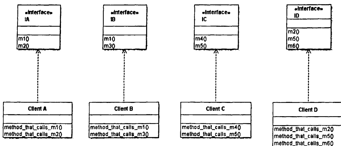
Σχήμα 1.2 Η σχεδίαση με εφαρμογή της ISP.
