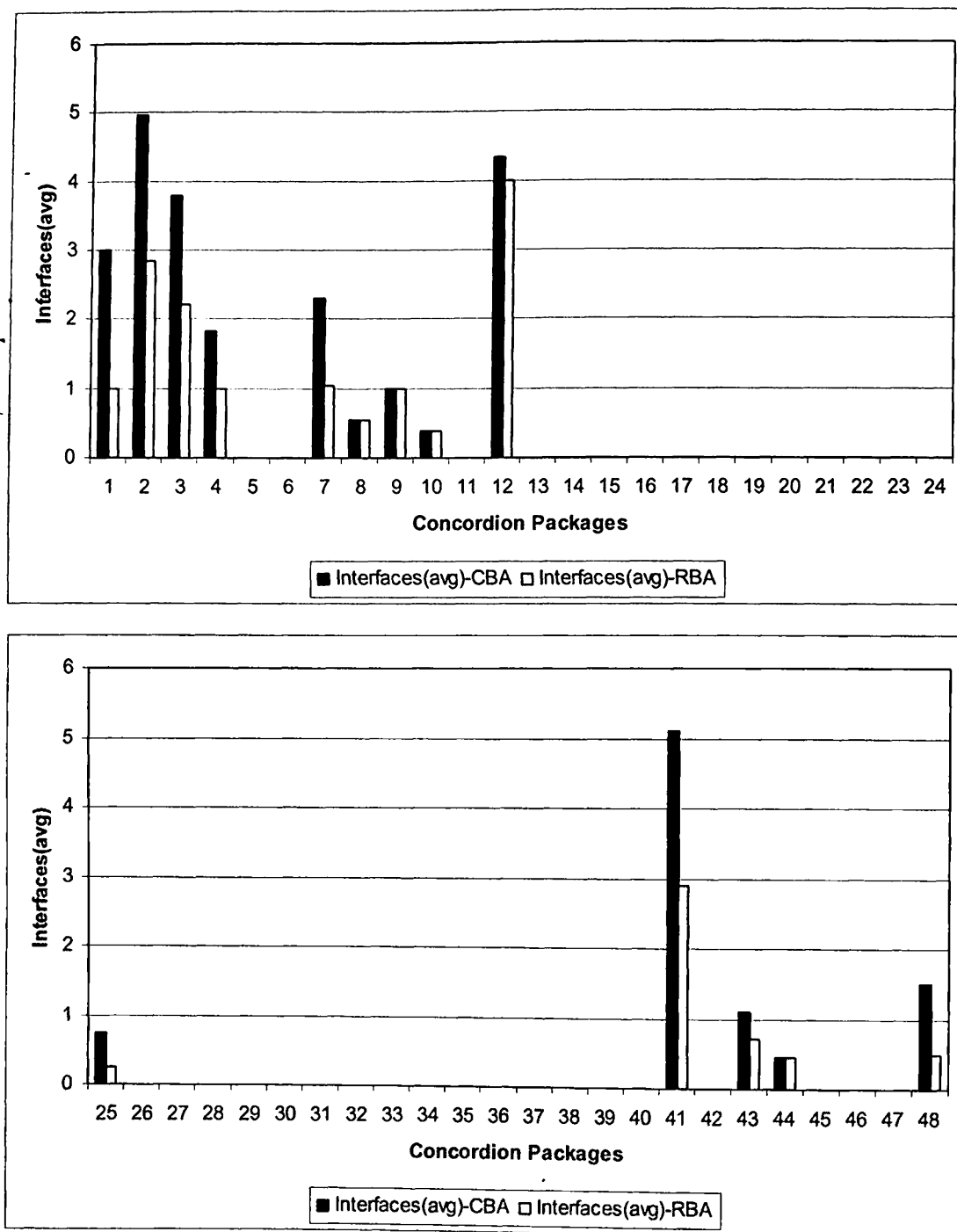
Σχήμα Β.20 Σύγκριση Μέσης Τιμής Πλήθους Διεπαφών μεταξύ CBA Adaptive και RBA.
