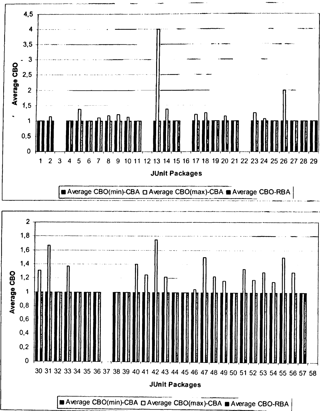
Σχήμα Α.7 Σύγκριση Μέσης Τιμής CBO μεταξύ CBA Average και RBA.
