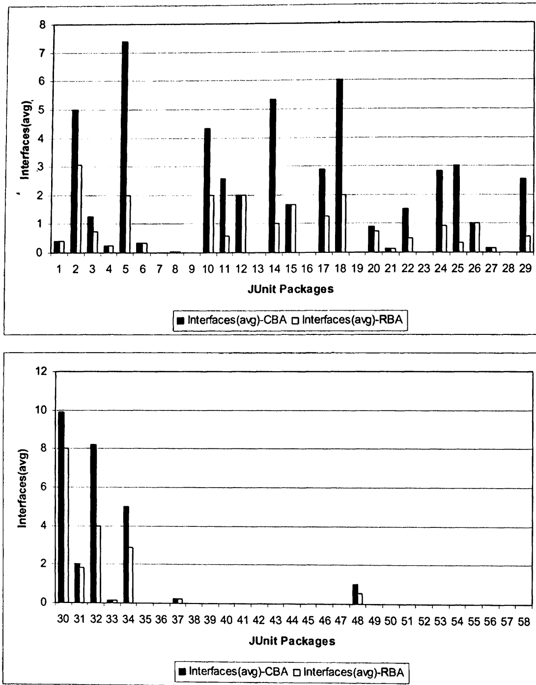
Σχήμα Α.19 Σύγκριση Μέσης Τιμής Πλήθους Διεπαφών μεταξύ CBA Median και RBA.
