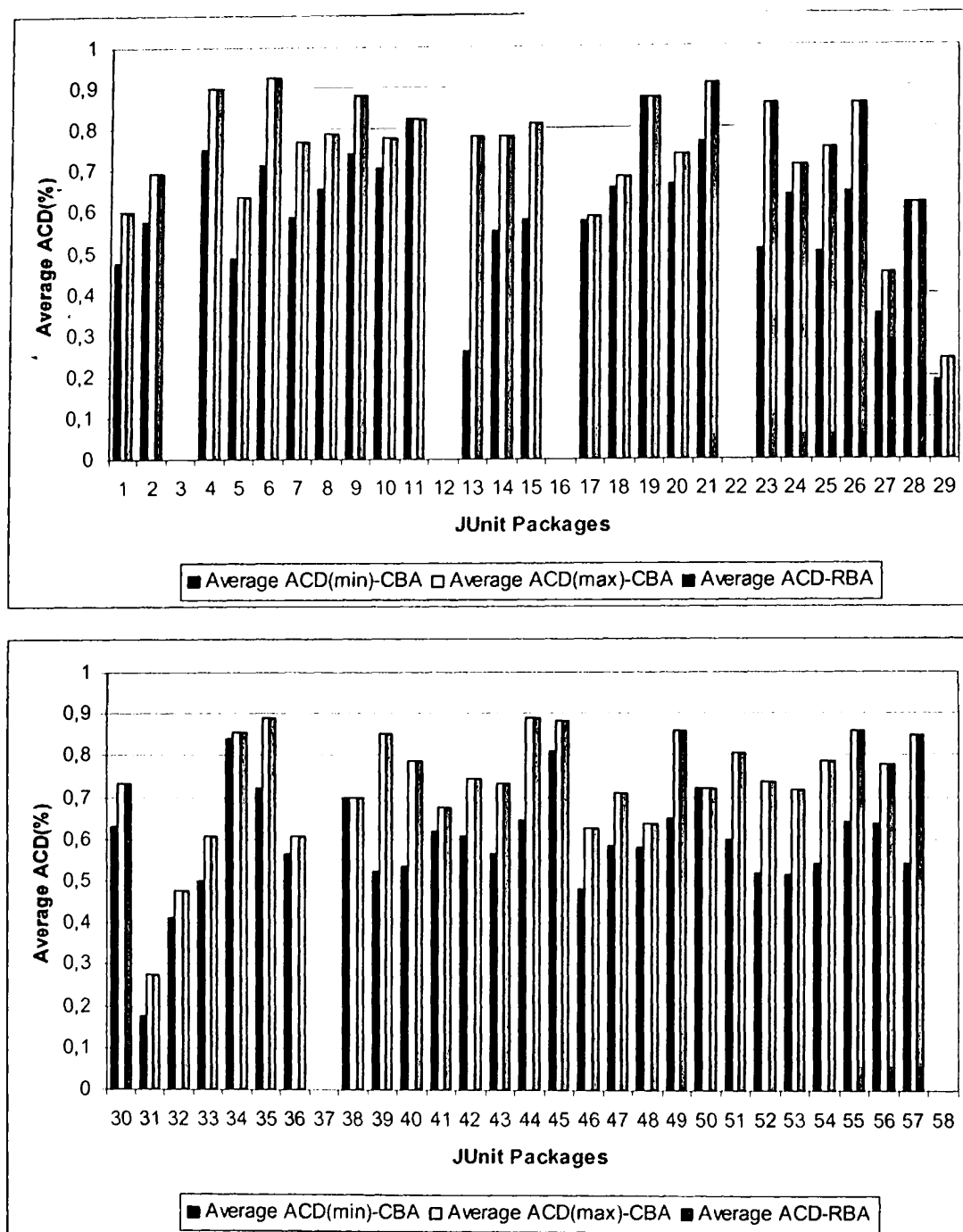
Σχήμα Α.3 Σύγκριση Μέσης Τιμής ACD μεταξύ CBA Complete και RBA.
