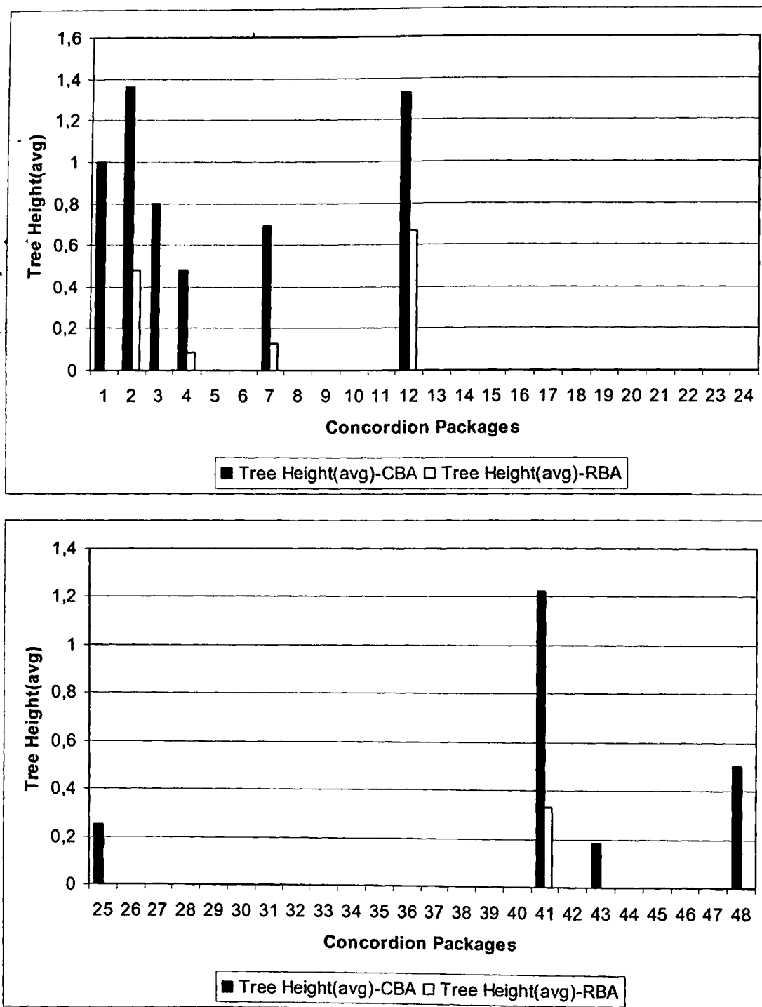
Σχήμα Β.26 Σύγκριση Μέσης Τιμής Ύψους Δένδρων CBA Single και RBA.
