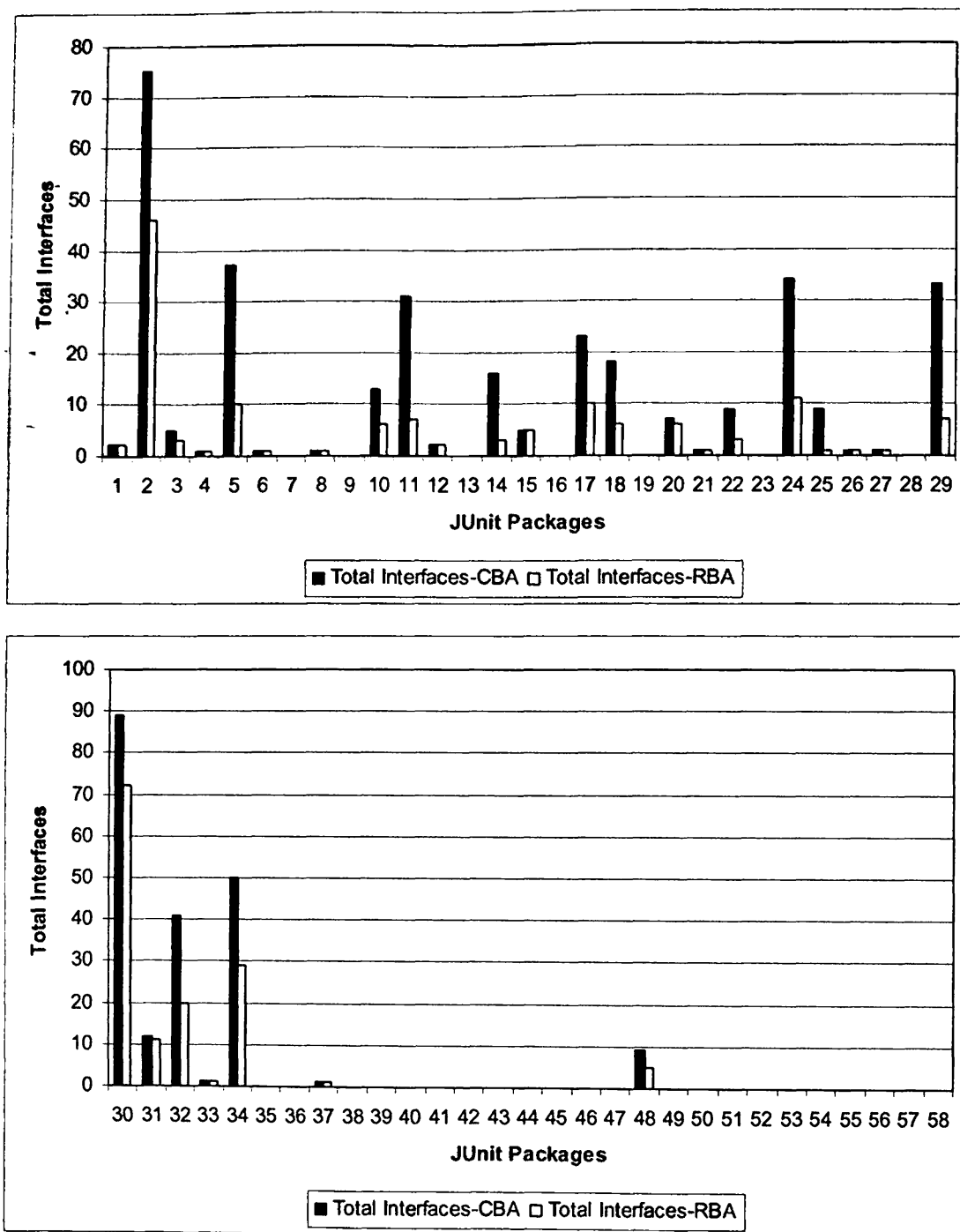
Σχήμα Α.14 Σύγκριση Συνολικού Πλήθους Διεπαφών μεταξύ CBA Median και RBA.
