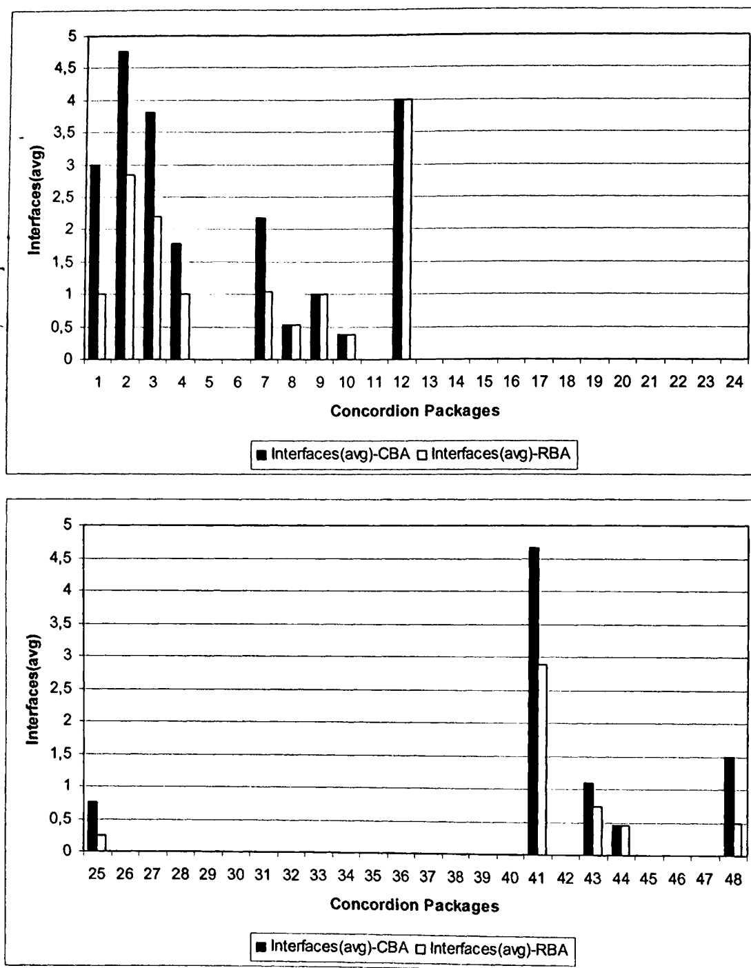
Σχήμα Β.18 Σύγκριση Μέσης Τιμής Πλήθους Διεπαφών μεταξύ CBA Complete και RBA.
