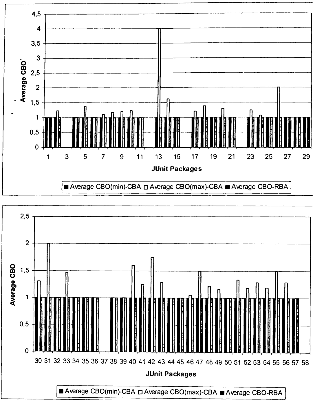
Σχήμα Α.6 Σύγκριση Μέσης Τιμής CBO μεταξύ CBA Single και RBA.
