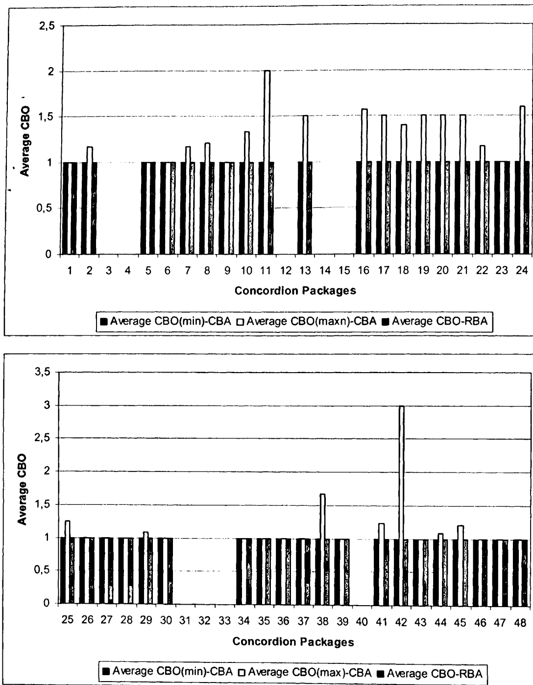
Σχήμα Β.6 Σύγκριση Μέσης Τιμής CBO μεταξύ CBA Single και RBA.
