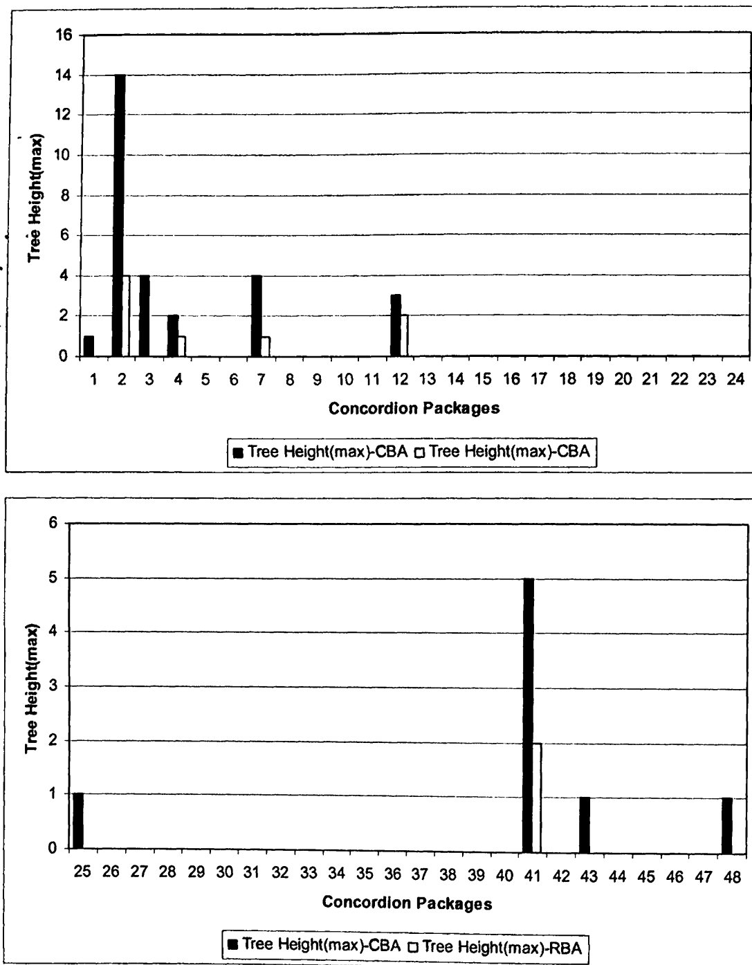
Σχήμα Β.21 Σύγκριση Μέγιστου Ύψους Δένδρων μεταξύ CBA Single και RBA.
