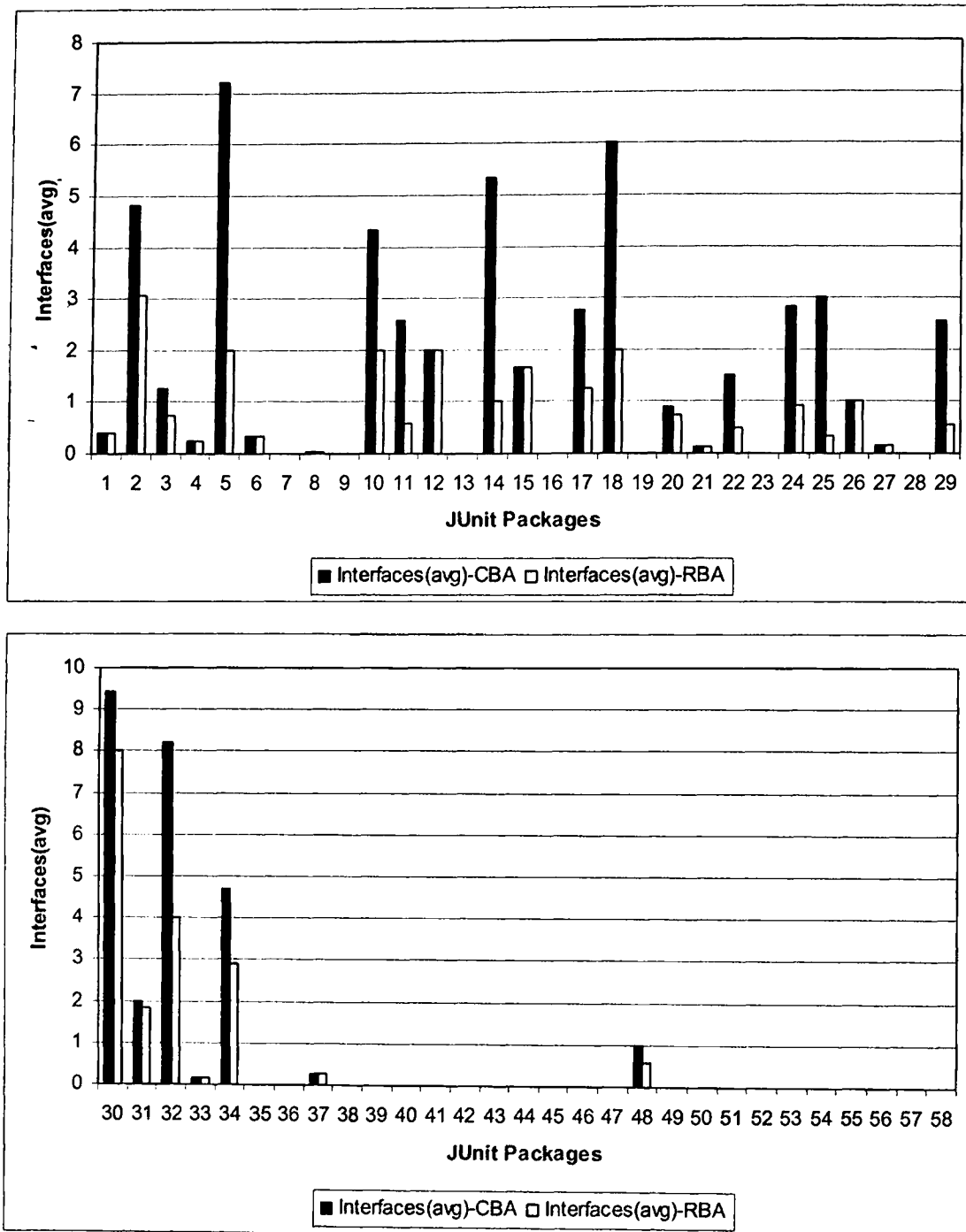
Σχήμα Α.18 Σύγκριση Μέσης Τιμής Πλήθους Διεπαφών μεταξύ CBA Complete και RBA.
