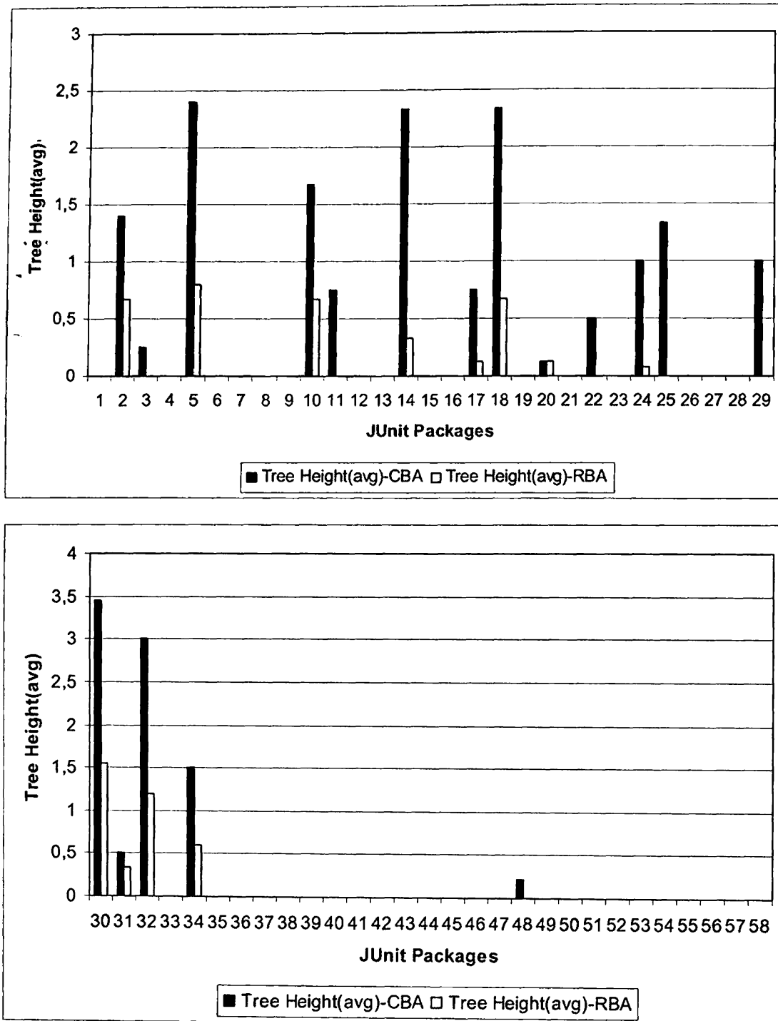
Σχήμα Α.30 Σύγκριση Μέσης Τιμής Ύψους Δένδρων CBA Adaptive και RBA.
