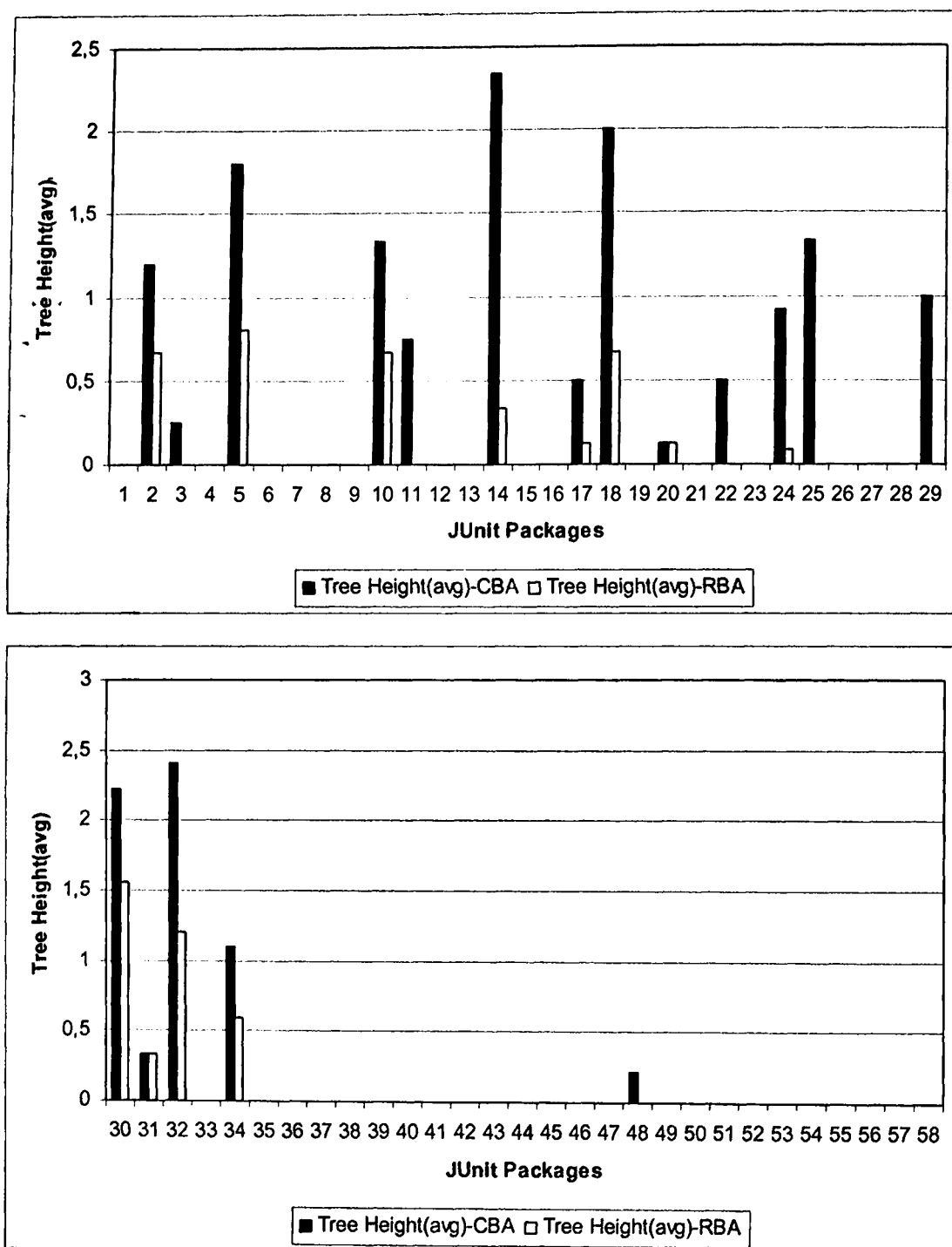
Σχήμα Α.28 Σύγκριση Μέσης Τιμής Ύψους Δένδρων CBA Complete και RBA.
