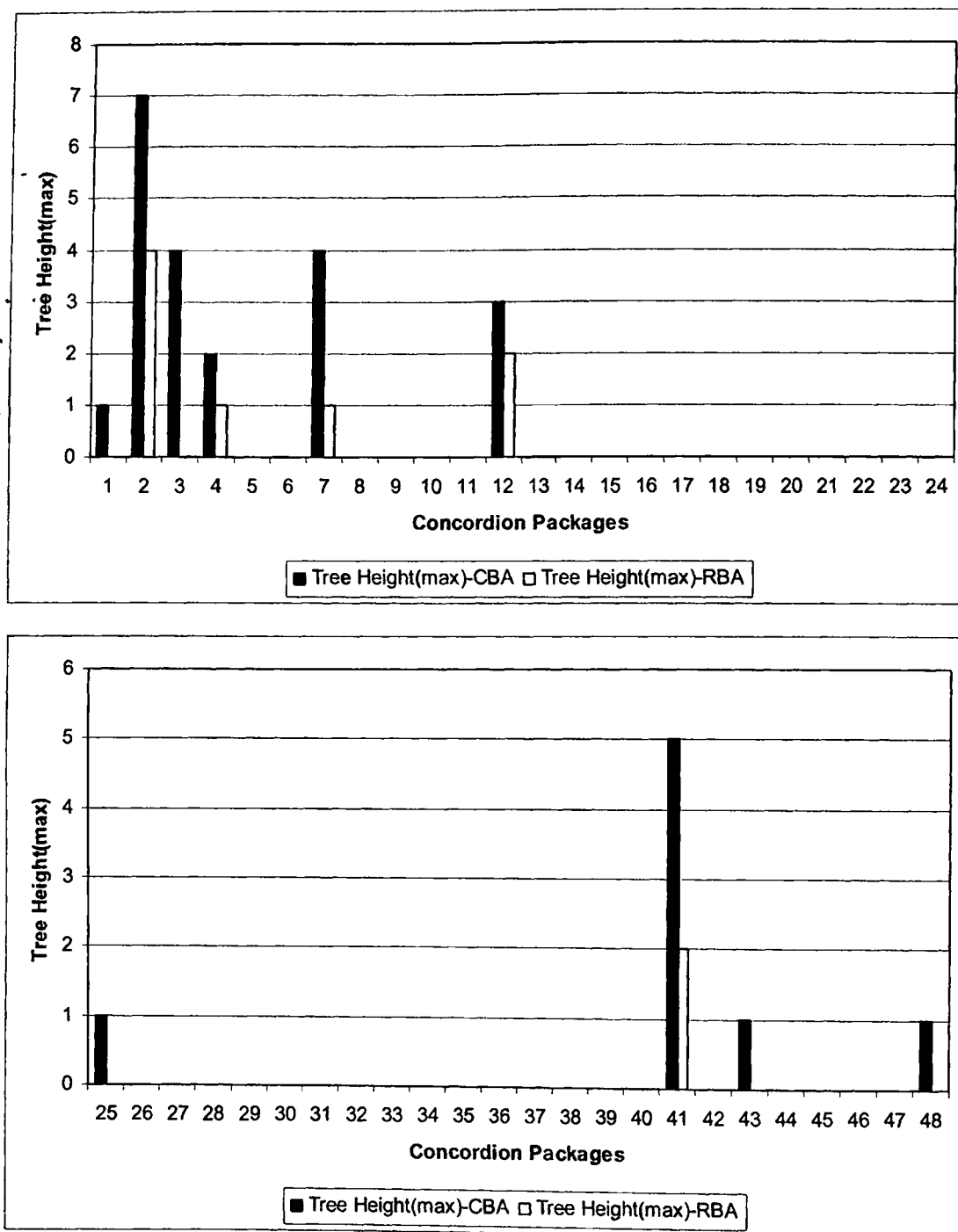
Σχήμα Β.25 Σύγκριση Μέγιστου Ύψους Δένδρων μεταξύ CBA Adaptive και RBA.
