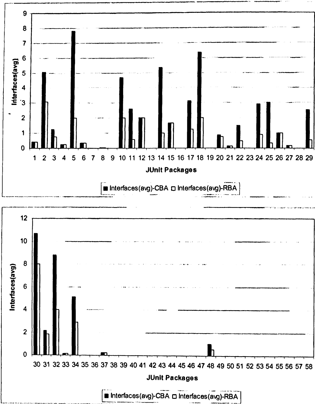
Σχήμα A.16 Σύγκριση Μέσης Τιμής Πλήθους Διεπαφών μεταξύ CBA Single και RBA.
