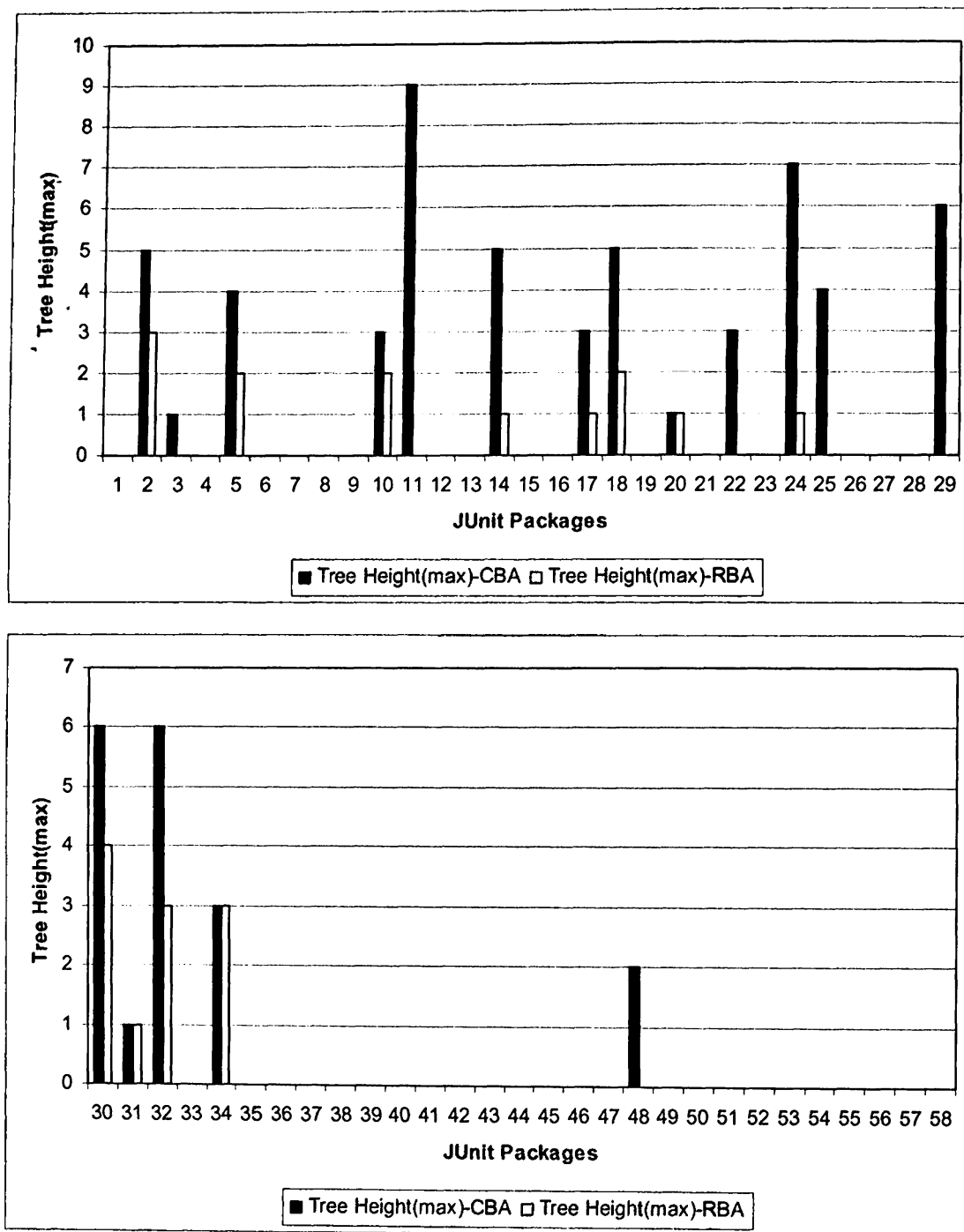
Σχήμα Α.23 Σύγκριση Μέγιστου Ύψους Δένδρων μεταξύ CBA Complete και RBA.
