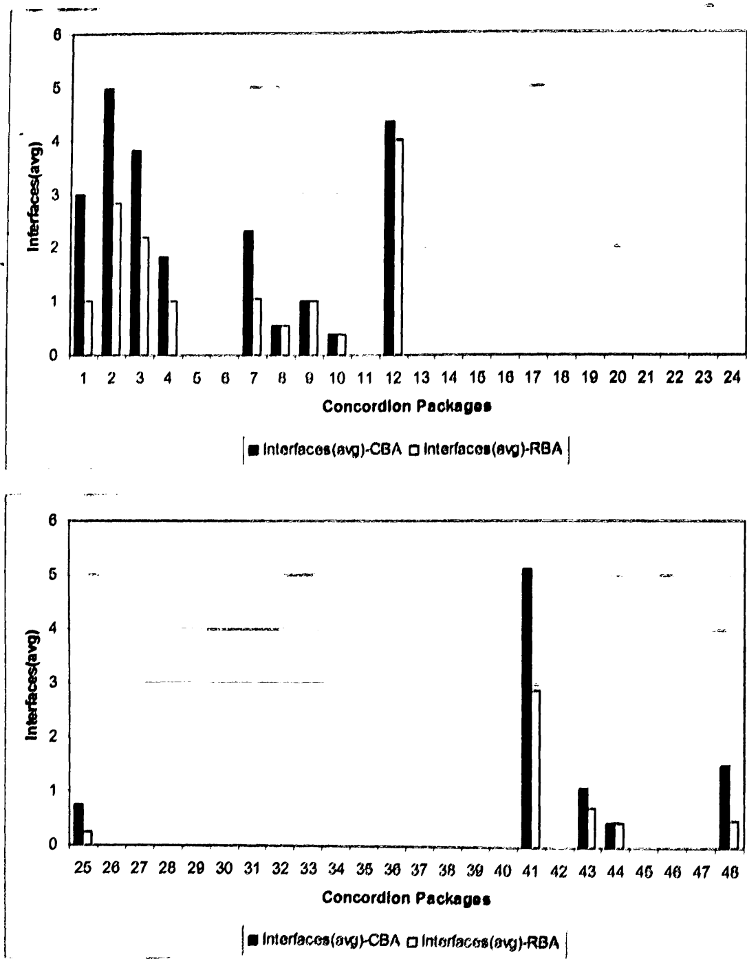
Σχήμα Β.17 Σύγκριση Μέσης Τιμής Πλήθους Διεπαφών μεταξύ CBA Average και RBA.
