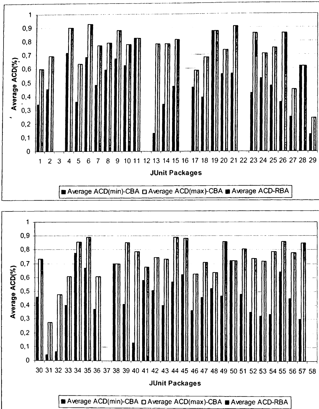
Σχήμα Α.2 Σύγκριση Μέσης Τιμής ACD μεταξύ CBA Average και RBA.
