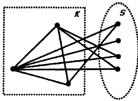
Σχήμα 2.4: Διαμέριση διαχωρισμού γραφήματος.
