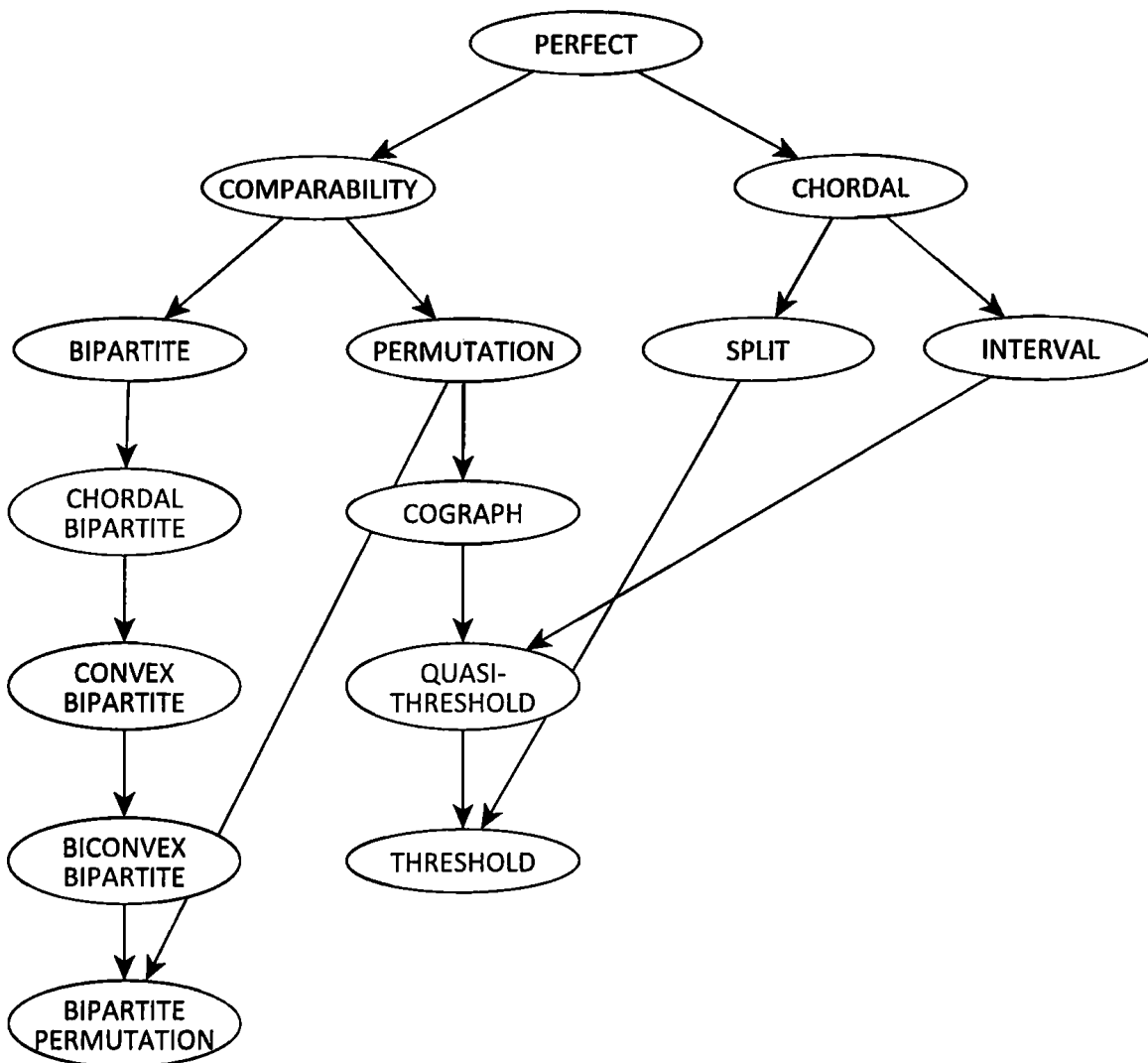
Σχήμα 3.3: Αναπαράσταση της πολυπλοκότητας του προβλήματος εύρεσης του αρμονικού αριθμού για γραφήματα που ανήκουν στις κλάσεις των τέλειων γραφημάτων. Το πρόβλημα στις κλάσεις με κόκκινη έλλειψη είναι NP-πλήρες ενώ στις κλάσεις με μαύρη έλλειψη είναι πολυωνυμικό.
