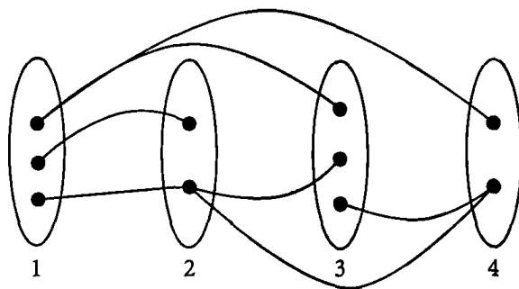
Σχήμα 4.2: Ένας αχρωματικός χρωματισμός του γραφήματος G .
