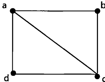
Σχήμα 2.1: Ένα τριγωνικό γράφημα (chordal graph).
