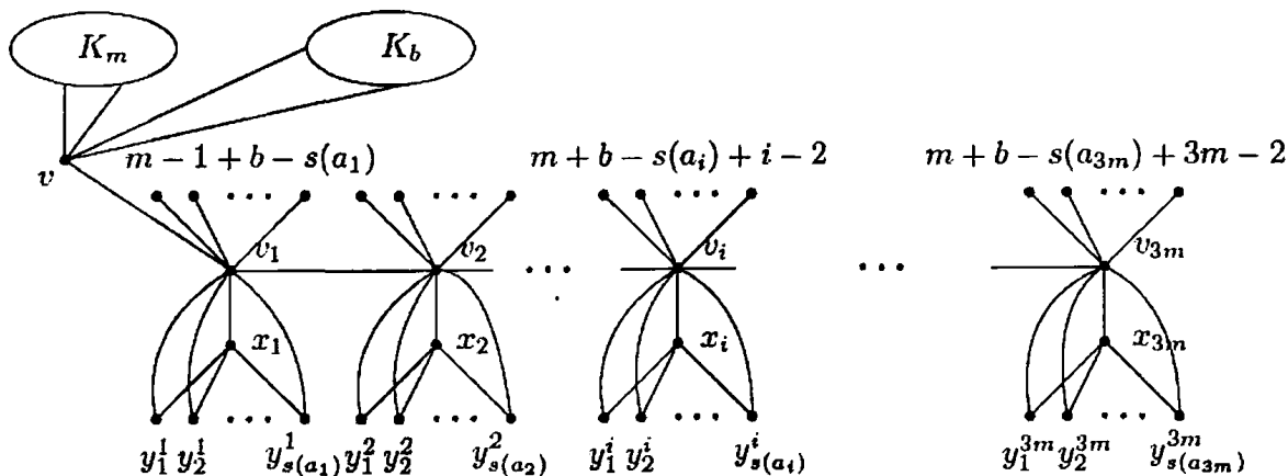
Σχήμα 3.5: Γράφημα διαστημάτων και ταυτόχρονα μεταθετικό γράφημα.
