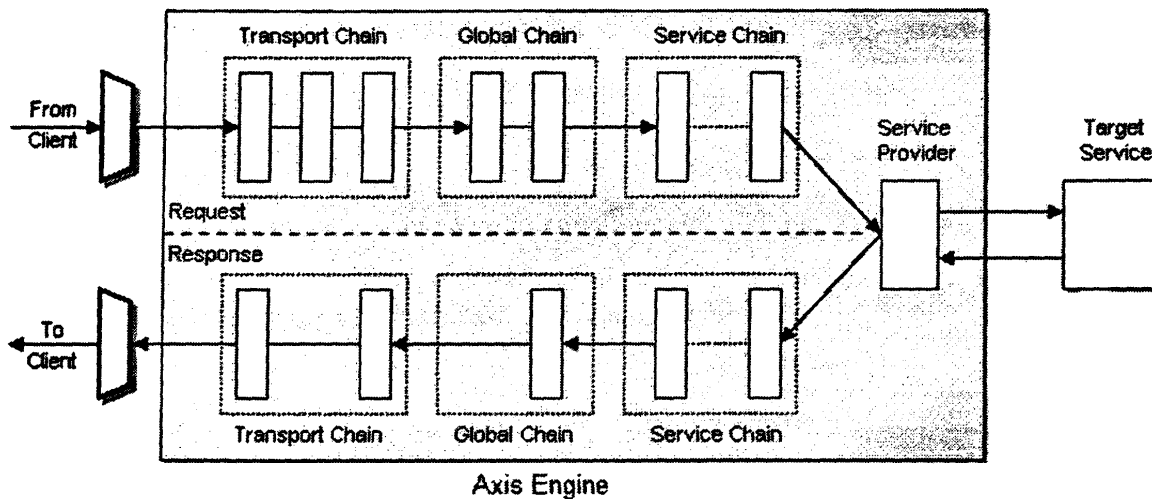
Σχήμα 4.1 Ο μηχανισμός της Axis
