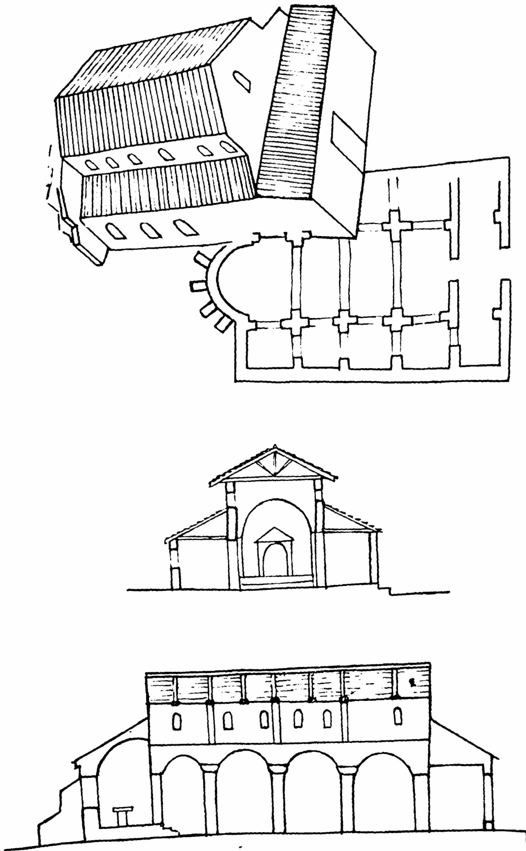
Σχ. 3. Δεύτερη απόπειρα αποκατάστασης της βασιλικής. α. Κάτοψη και τρόπος στέγασης, β. Τομή κατά πλάτος, γ. Τομή κατά μήκος.
