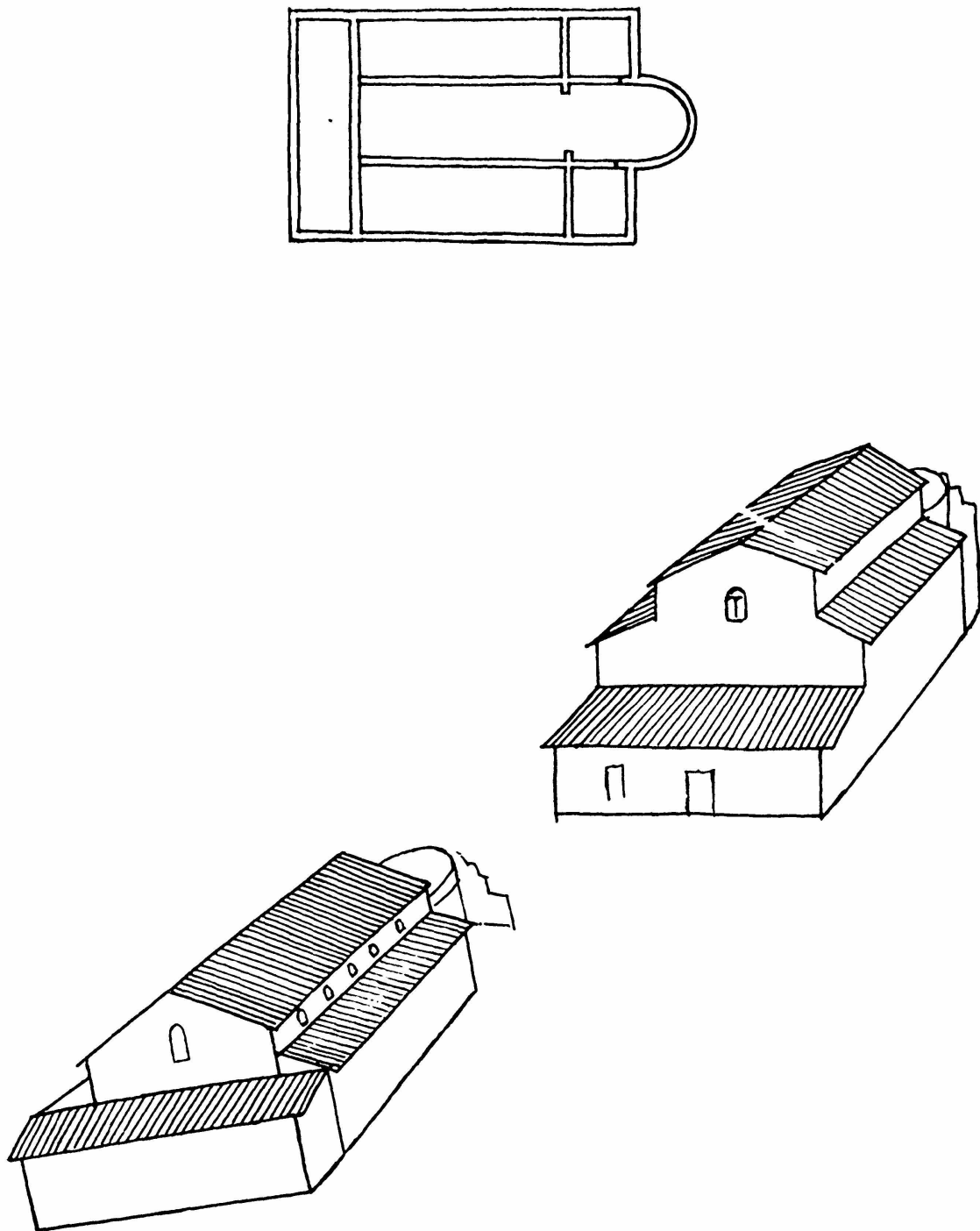
Σχ. 2. Πρώτη απόπειρα αποκατάστασης της βασιλικής. α. κάτοψη, β. πρώτος τρόπος στέγασης, γ. δεύτερος τρόπος στέγασης.
