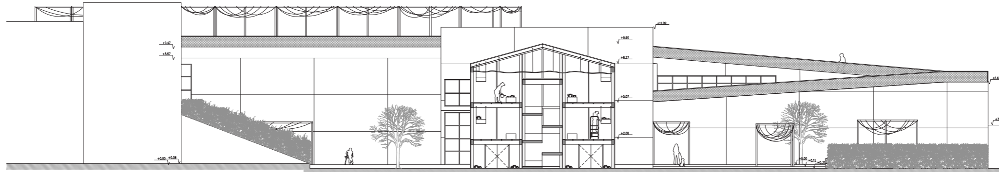
Τομή Β-Β' ΝΟΤΙΑ ΟΨΗ
