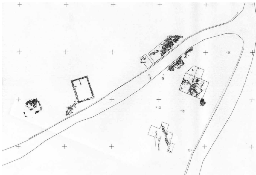
Εικ. 4 α, β: Κάτοψη των κατασκευών του βορείου (α) και του νοτίου (β) συγκροτήματος
